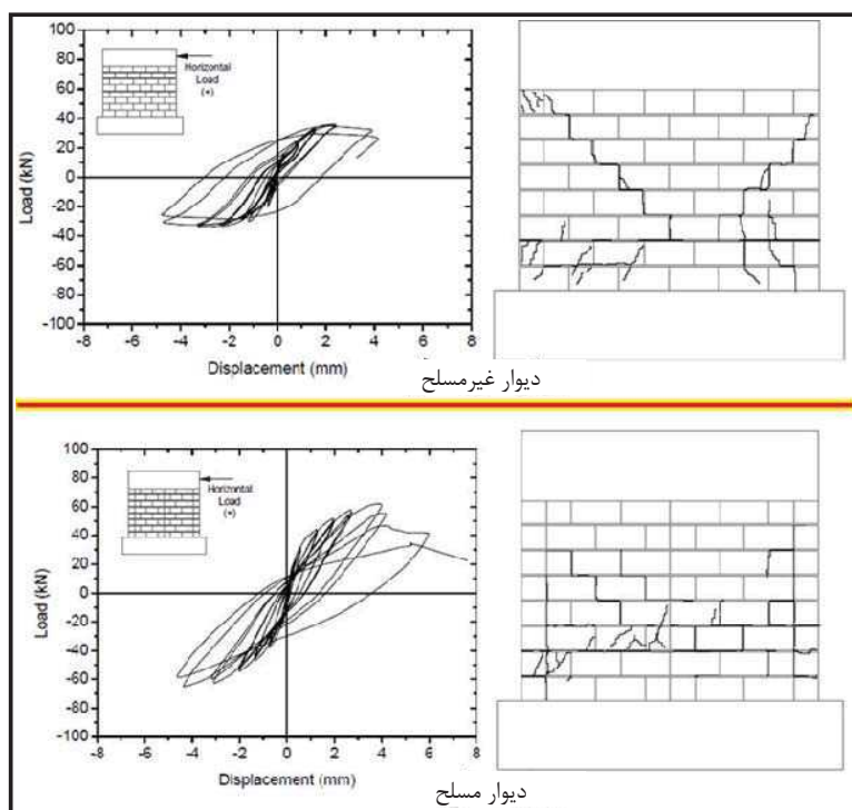
شکل 1-18- مقایسه رفتار درون صفحه دیوار مسلح با رفتار دیوار غیرمسلح متناظر [19]
