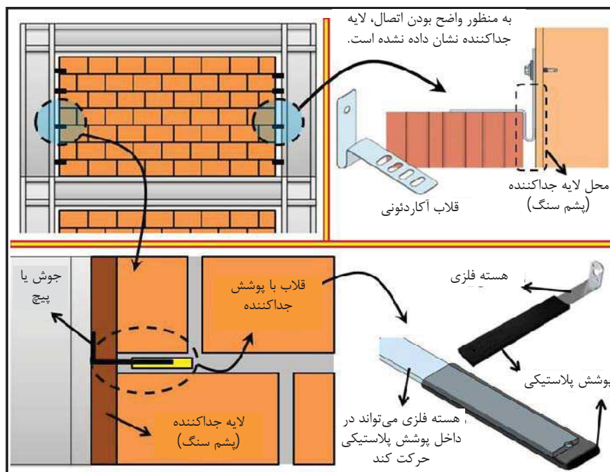
شکل 4-6- اتصال جداساز دیوار به ستون با استفاده از قلاب با پوشش جدا کننده و قلاب آکاردئونی
