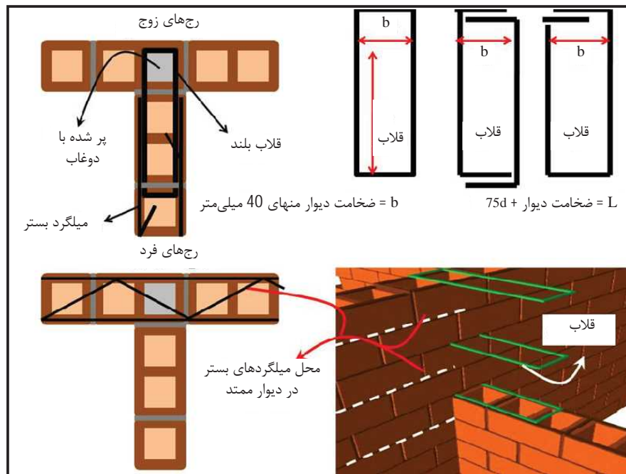
شکل 6-10- اتصال دو دیوار متعامد با استفاده از قلاب بلند و میلگرد بستر - اتصال گیردار
