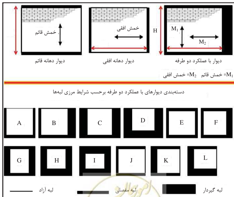
شکل 1-4- دیوارهای دهانه افقی، دهانه قائم و دیوارهای با عملکرد دو طرفه
