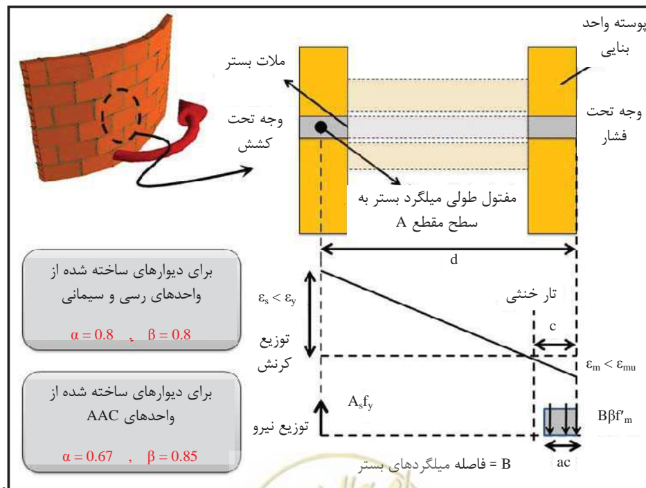
شکل 5-2- توزیع کرنش و نیرو در مقطع دیوار بنایی با میلگرد بستر ساخته شده از واحدهای بنایی توخالی
