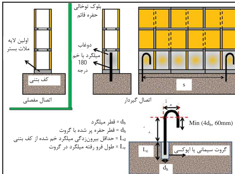
شکل 2-6- اتصال مفصلی و گیردار دیوار بنایی غیرسازه‌ای به کف
