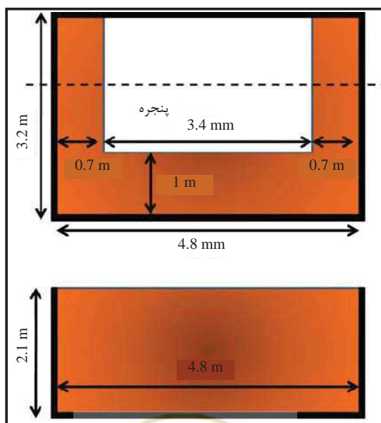
شکل پ.2-9- دیوار D به همراه پانل معادل آن
