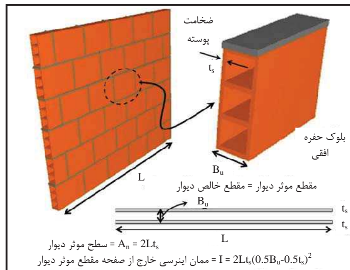
شکل 2-2- مقطع موثر و خالص دیوار ساخته شده با بلوک‌های توخالی حفره افقی و بند بستر تمام ملات
