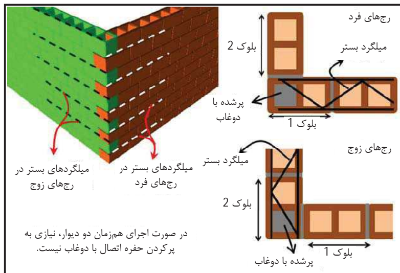
شکل 6-7- اتصال دیوار به دیوار با استفاده از پیوند بنایی (لابند) - اتصال مفصلی
