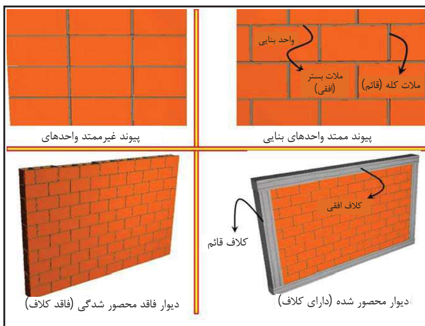
شکل پ.4-2- انواع چینش واحدهای بنایی - دیوارهای محصور شده و محصور نشده
