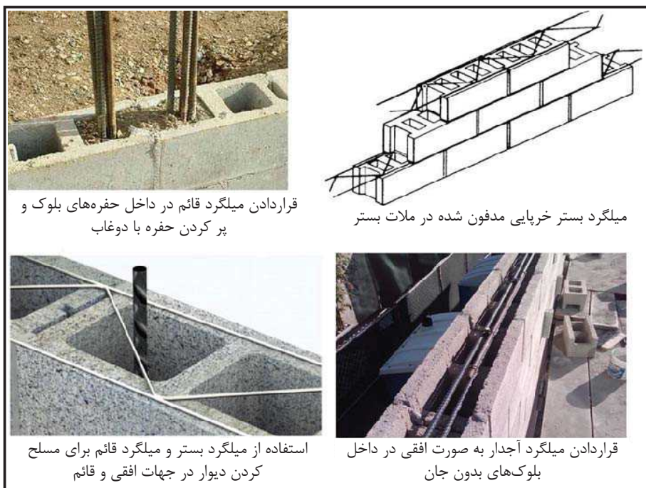
شکل پ. 4-5- دیوارهای بنایی مسلح
