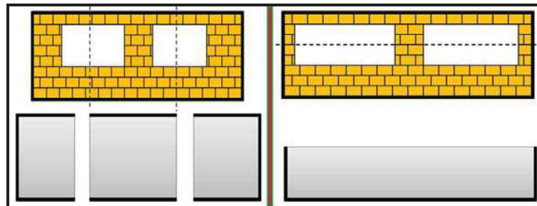
شکل 4-3- تبدیل دیوارهای دارای دو یا چند بازشو به پانل‌های معادل
