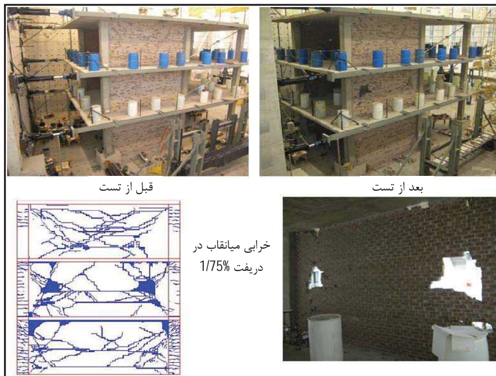
شکل 11-1- رفتار نامناسب میانقاب بنایی غیرمسلح و فروریزش آن در حین تست شبه دینامیکی [17]
