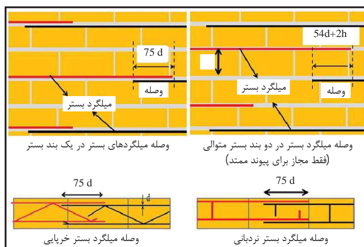
شکل 5-3- الزامات مربوط به وصله میلگردهای بستر
