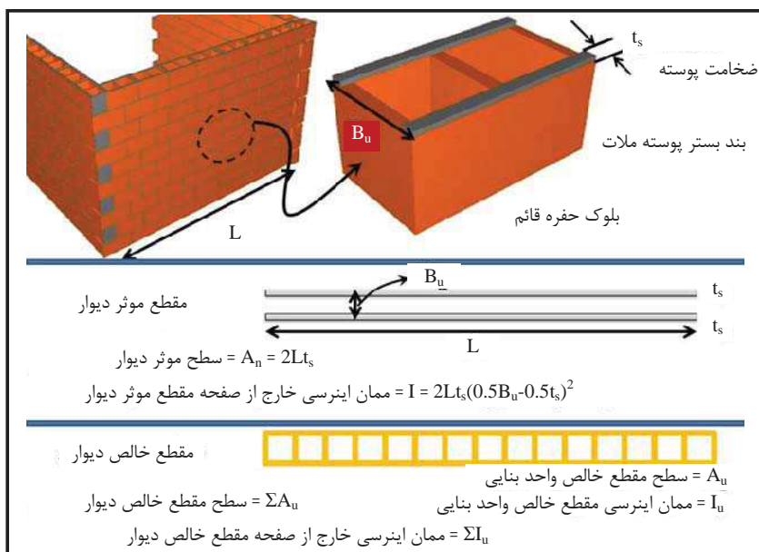
شکل 1-2- مقطع موثر و خالص دیوار ساخته شده با بلوک‌های توخالی حفره قائم و بند بستر پوسته ملات
