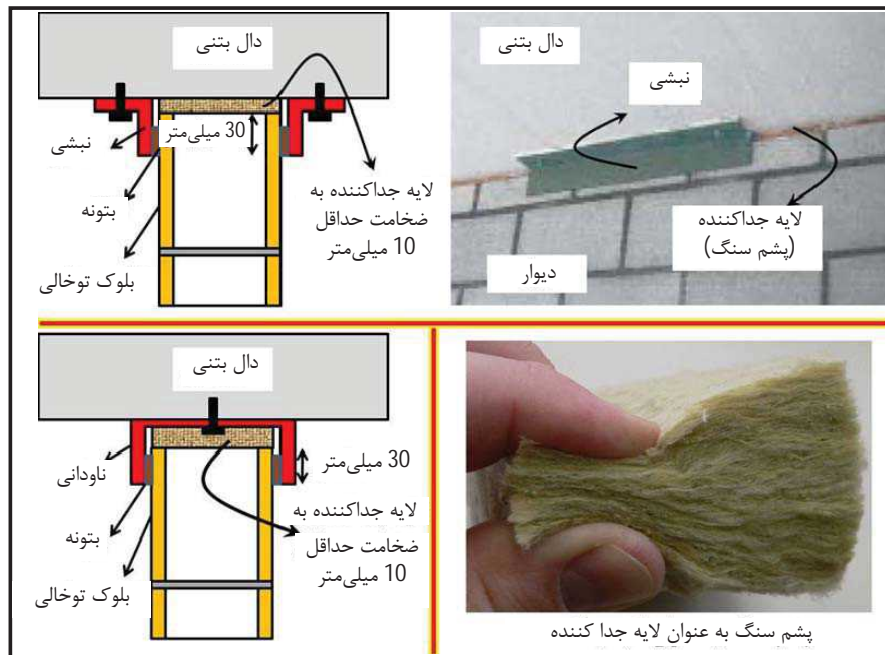
شکل 6-3- اتصال مفصلی دیوار به سقف
