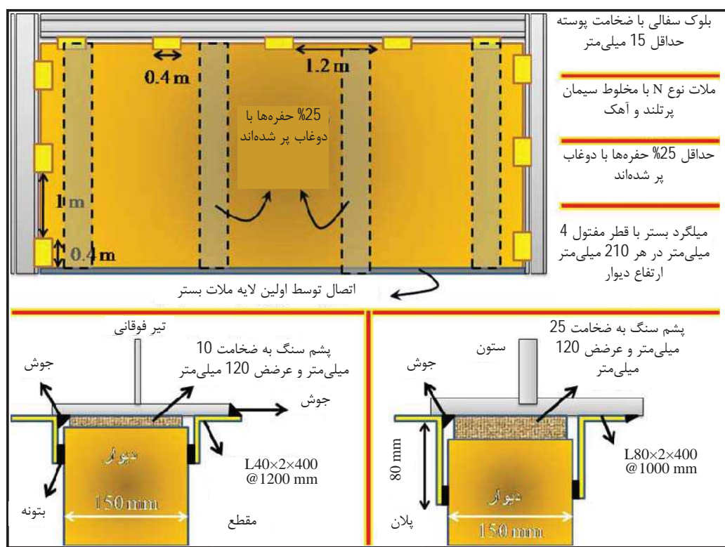
شکل پ.2-4- طرح نهایی دیوار A
