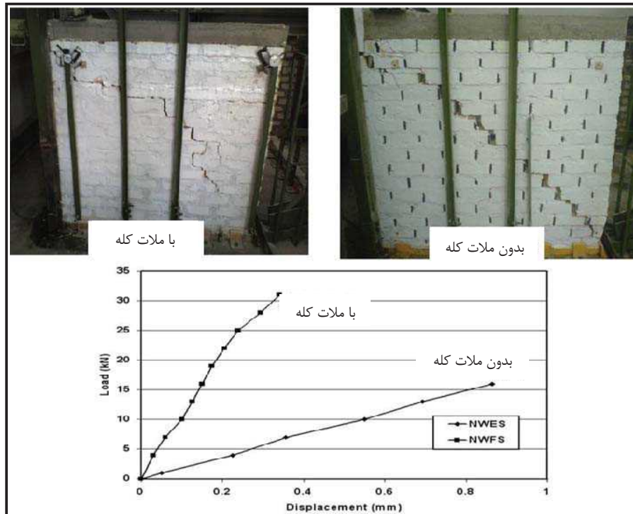
شکل 1-7- اثر ملات کله (قائم) در رفتار داخل صفحه دیوار [2]
