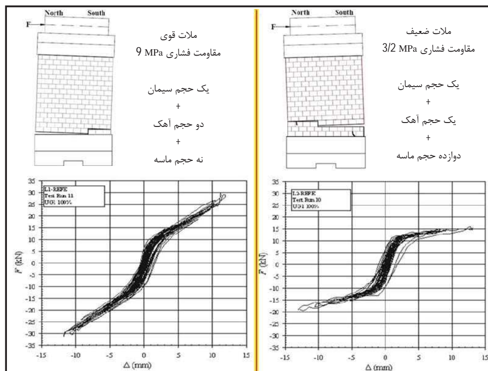
شکل 8-1- تاثیر نوع ملات بر رفتار داخل صفحه دیوارهای بنایی غیرمسلح [10]
