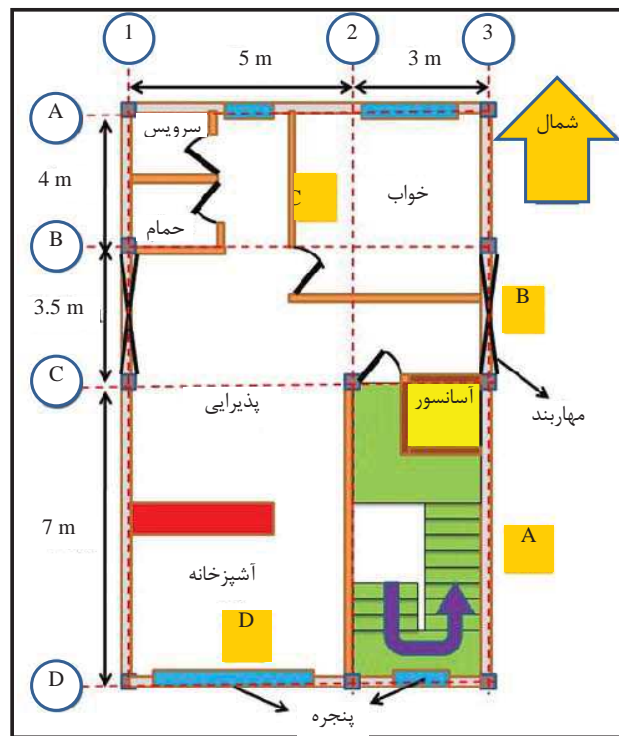
شکل پ.2-1- پلان ساختمان مورد نظر
