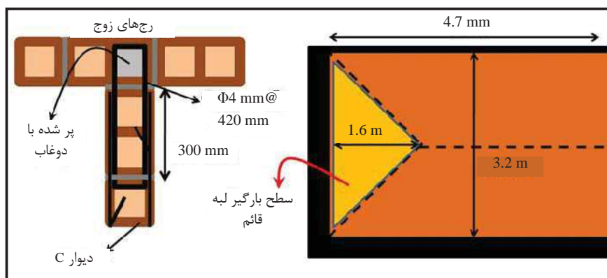
شکل پ. 2-8- اتصال گیردار دیوار به دیوار برای دیوار C
