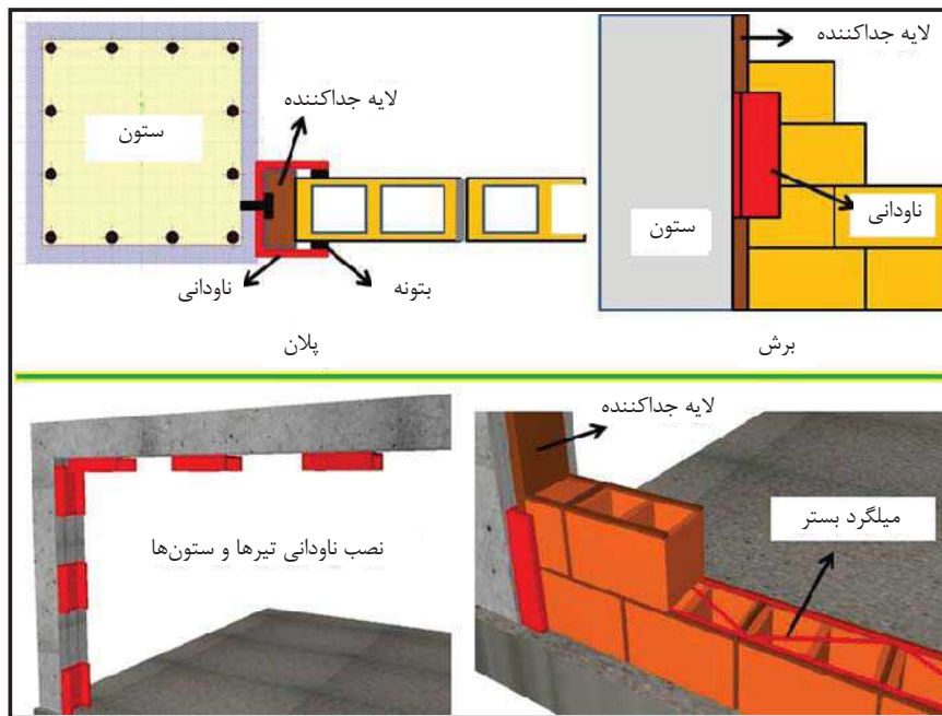
شکل 6-5- اتصال جداشده دیوار به قاب سازه‌ای با ناودانی و لایه جداکننده
