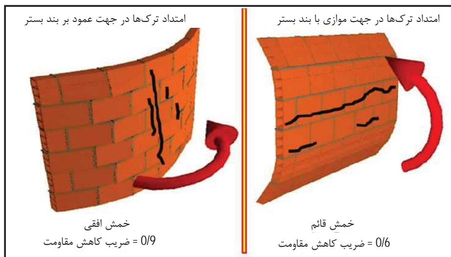
شکل 5-1- خمش افقی و قائم به همراه ضرایب کاهش مقاومت خمشی در دیوارهای بنایی دارای میلگرد بستر افقی
