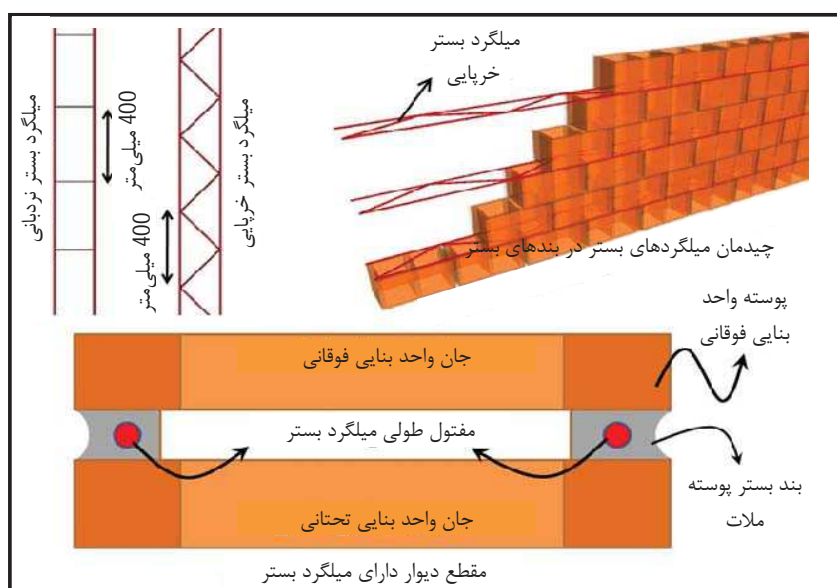
شکل 3-2- مشخصات هندسی میلگردهای بستر و چینش آن‌ها به عنوان میلگرد افقی در دیوار
