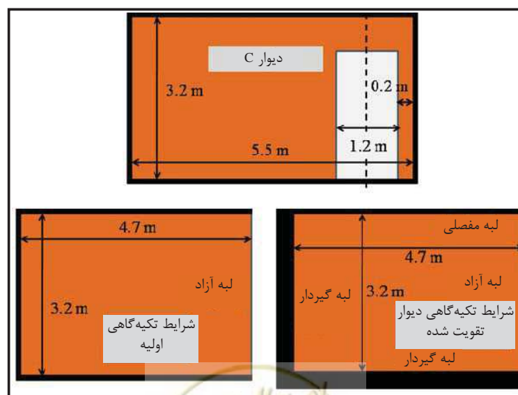
شکل پ.2-6- ابعاد و شرایط تکیه‌گاهی اولیه دیوار C
