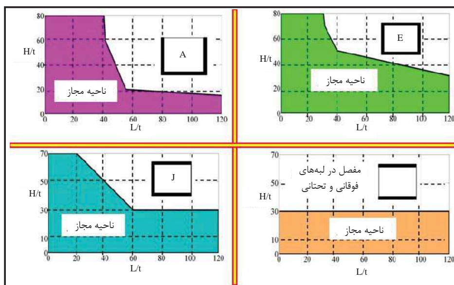
شکل 6-1- حداقل ضخامت دیوار بر حسب شرایط مرزی
