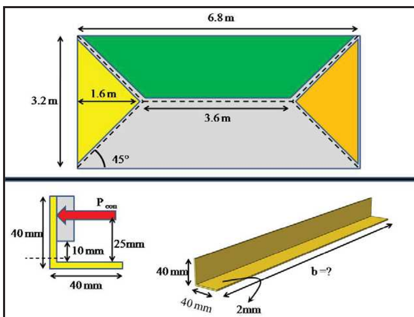
شکل پ.2-3- سطح بارگیر لبه فوقانی دیوار و طراحی نبشی در اتصال جداکننده دیوار به سقف
