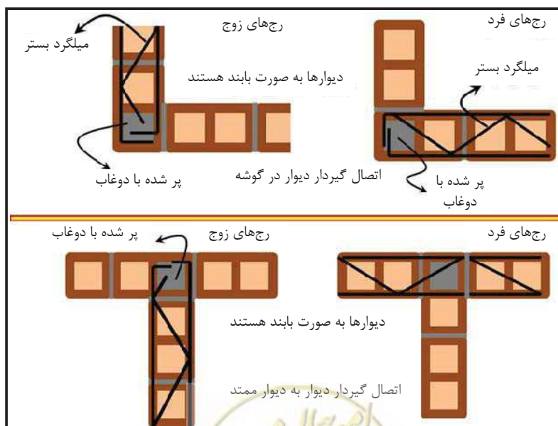
شکل 6-8- اتصال دیوار به دیوار با استفاده از پیوند بنایی (لابند) و میلگرد بستر - اتصال گیردار
