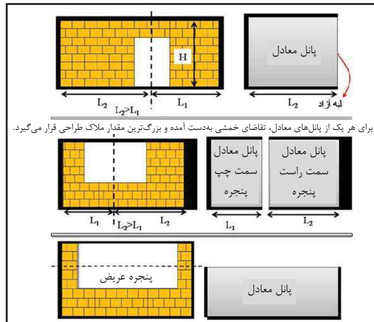
شکل 4-2- تقسیم دیوار دارای بازشو به پانل‌های معادل
