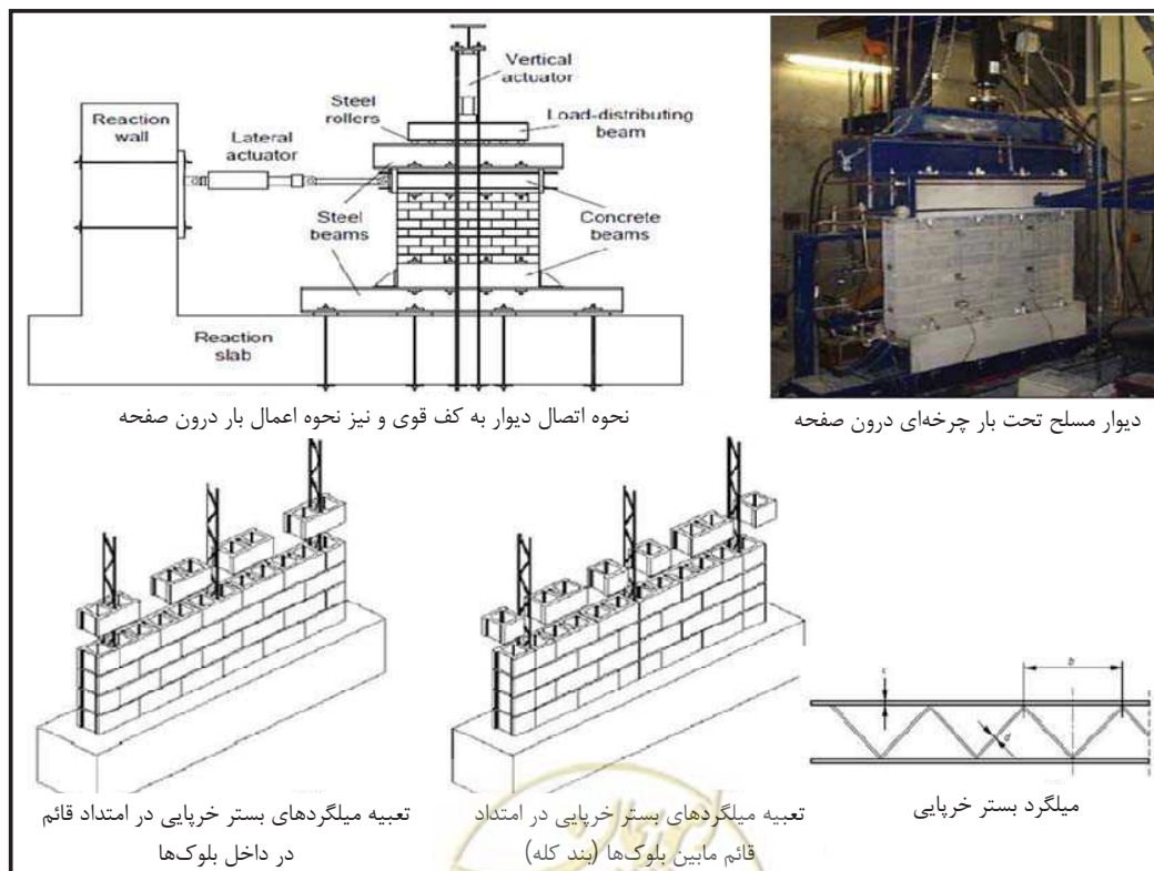
شکل 1-17- تعبیه میلگرد بستر خرابایی در جهت افقی و قائم و آماده‌سازی دیوار برای انجام تست [19]
