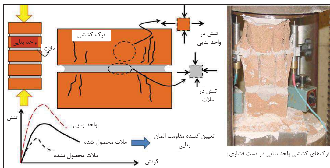
شکل 1-1- تاثیر مقاومت واحد بنایی و ملات در مقاومت فشاری المان بنایی
