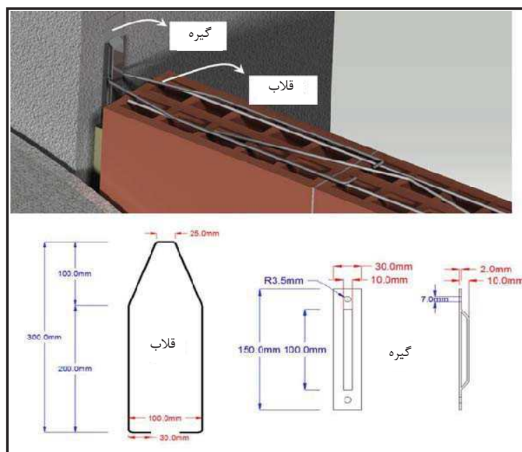
شکل 6-6- اتصال جدانشده دیوار به ستون با استفاده از قلاب و گیره (Tie and Anchor)
