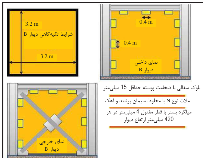
شکل پ. 2-5- طراحی دیوار B به همراه جزئیات آن
