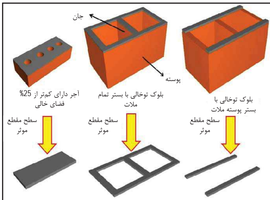
شکل پ.4-4- سطح مقطع موثر در واحدهای بنایی گوناگون با ملات بستر گوناگون
