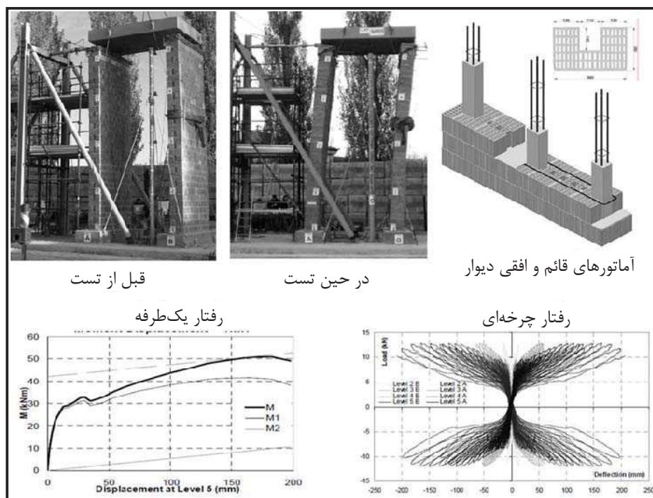
شکل 12-1- تست چرخه‌ای بر روی دیوار بنایی مسلح در امتداد خارج از صفحه [20]
