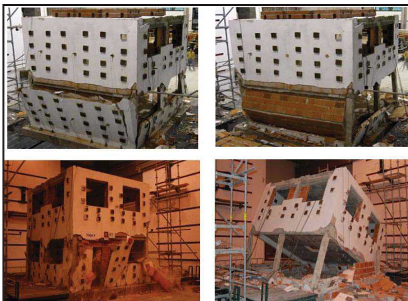
شکل 1-13- فروریزش خارج از صفحه میانقاب‌های دو لایه فاقد میلگرد بستر [21]
