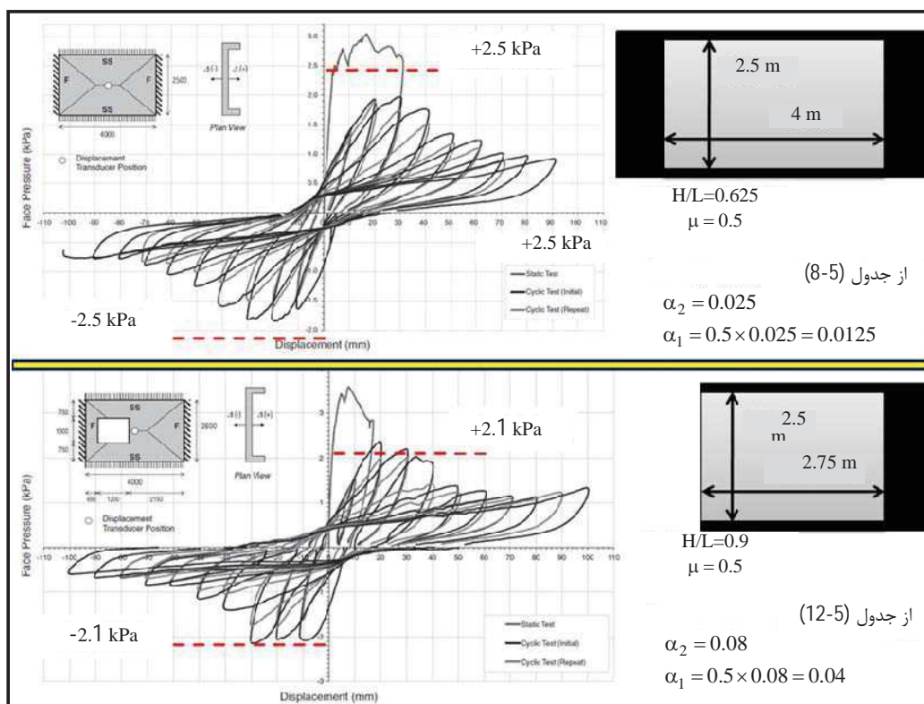
شکل پ.1-1- مقایسه فشار شکست به دست آمده از روش ضرایب خمش با نتایج آزمایشگاهی
