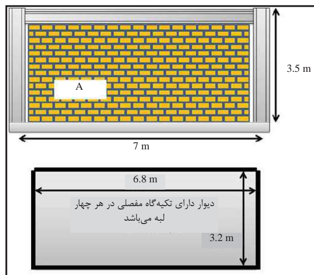
شکل پ.2-2- ابعاد و شرایط تکیه‌گاهی دیوار A
