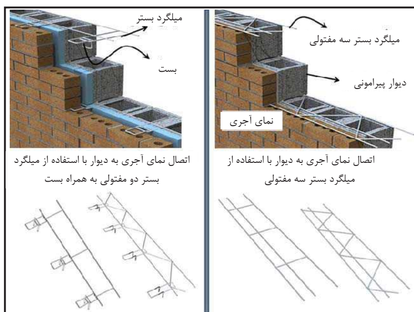
شکل 3-3- اتصال نمای بنایی به دیوارهای پیرامونی با استفاده از میلگردهای بستر
