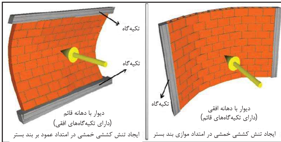
شکل پ.4-3- خمش خارج از صفحه دیوارهای بنایی با دهانه‌های قائم و افقی
