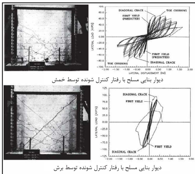
شکل 1-16- مقایسه رفتار دیوارهای بنایی مسلح با مکانیزم تخریب خمشی و برشی [23]
