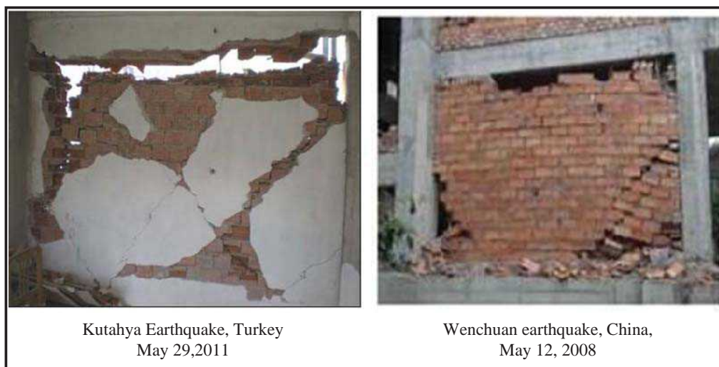
شکل 1-10- خرابی داخل صفحه میانقاب‌های رسی (سفالی) غیرمسلح در زلزله‌های کوتاهیا و ونچوان
