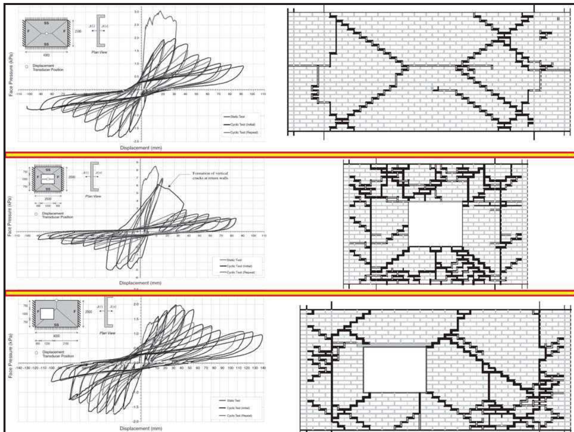
شکل 6-1- رفتار خارج از صفحه دیوارهای بنایی غیرمسلح به همراه ترک‌های ایجاد شده [7]
