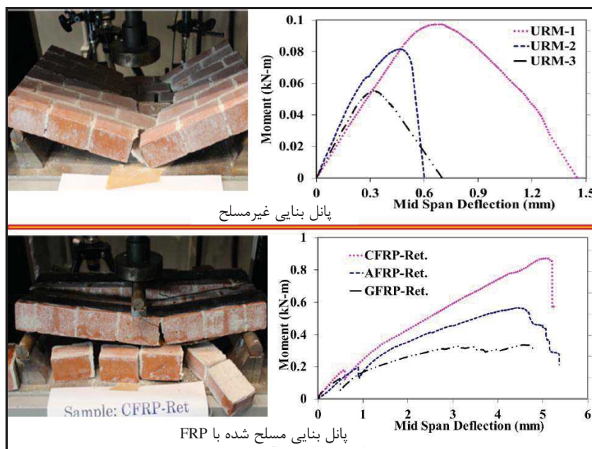
شکل 15-1- مسلح کردن المان بنایی با استفاده از FRP برای بهبود رفتار خمشی [22]
