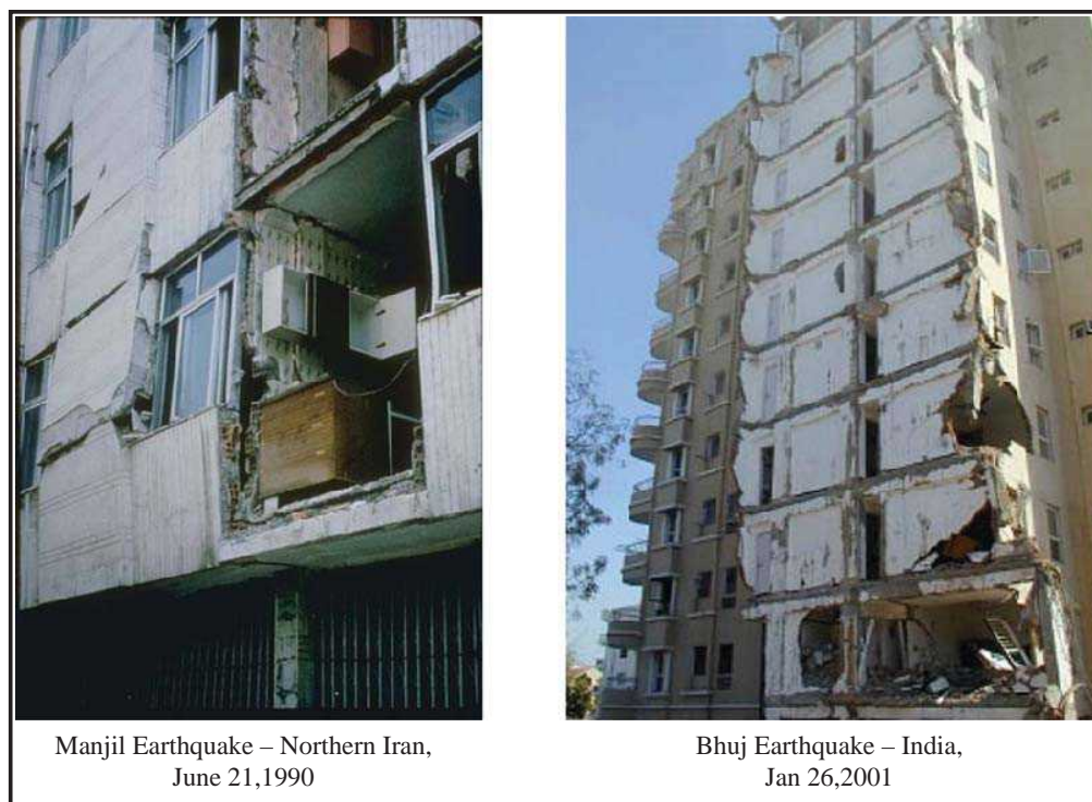
شکل 1-4- تخریب خارج از صفحه دیوارهای بنایی غیرمسلح در زلزله‌های منجیل و بوج
