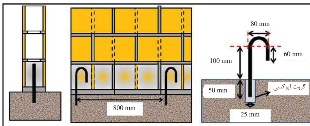
شکل پ. 2-7- جزئیات اتصال گیردار دیوار C به کف بتنی
