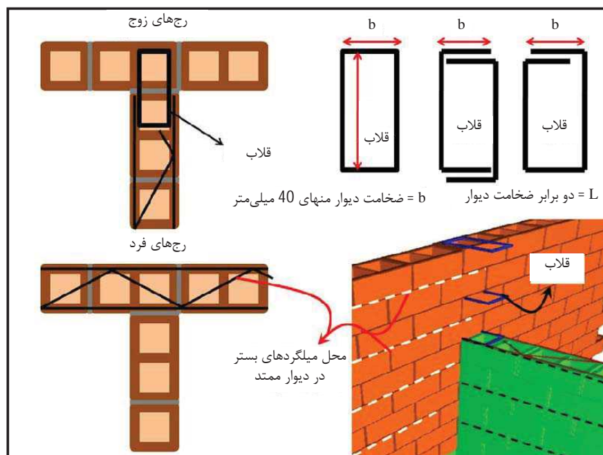
شکل 6-9- اتصال دو دیوار متعامد با استفاده از قلاب و میلگرد بستر - اتصال مفصلی
