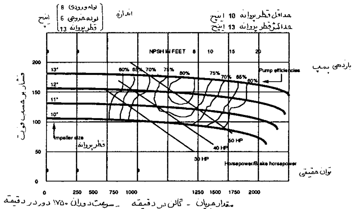
شکل ۶-۱ منحنی های پمپ
