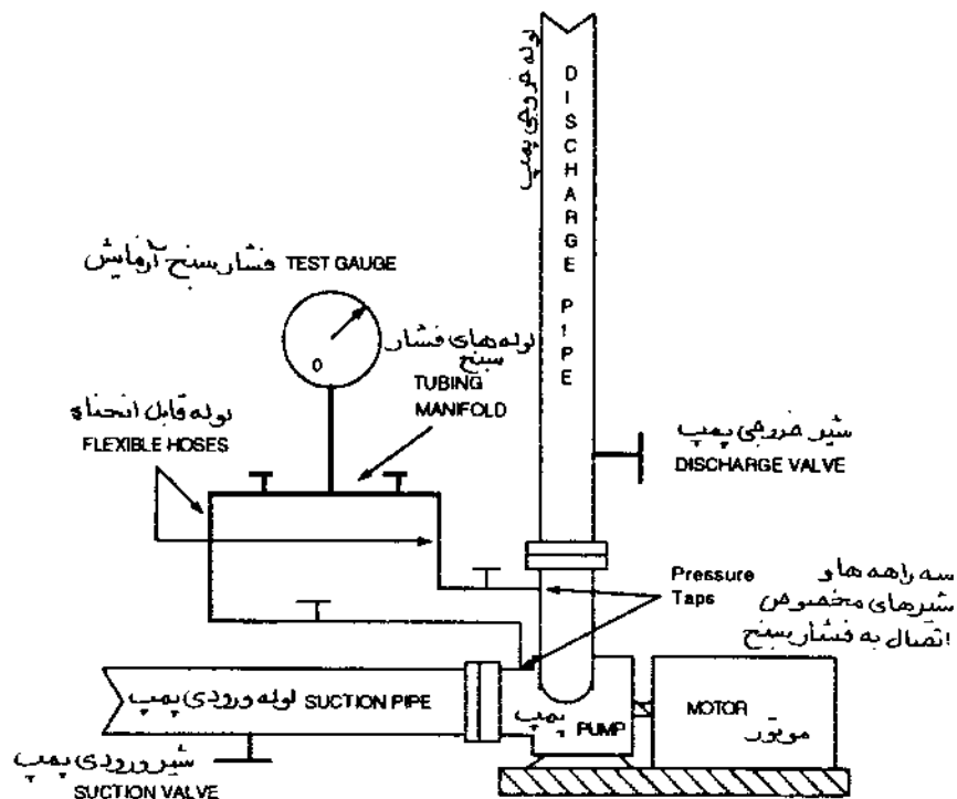
شکل ۵-۳ فشار سنچ و لوله های آن در نوع بوردون
