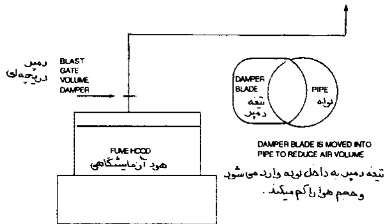
شکل ۴-۸ دمپره دریچه‌ای
