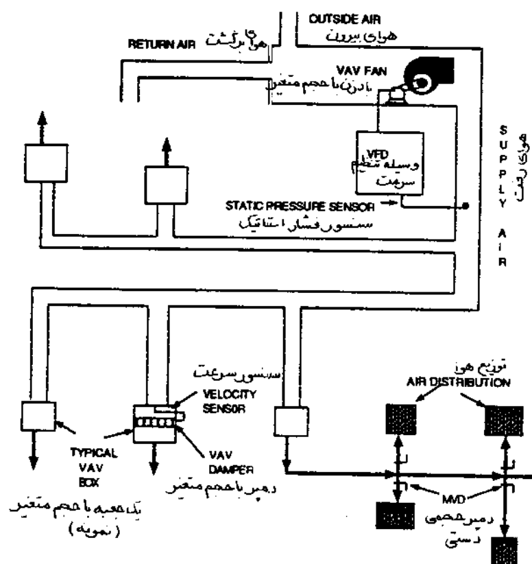
شکل ۲۲-۳ جعبه های حجم متغیر مستقل از فشار
