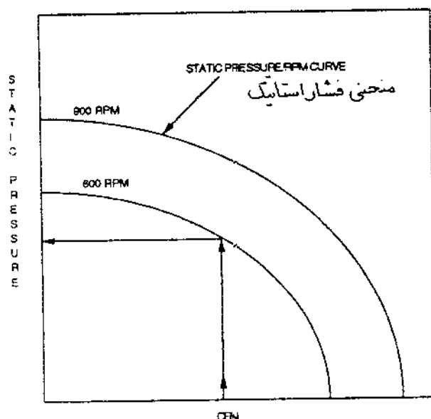
شکل ۲-۴ تعیین فشار استاتیک با داشتن مقدار هوادهی و سرعت دورانی
