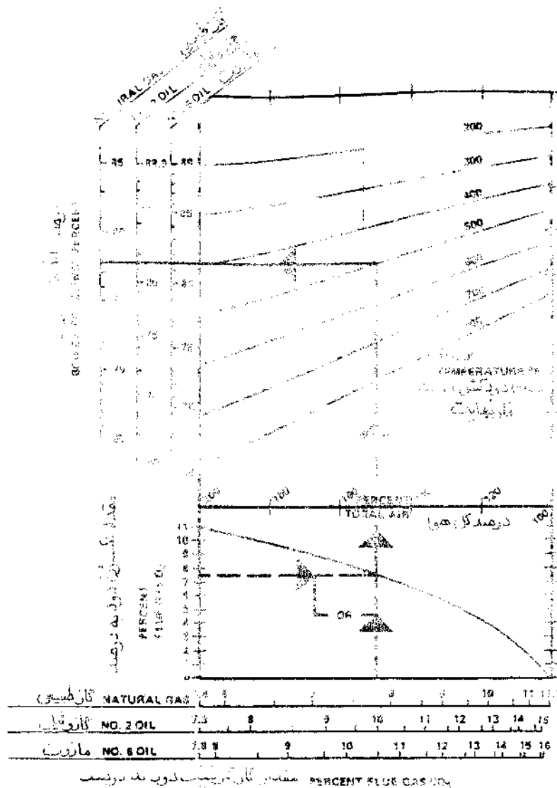
شکل ۸-۱ اثر ترکیب دود و دمای دود بر راندمان دیگ
