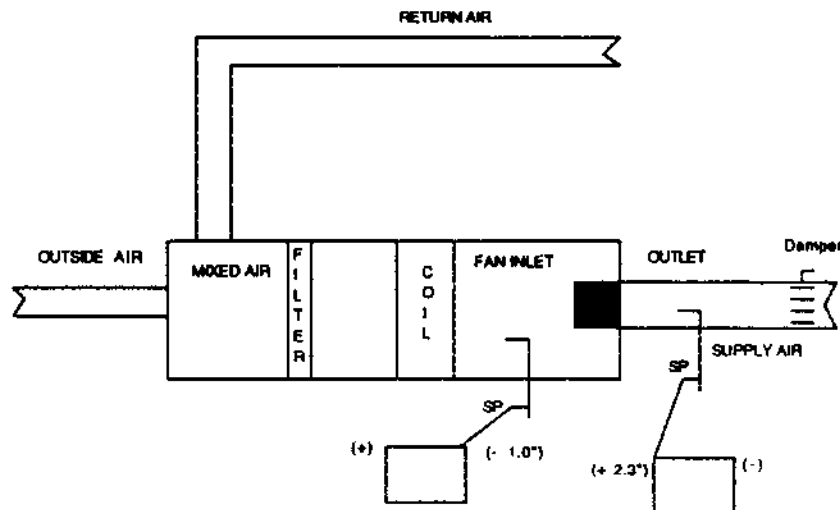
شکل ۱-۹ اندازه‌گیری فشار استاتیک کل بادزن
