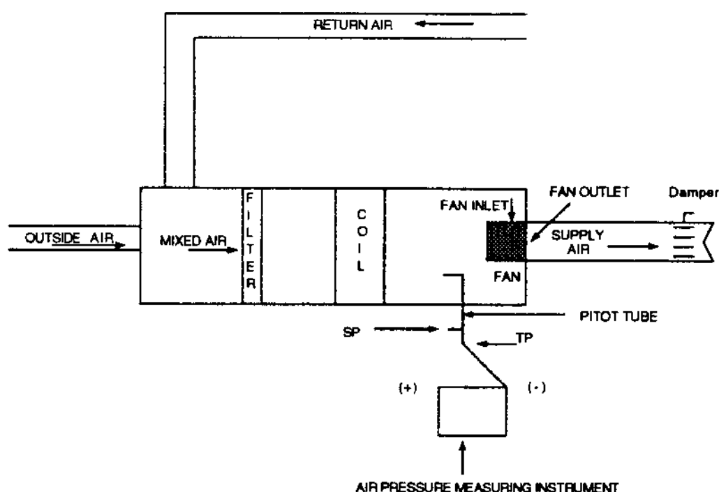
شکل ۱-۵ اندازه‌گیری فشار کل در مکش بادزن
