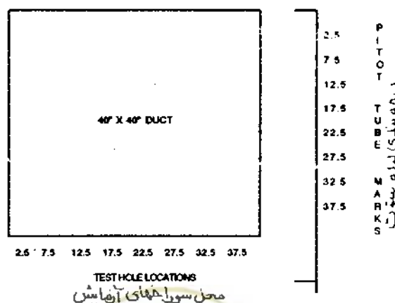
شکل ۳-۸ محل سوراخهای تست و درجه‌بندی لوله پیتوت
