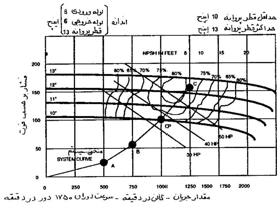
شکل ۶-۲ منحنی سیستم
