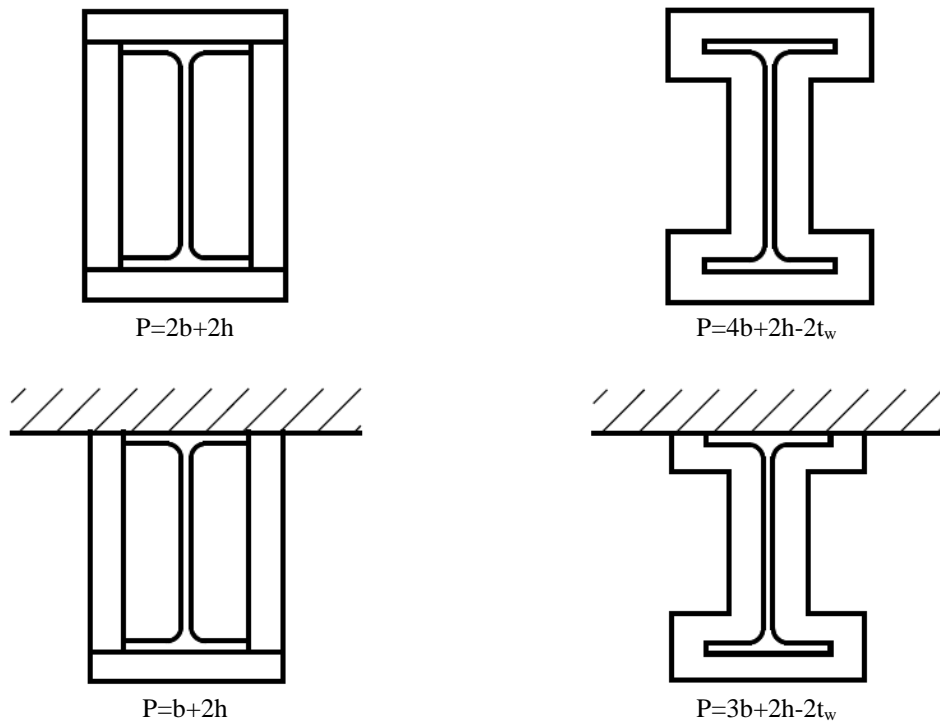
شكل ۴-۱- نحوه تعيين ضريب مقطع براي ستون ها و تيرهاي فولادي با مقطع I يا H شكل
