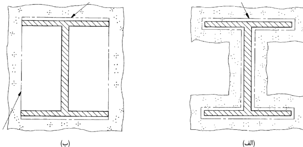
شکل ۵-۶- مواردی از کاربرد مش فولادی در گیر کننده
