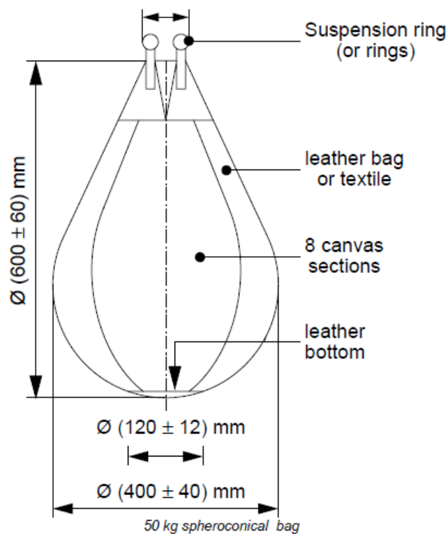
شکل ۳- ۱- ضربه زننده جسم نرم
