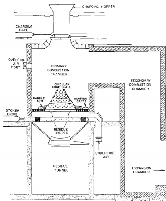
شکل ۳: کوره سیلندر عمودی
