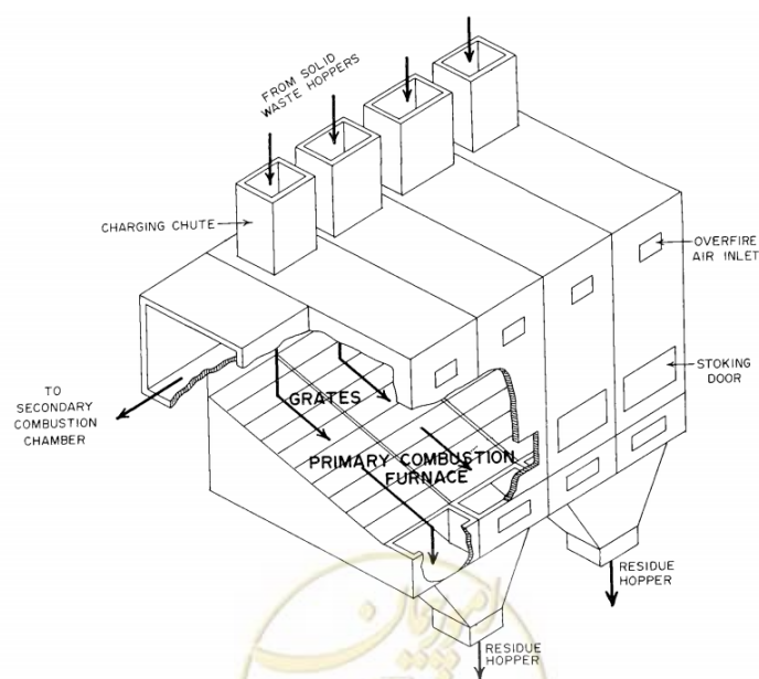
شکل ۴: کوره چندسلولی مستطیل شکل
