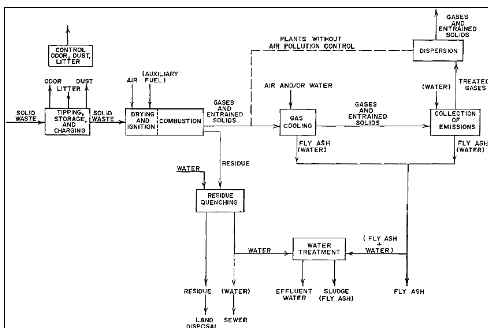
شکل ۱۱: نمودار سیستم های داخلی کارخانه بر پایه جمع آوری و انتقال خاکستر بادی خشک از فرایندهای خنک سازی و جمع آوری
