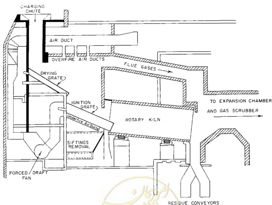
شکل ۶: کوره دوار
