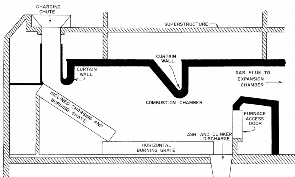
شکل ۵: کوره مستطیل شکل
