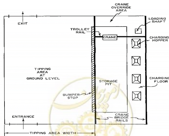
شکل ۱: نمای سالن تخلیه و سالن ذخیره همراه با جرثقیل
