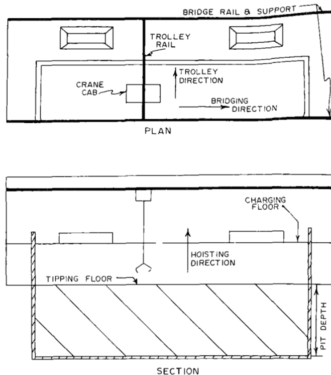
شکل ۲: نمای بالا و نمای برش‌یافته (مقطعی) از جرثقیل سقفی
