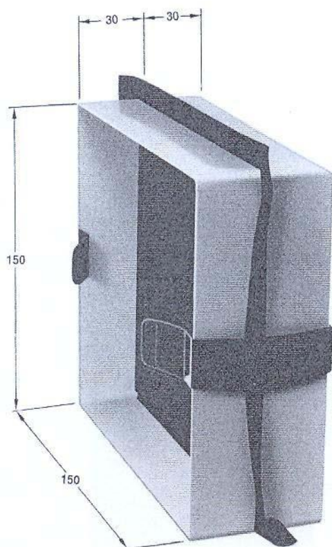
شکل ۳-۱: قاب نگهدارنده برای نشان دهنده‌های عمودی
