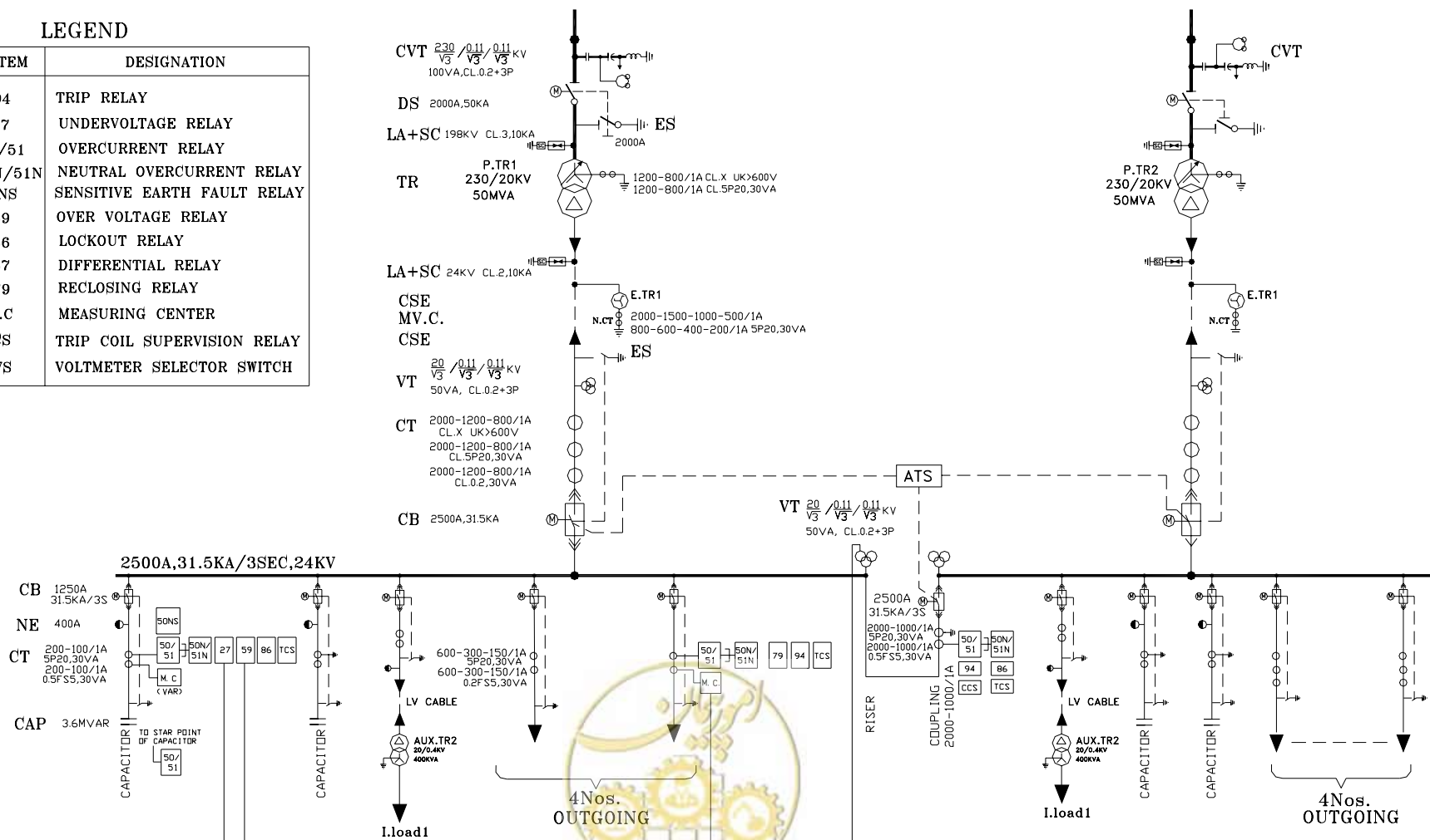
شکل ۱-۲: دیاگرام تک خطی یک سوئیچگیر ۲۰ کیلوولت نمونه
