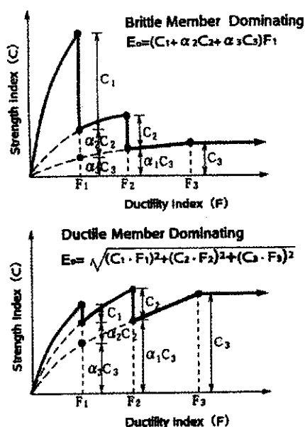
شکل ۳: برش طبقه - رابطه‌های تغییر با انواع مختلف از اعضای عمودی
