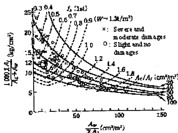
شکل ۵: نتایج اولین تفکیک ( I_S ) و سطوح خرابی در زلزله ۱۹۶۸ توکاچی اکایی و ۱۹۷۸ میاگیکن اکایی
