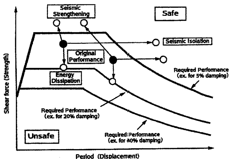
شکل ۱۱: مقاوم سازی، جدا سازی و استهلاک انرژی لرزه‌ای
