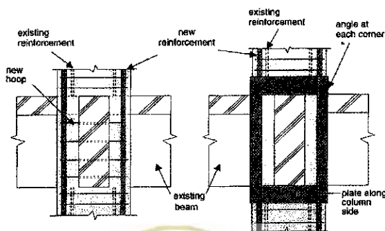
شکل ۱۷: محدود نمودن اتصال
