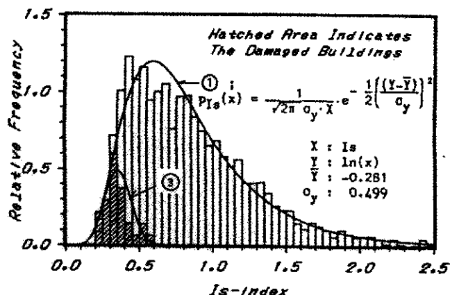
شکل ۴: هیستوگرام ظرفیت لرزه‌ای بتن‌آرمه RC موجود در ژاپن که به وسیله استانداردهای ارزیابی ظرفیت لرزه‌ای ارزیابی شد.
