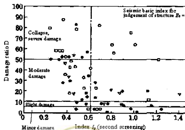
شکل ۸: نتایج دومین تفکیک ( I_s ) و سطوح خرابی به وسیله زلزله هیوگوکن ۱۹۹۵ (زلزله کوبه)
