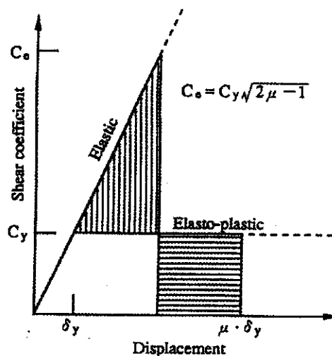
شکل: پاسخ الاستیک و الاستوپلاستیک
