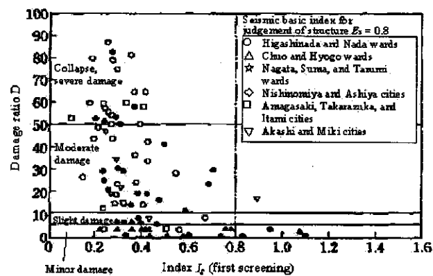
شکل ۷: نتایج اولین تفکیک ( I_s ) و سطوح خرابی زلزله ۱۹۹۵ هیوگوکن نانبو (زلزله کوبه)
