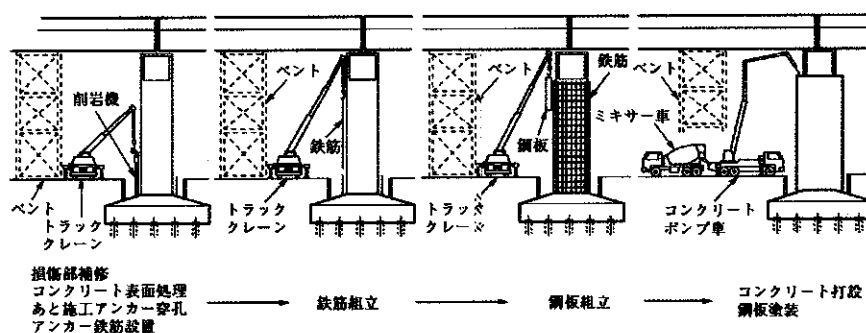
شکل شماره ۴- مراحل ساخت پایه‌های مرمت‌شده و تقویت‌شده
