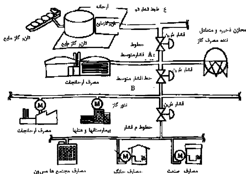
شکل ۱: کلیات سیستم گازرسانی شرکت گاز اوزاکا
