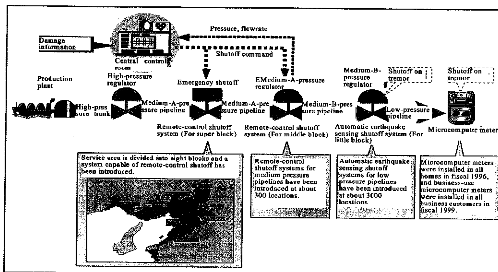
شکل ۳-۲: کلیات سیستم قطع گاز [۴]
