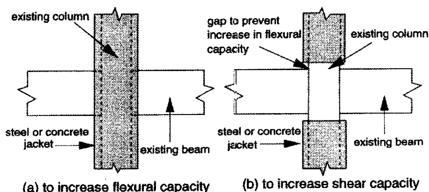
شکل ۱۴: پوشش ستون
