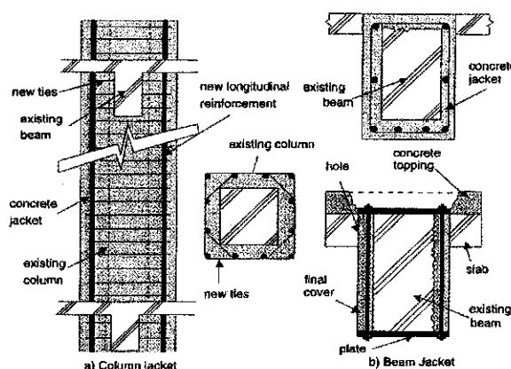
شکل ۱۶: پوشش به منظور افزایش ظرفیت خمشی
