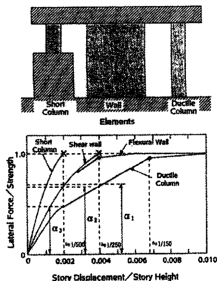
شکل ۲: طبقه ایده‌آل ساختمان و رابطه‌های مکان بارگذاری تغییر مکان المان‌ها
