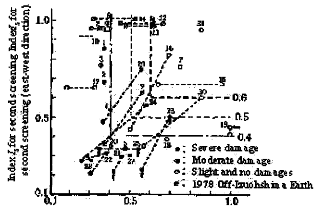
شکل ۶: نتایج دومین تفکیک ( I_s ) و سطوح خرابی زلزله ۱۹۶۸ توکاجی اکایی و ۱۹۷۸ میاگیکن اوکایی و ۱۹۷۸ ایزوشیما- کینکا
