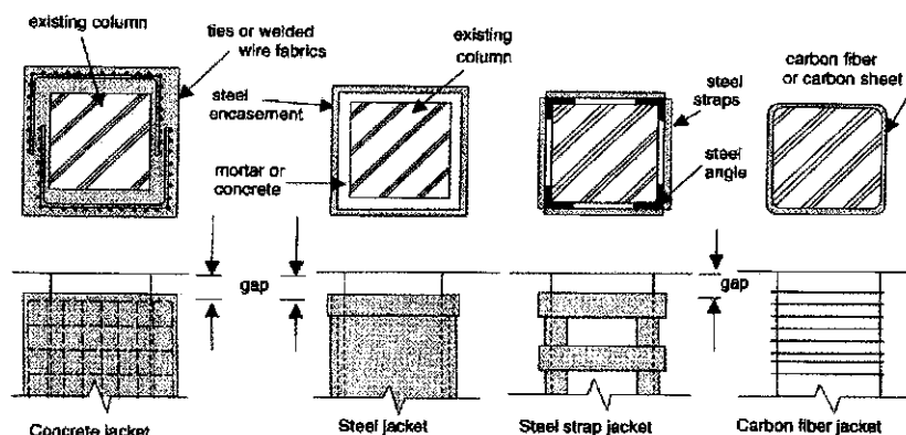
شکل ۱۵: پوشش به منظور افزایش ظرفیت برشی
