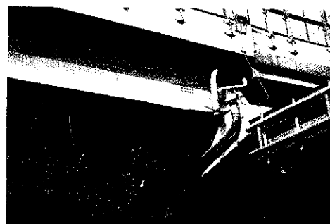
b) Buckling
