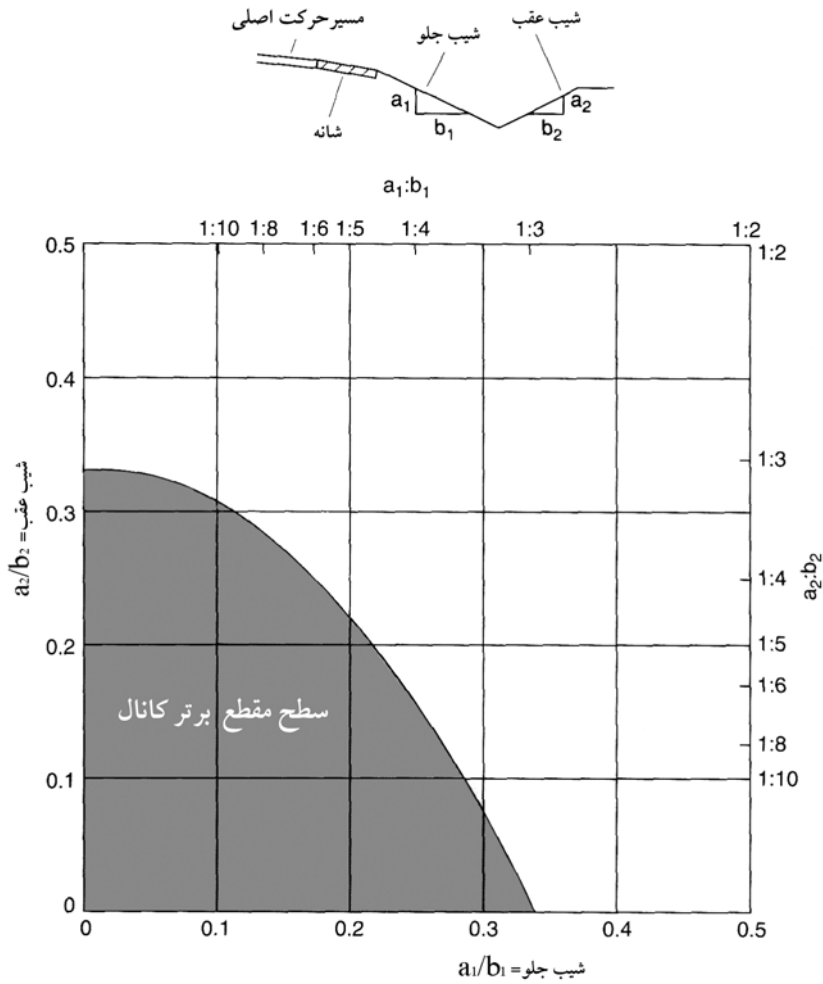
شکل ۳-۴- سطح مقطعهای برتر با تغییر شیب ناگهانی برای کانالهای کناری، نمودار مزبور برای تمام کانالهای ۷ شکل، کانالهای گرد با عرض تحتانی کمتر از ۲/۴ متر و کانالهای دوزنقه‌ای با عرض کف کمتر از ۱/۲ متر قابل استفاده است.
