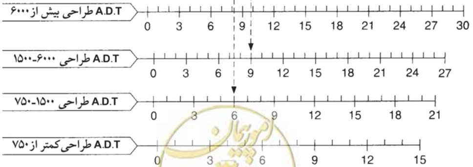
شکل ۳-۱- منحنی‌های تعیین عرض ناحیه بازیابی عرض ناحیه بازیابی (متر)
