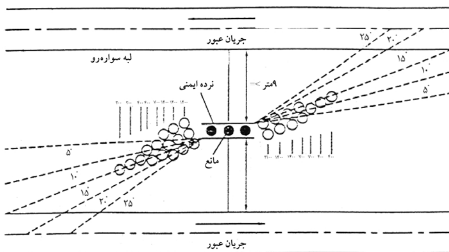
پلان
