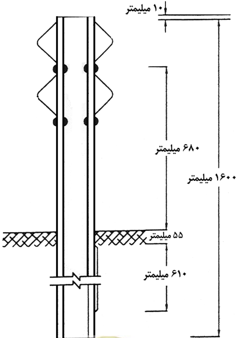
شکل ۳-۹- حفاظ فلزی با سپر دوج
