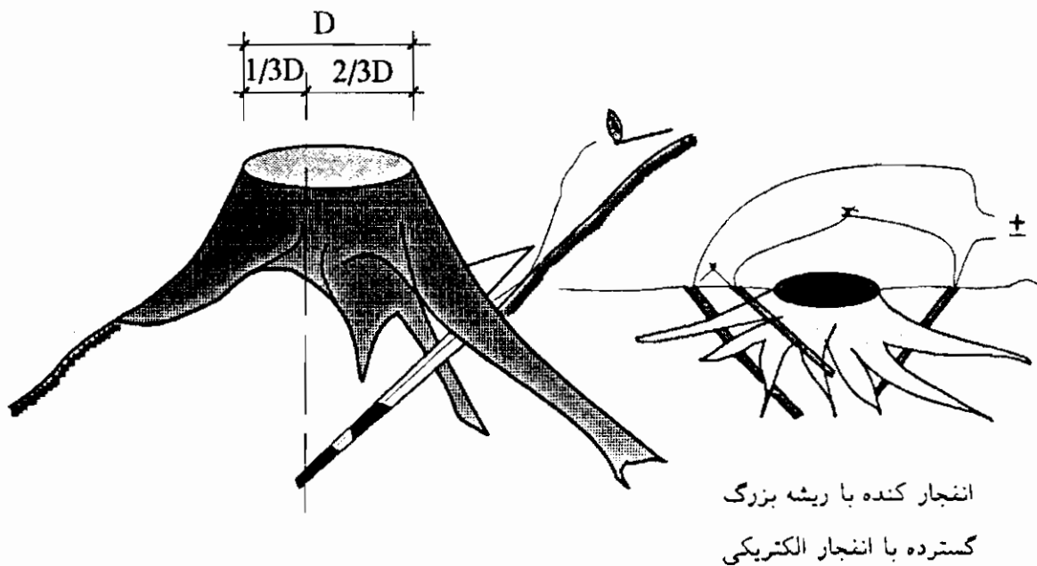
شکل ۳-۴ - روش‌های منفجر کردن کنده
