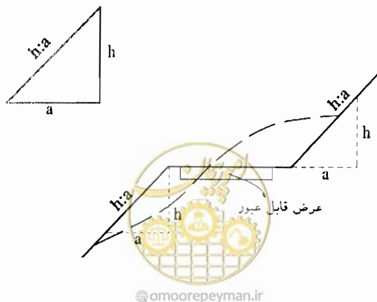
شکل ۴-۲- طرز نمایش شیب شیروانی‌ها در راه‌های جنگلی
