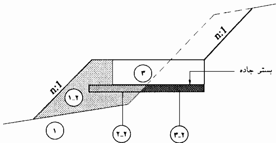
شکل ۳-۱ - قسمت‌های مختلف زیر سازی راه
