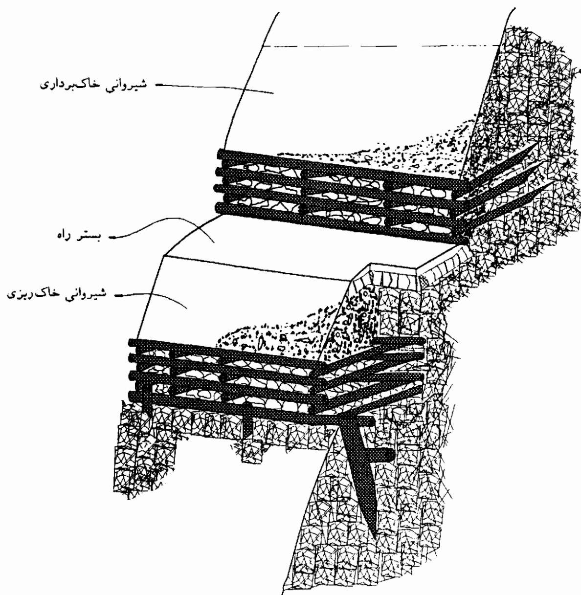
شکل ۴-۸- تثبیت شیروانی‌ها (برش و خاکریز) با مصالح چوبی
