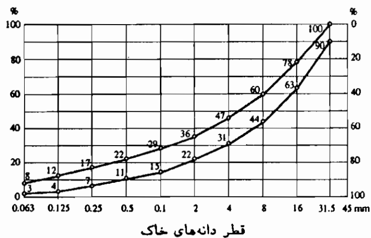
شکل ۳-۱۲ - منحنی‌های دانه‌بندی مناسب برای روسازی راه‌های جنگلی
