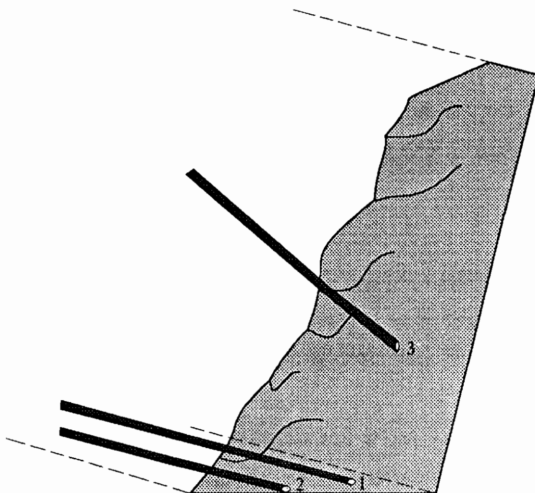
شکل ۳-۱۰ - روش انفجار افقی (باد بزنی)
