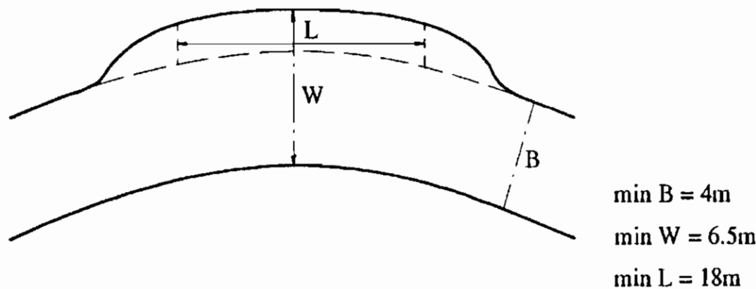
شکل (۲-۱۴) فرم و ابعاد گذرگاه درروی قوس
