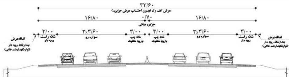
F۳- آزادراه شش خطه با DDHV کمتر از ۲۵۰
