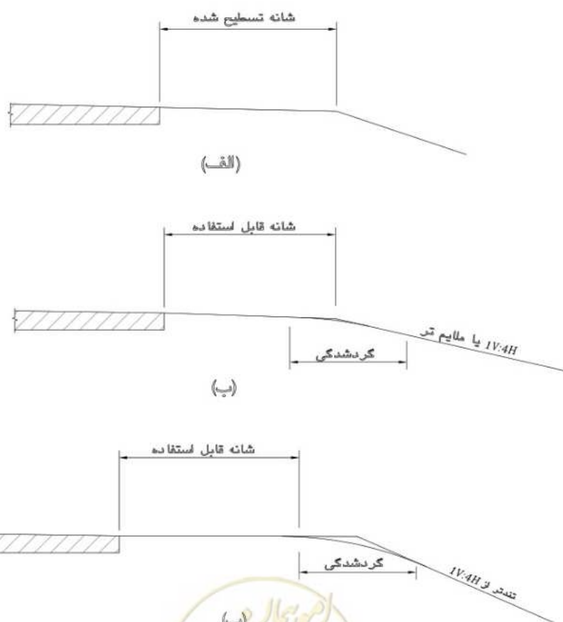
شکل ۶-۴- شانه های قابل استفاده و تسطیح شده
