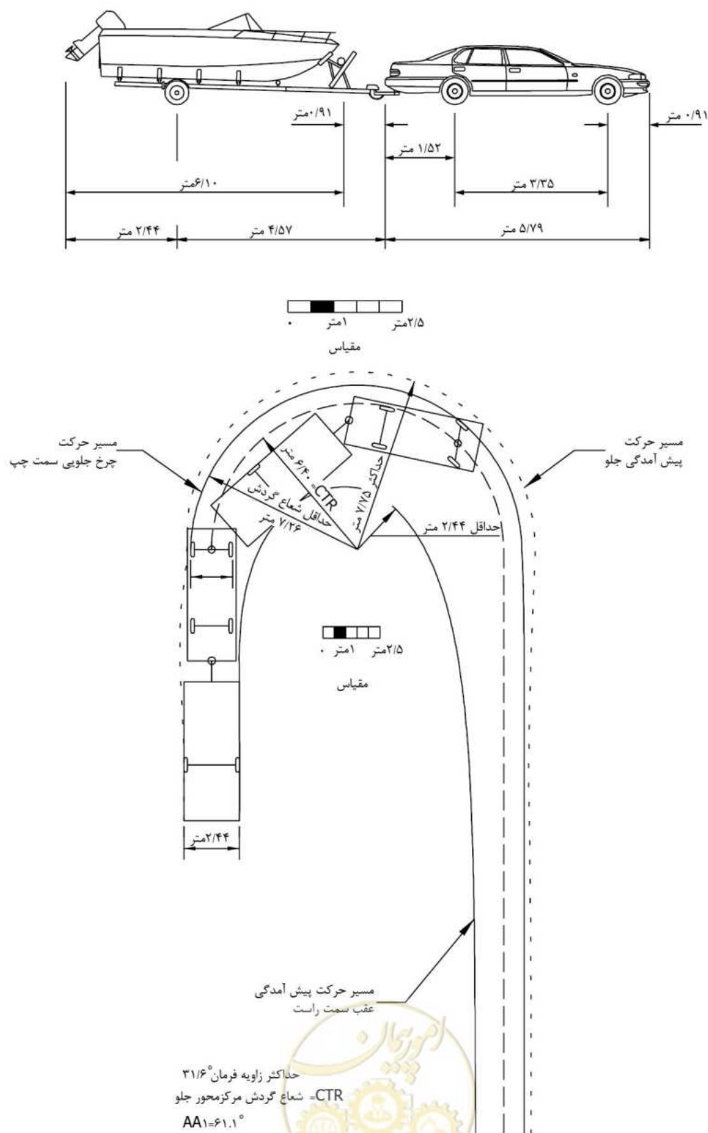
شکل ۴-۱۰- حداقل مسیر گردش برای وسیله طرح سواری با یدک قایق
