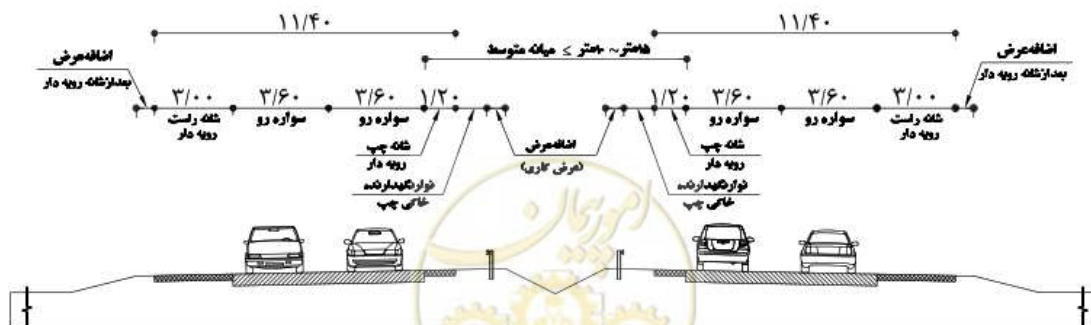
F۷- آزادراه چهار خطه با DDHV کمتر از ۲۵۰ با میانه متوسط
