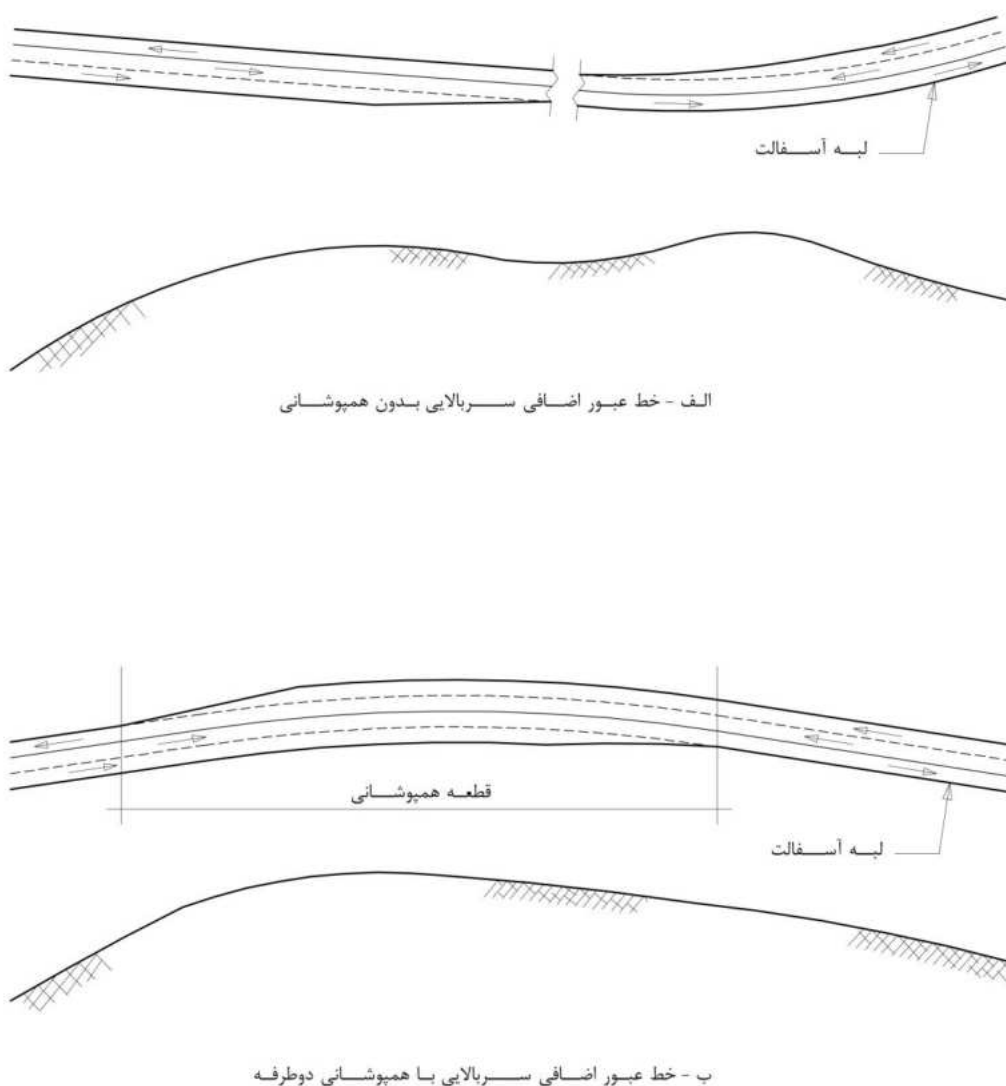
شکل ۵-۱۴ - خطهای کمکی سربالایی در راه های دو خطه دو طرفه
