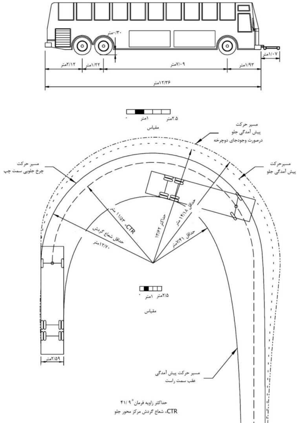
شکل ۴-۵- حداقل مسیر گردشی برای وسیله طرح اتوبوس نوع ۱
