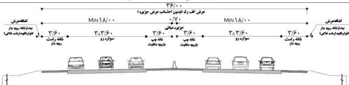
F۴- آزادراه شش خطه با DDHV برابر و بیشتر از ۲۵۰
