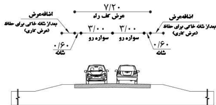
C۲- راه جمع کننده دو خطه با ADT بین ۲۵۰ تا ۴۰۰
