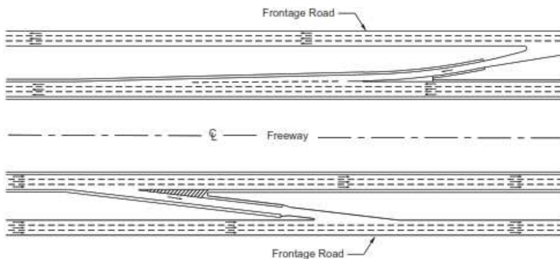
شکل ۶-۱۳- راه جانبی سه خطه یک طرفه در دو سمت آزادراه و رابط‌های کناری
