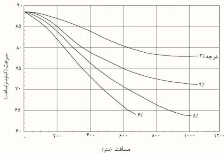
شکل ۵-۱۱- منحنی سرعت-مسافت وسیله نقلیه تیپ تفریحی
