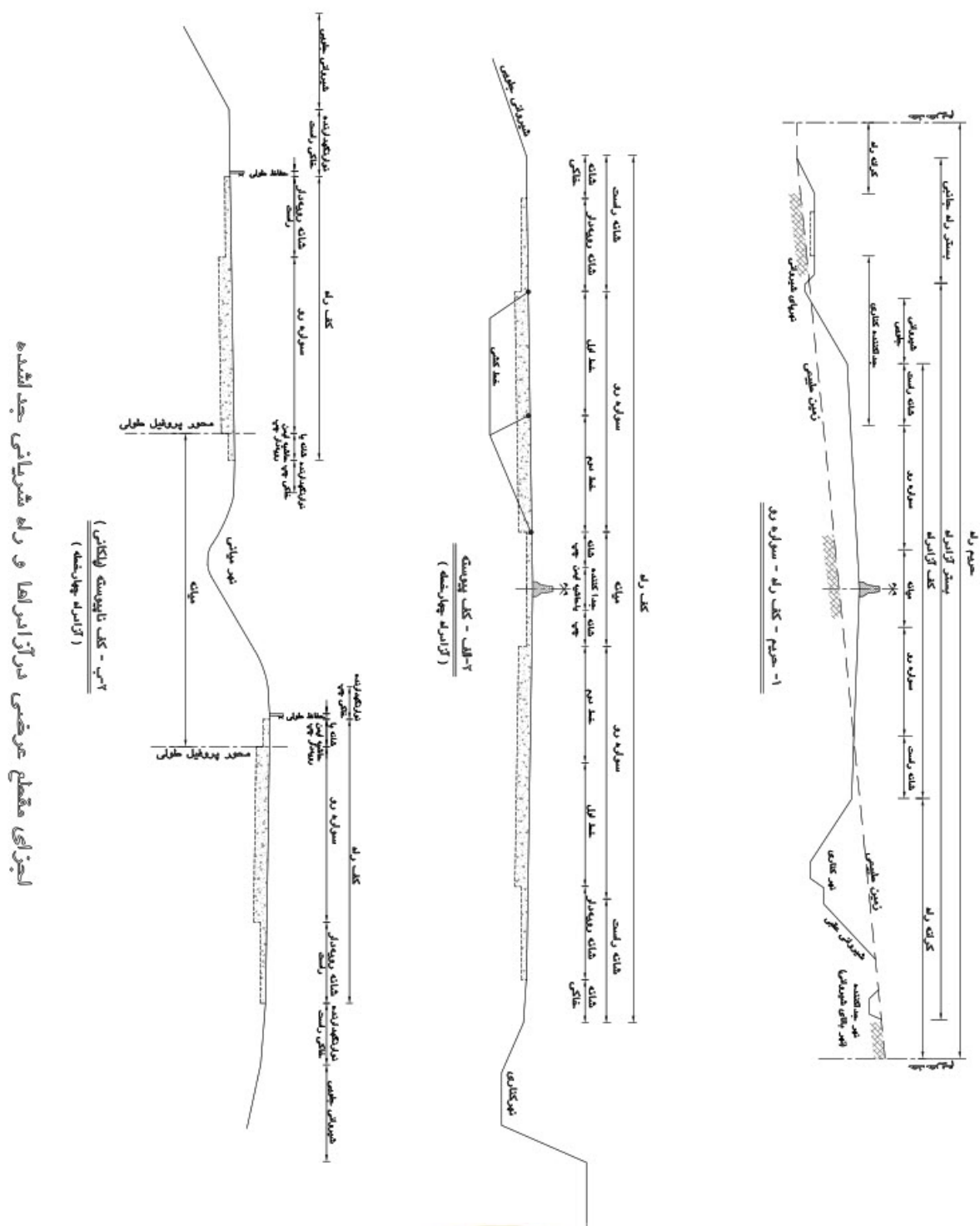
شکل ۶-۱- اجزای مقطع عرضی در آزادراه‌ها و راه شریانی جداشده
