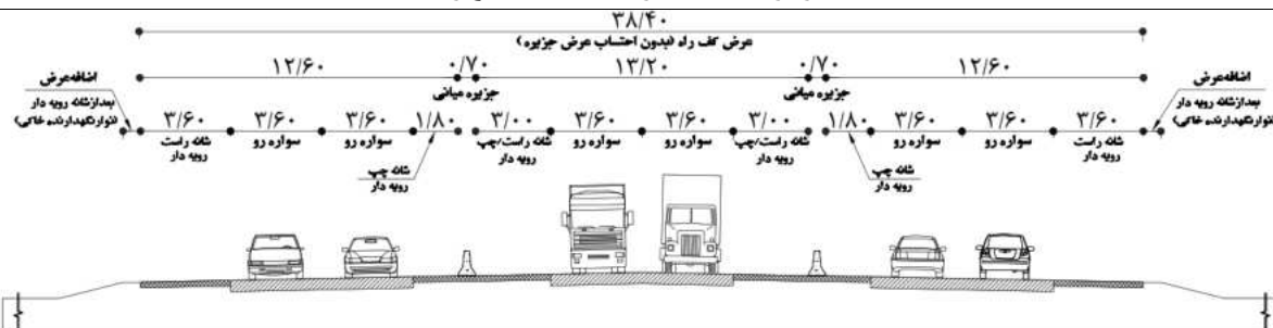
F۶- آزادراه با سه کف راه با DDHV برابر و بیشتر از ۲۵۰
