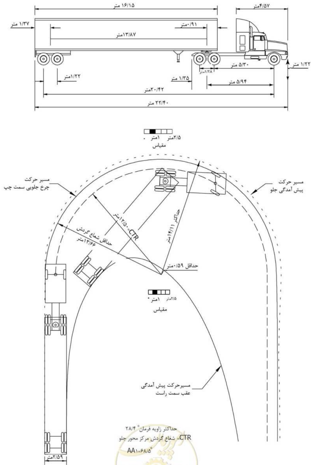
شکل ۴-۹- حداقل مسیر گردشی برای وسیله طرح تریلی نوع ۳
