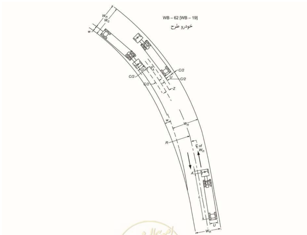
شکل ۵-۴- تعریض راه در قوس افقی
