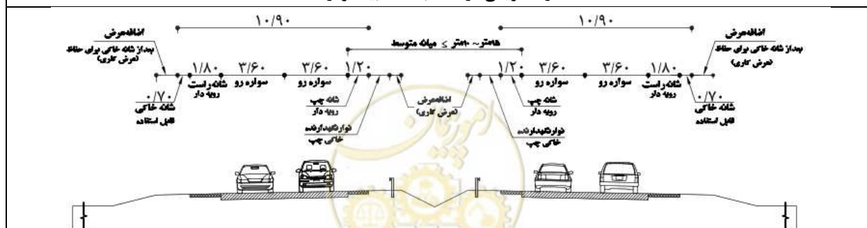
A۵- راه شریانی جداشده چهار خطه با میانه متوسط
