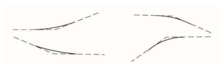
گردش‌دگی گوشه‌های سواره رو در محل اعمال بریلندی
