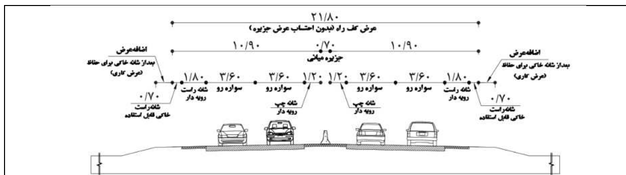
A۱- راه شریانی جداشده چهار خطه
