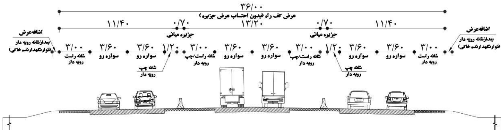
F۵- آزادراه با سه کف راه با DDHV کمتر از ۲۵۰
