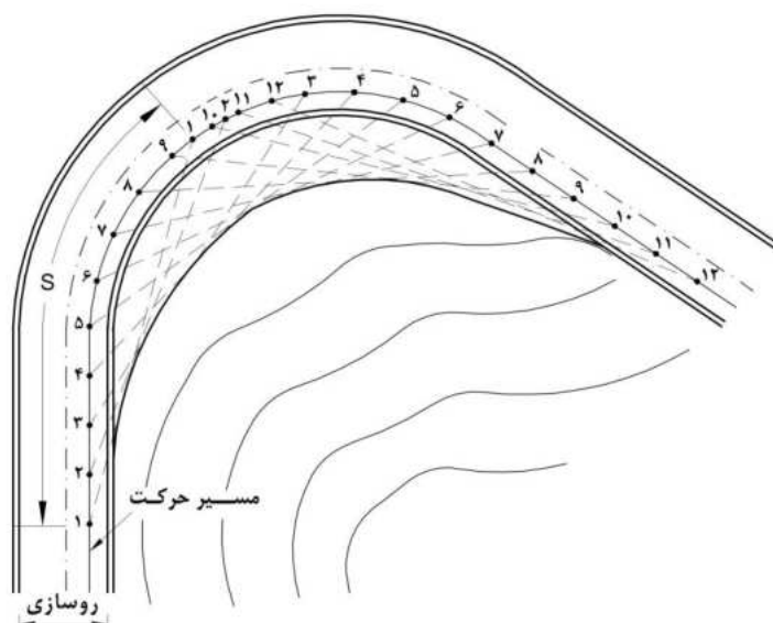
شکل ۵-۶- نحوه تعیین میزان بی‌مانع نمودن محوطه در قوس افقی
