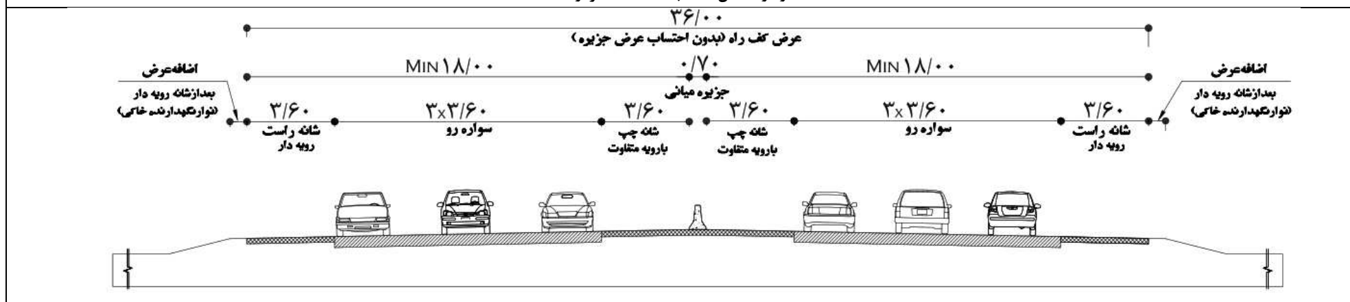
F۴- آزادراه شش خطه با DDHV برابر و بیشتر از ۲۵۰
