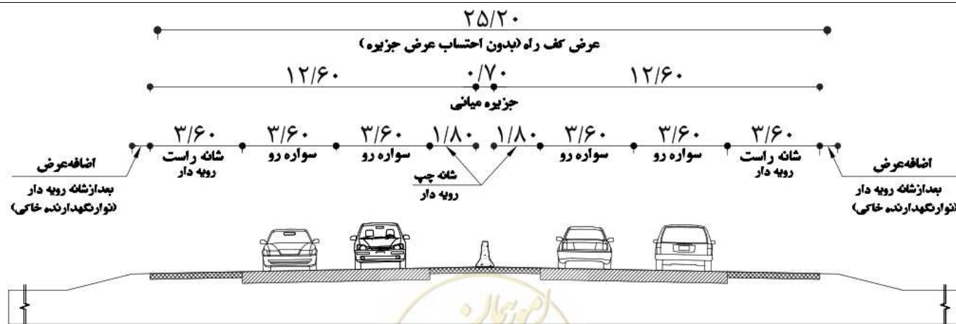
F2- آزادراه چهار خطه با DDHV برابر و بیشتر از ۲۵۰
