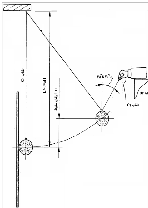
شکل ۳-۲- انجام آزمایش ضربه جسم سخت
