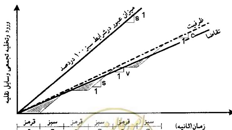
شکل ۵-۶- نمودار ورود و تخلیه وسایل نقلیه در یک ورودی تقاطع در حالت غیراشباع [۹۱]
