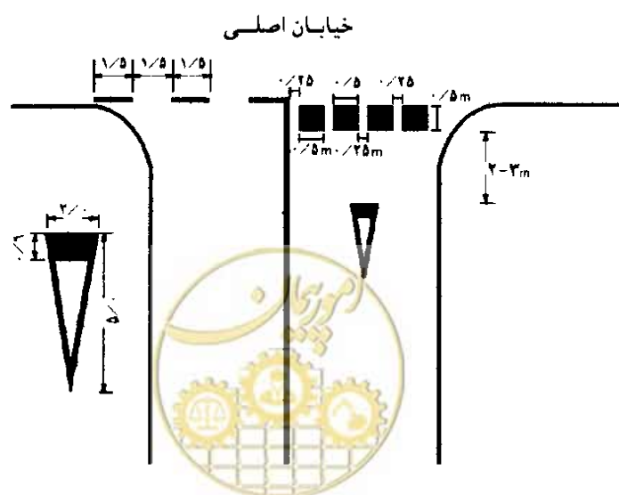
شکل ۴-۶۱- خط و مثلث رعایت حق تقدم عبور براساس دستورالعمل آلمان [۷۵]
