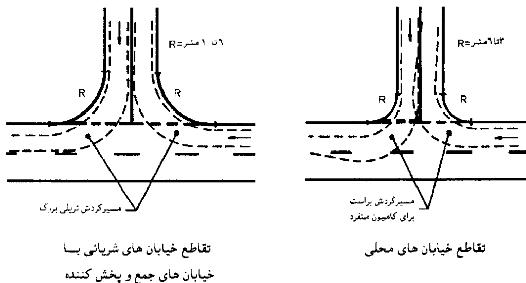
شکل ۳-۵۸- کاربرد قوس گوشه دایره ساده برای گردش به راست در تقاطع های شهری [۶۵]
