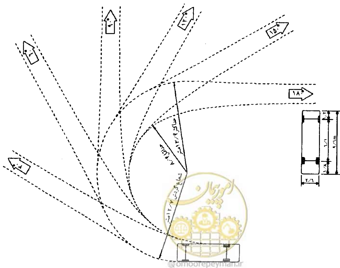
شکل ۳-۱۷- نمودار گردش نمای کامیون (متر) [۲۲]
