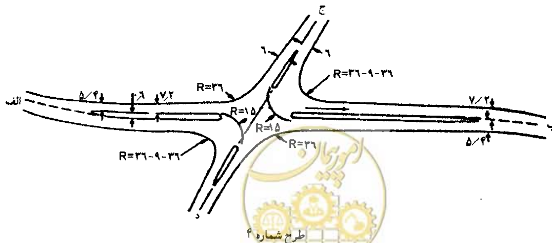
شکل ۳-۲- نمونه ای از طرح های اولیه یک تقاطع همسطح (متر)
