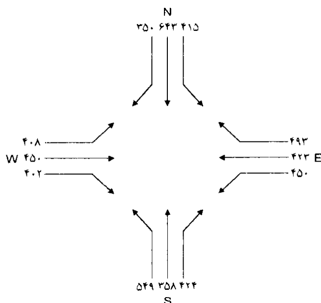
شکل ۵-۳۰- حجم تردد مسیرهای ورودی برحسب وسیله نقلیه سواری معادل در ساعت
