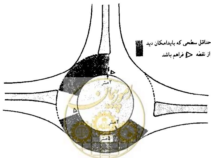
شکل ۳-۹۹- مسافت دید لازم در مسیر گردشی میدان
