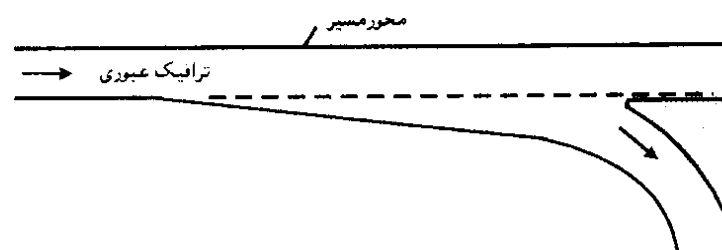
ب - خط کاهش سرعت اریب
