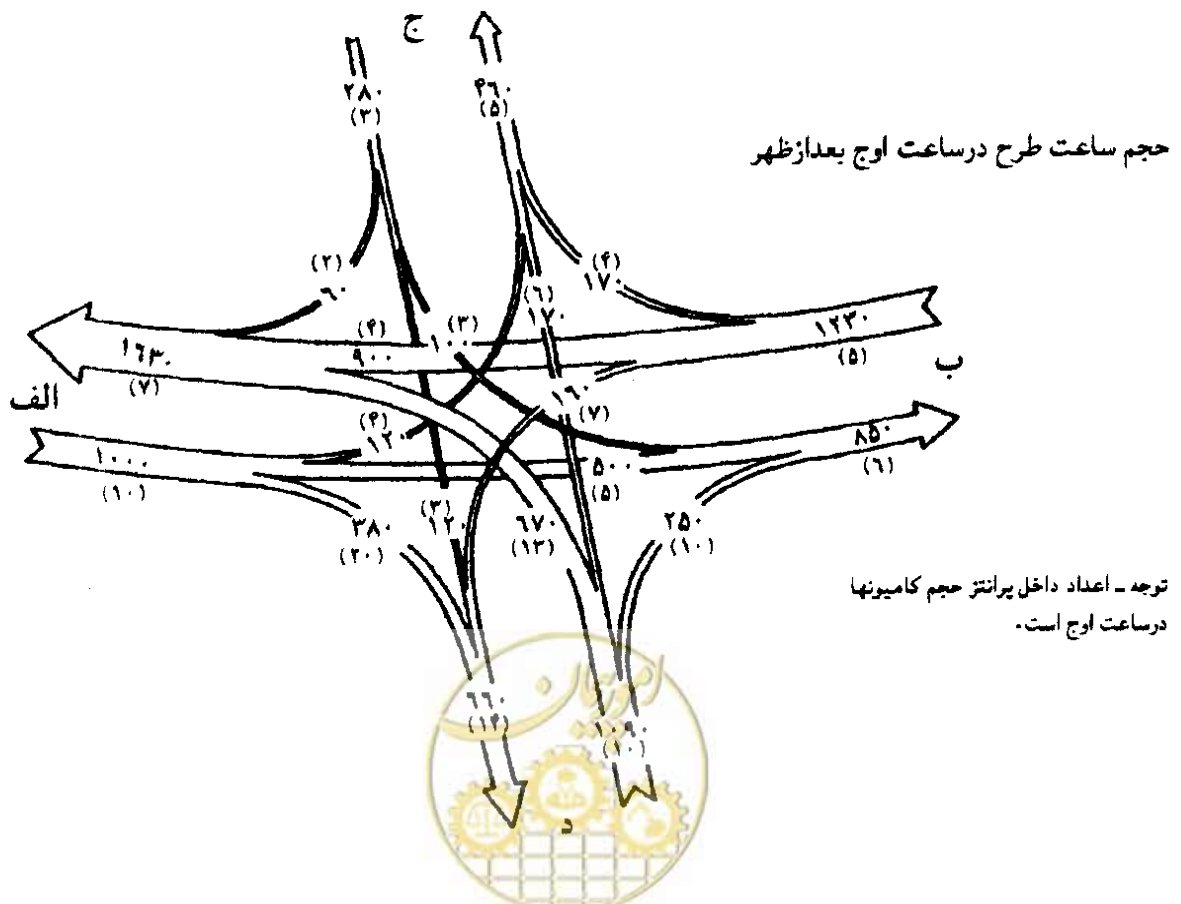
شکل ۲-۲- نحوه ارائه اطلاعات همزمان حجم ترافیک در تقاطع
