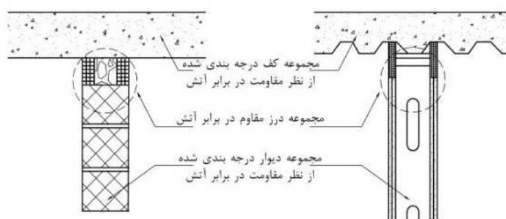
شکل ۱-۱۶- نمونه‌هایی از سیستم درزبندی آتش
