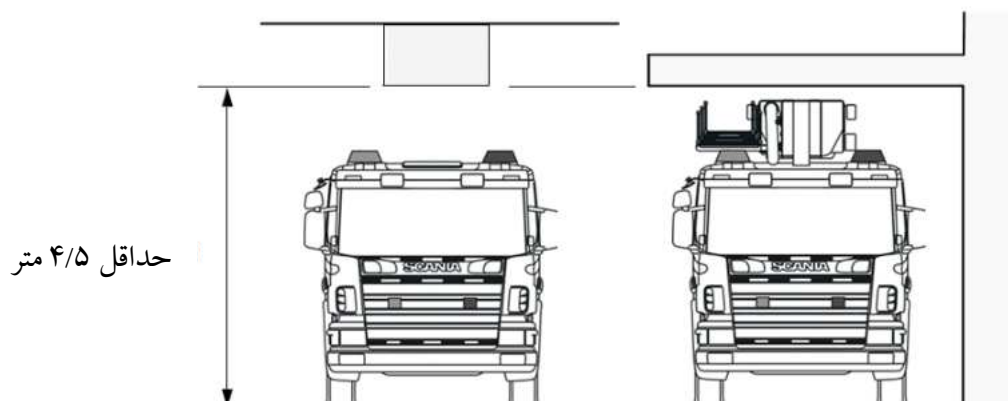
شکل ۱۴-۱- ارتفاع سر در برای عبور ماشین آلات آتش‌نشانی
