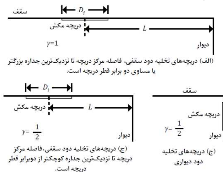
شکل ۱۰-۱۱- محاسبات پلاگ‌هولینگ
