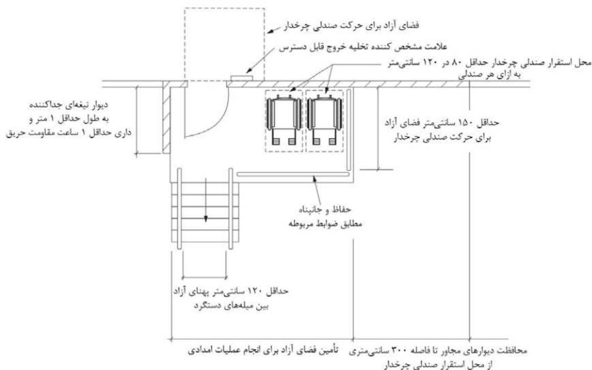
شكل ٦-٤٢- (الف): الزمات تخلیه خروج قابل دسترس (یلان)
