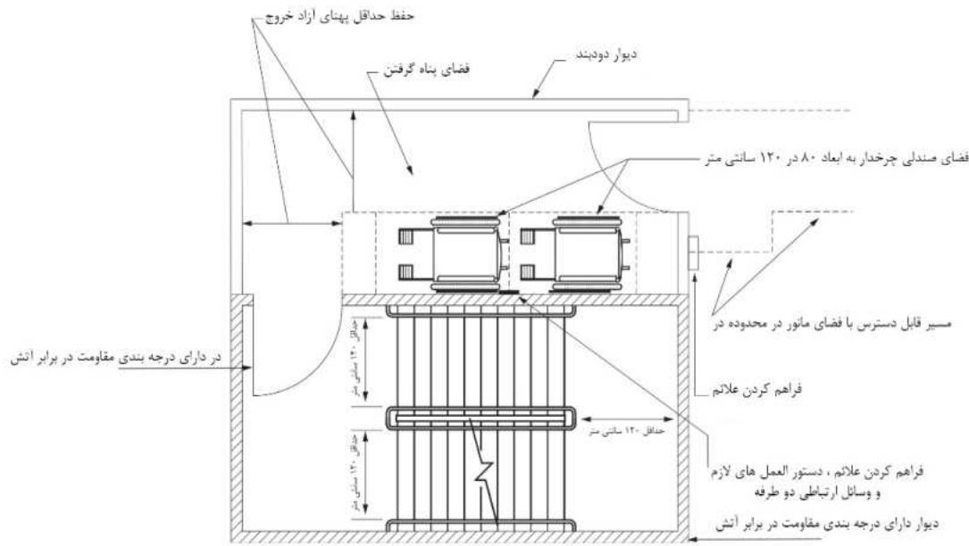
شکل ۶-۴۰-ب): راه‌پله در مجاورت فضای پناه گرفتن به عنوان راه خروج قابل دسترس
