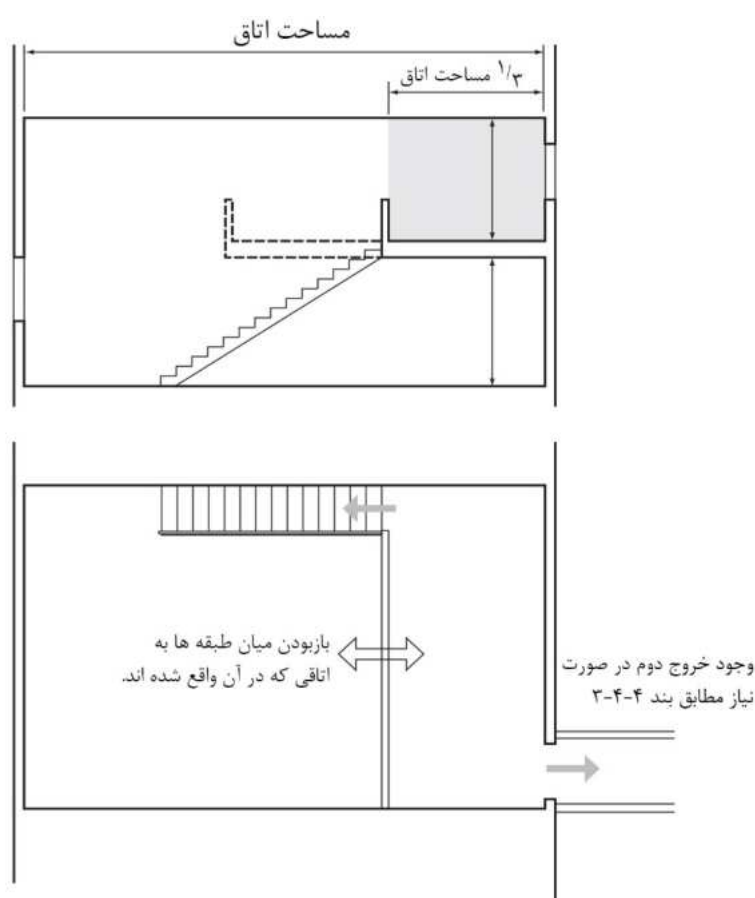
شکل ۴-۲- باز بودن میان طبقه‌ها و پیش بینی راه‌های خروج
