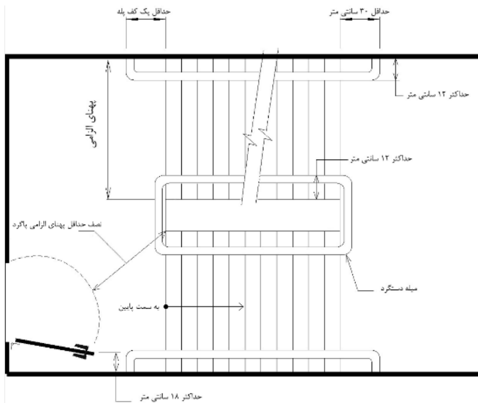
شکل ۶-۲۵- پیش‌آمدگی میله دستگرد در پلکان
