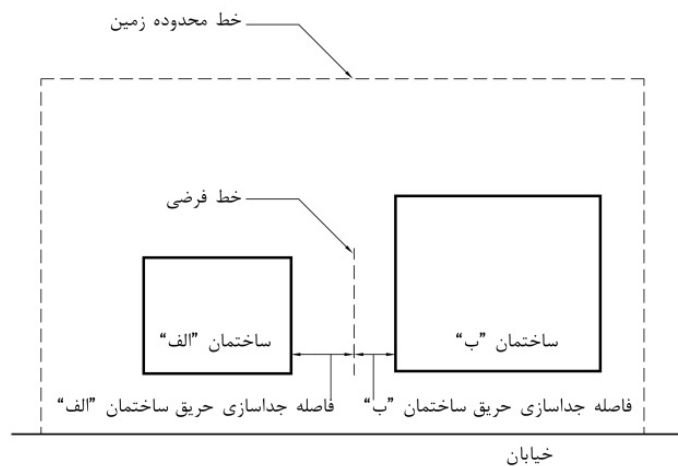
شکل ۱- ۲۷- اندازه‌گیری فاصله مجزاسازی حریق در خط فرضی بین دو ساختمان
