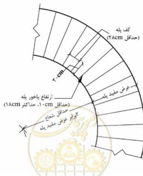
شکل ۶-۱۷- اندازه‌های مجاز پله قوسی
