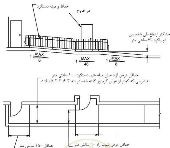
شکل ۶-۲۰- ابعاد و اندازه‌های مجاز شیب‌راه
