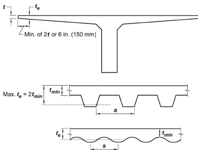
شکل ۸-۱۱- ضخامت معادل دیوارها و دال‌های بتنی لبه‌دار، کنگره‌دار و موجی شکل
