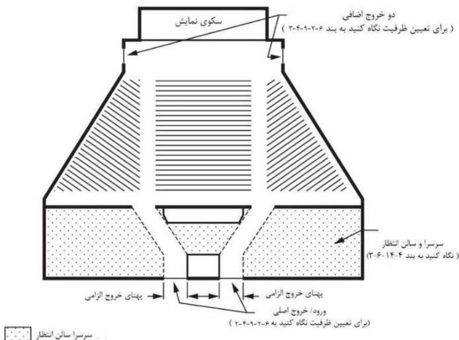
شکل ۶-۴۸- تصرف جمعی دارای فضای انتظار
