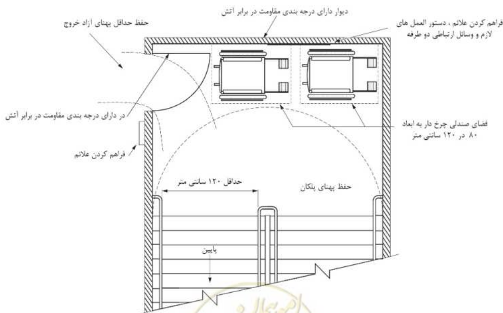
شکل ۴۰-۶ (الف): راه پله با پاگرد بزرگتر به عنوان راه خروج قابل دسترس
