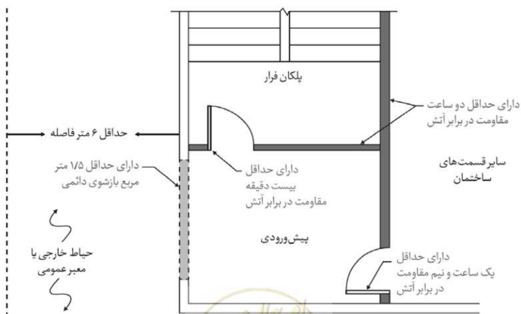
شکل ۱۰-۲- مشخصات پیش ورودی محافظت کننده یلکان با تهویه طبیعی
