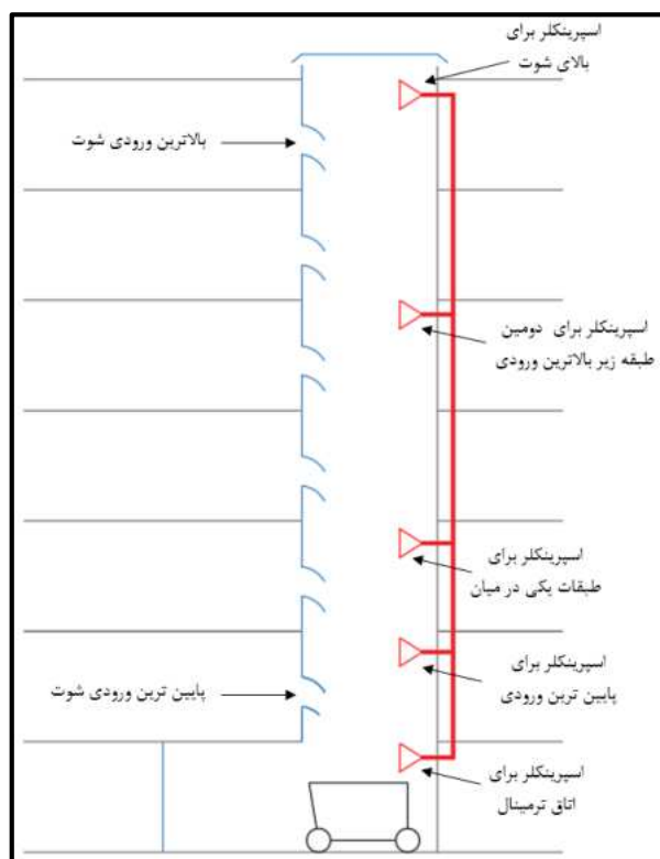
شکل ۹-۱۰- مثالی از استقرار اسپرینکلر در طبقات شوت زباله و لباس
