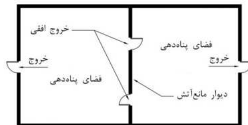
شکل ۱-۱۲- خروج افقی
