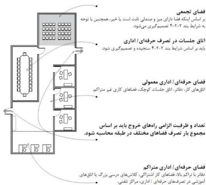
شکل ۲-۲-۲ مثال‌ها و توضیحاتی در خصوص فضاهای مختلف اداری / حرفه‌ای
