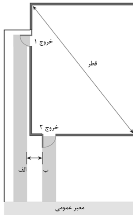
شکل ۶-۳۲- واگرایی تخلیه خروج‌ها و محاسبه فاصله بر اساس قطر طبقه
