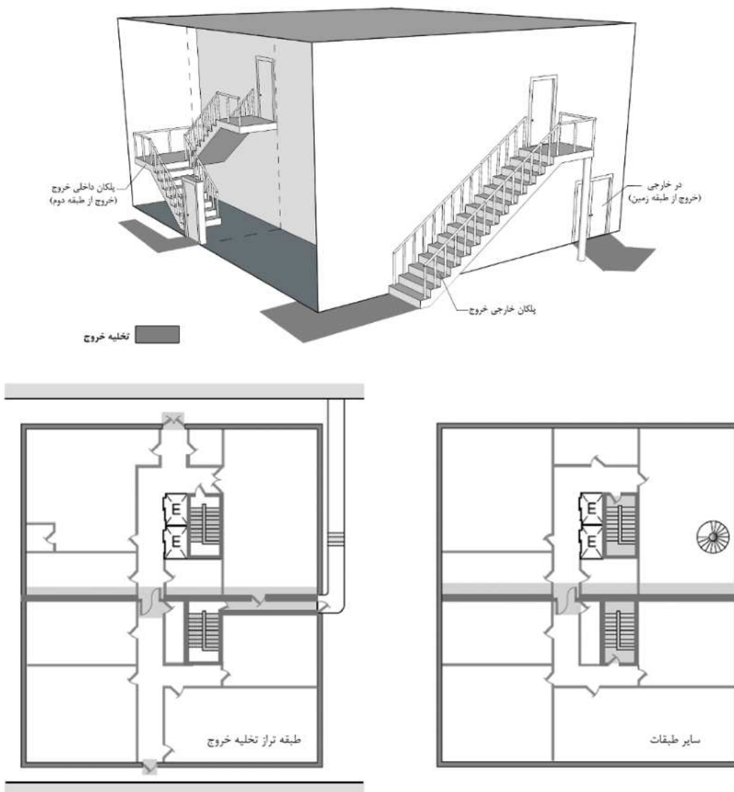
شکل ۶-۷- نمایش نمونه‌وار انواع خروج‌ها در پلان و به صورت سه‌بعدی،
