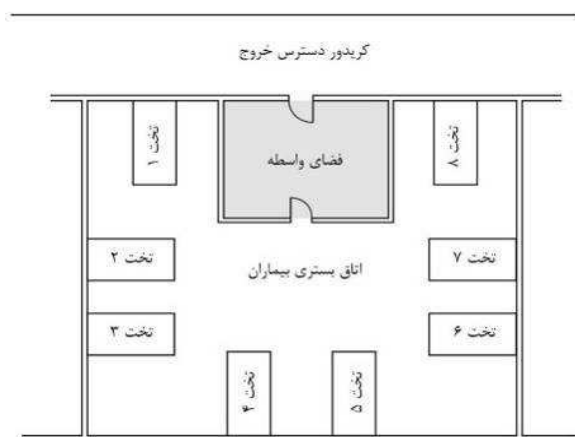
شکل ۶-۴۴- (ب) دسترسی با واسطه در اتاق‌های بستری با ظرفیت حداکثر ۸ تخت بستری
