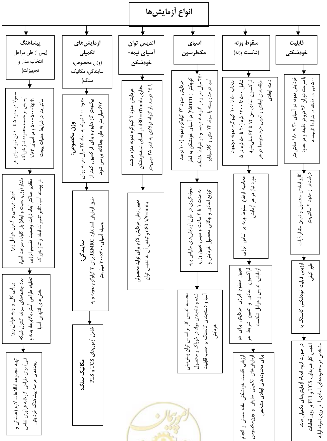
نمودار ۴-۱- نحوه انجام آزمایش‌های استاندارد آسیاهای خودشکن و نیمه‌خودشکن
