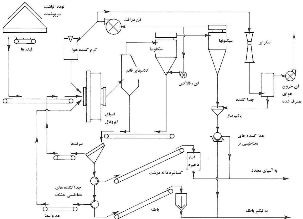
شکل ۴-۸- نمونه‌ای از مدار آسیای نیمه خودشکن در خردایش تر و در مقیاس پایلوت
