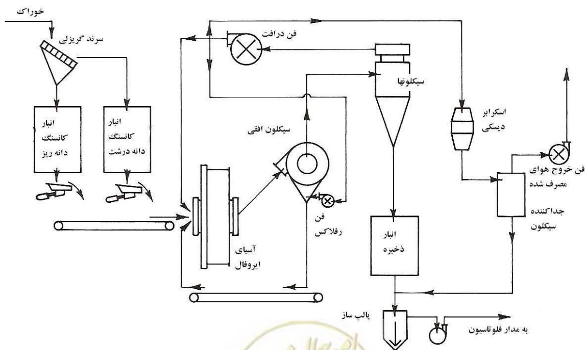
شکل ۴-۷- فلوشیت مدار آسیای ایروفال در مدار بسته
