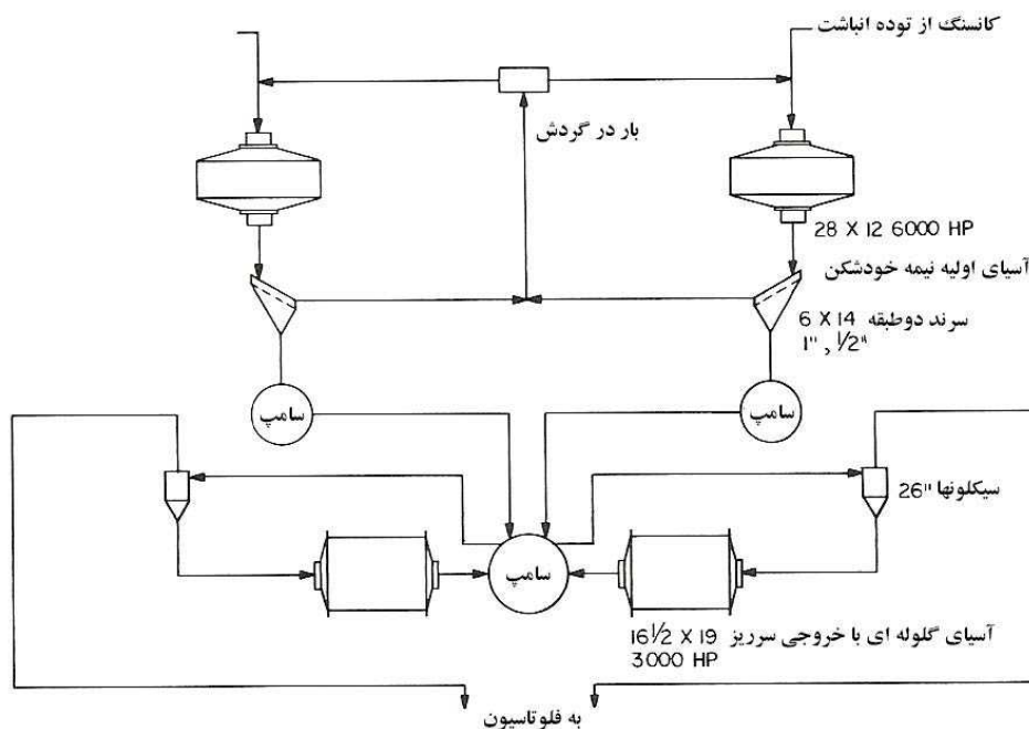
شکل ۴-۱۰- نمونه مدار آسیای نیمه‌خودشکن در شرایط تر و در دو خط موازی کانه‌آرایی
