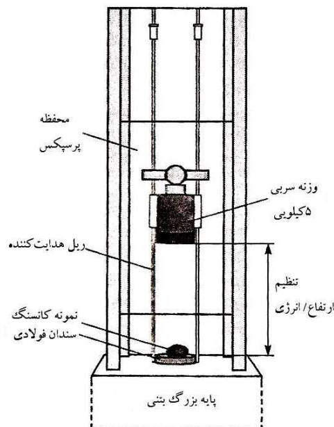
شکل ۴-۱-۲- تجهیزات آزمایش سقوط وزنه
