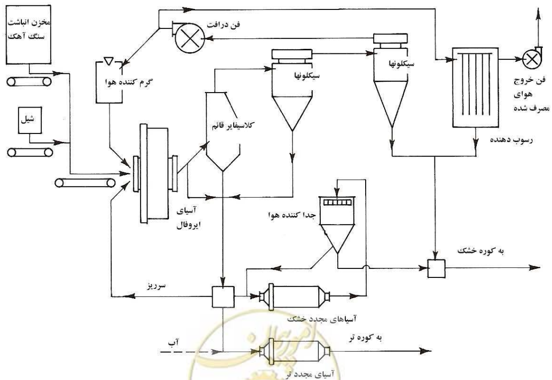
شکل ۴-۹- نمونه‌ای از مدار آسیای نیمه خودشکن در خردایش تر و در مقیاس پایلوت
