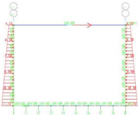
شکل ۱۰-۷۳- بار جانبی
