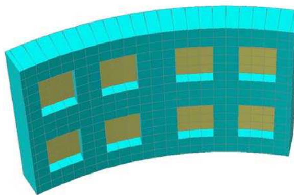
شکل ۱۰-۳۸- نمای پوشش داخلی سگمندی
