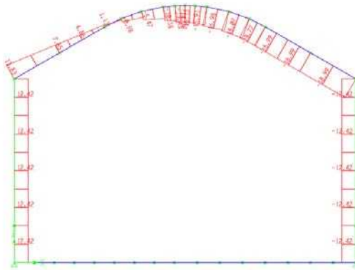
شکل ۱۰-۶۲- نیروی محوری ایجاد شده ناشی از بار زلزله
