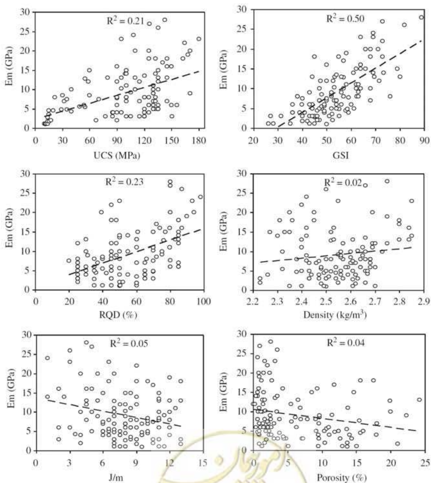
شکل ۶-۱۲- رابطه بین مدول تغییرشکل پذیری توده سنگ‌ها و پارامترهای غیروابسته [۱۵۱]
