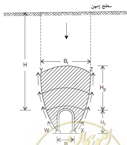
شکل ۶-۱- مفهوم بار سنگ در تونلها [۴۵]
