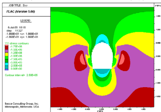
شکل ۸-۷- کننتور تنش Syy در اطراف تونل اصفهان- شیراز با استفاده از نرم افزار FLAC
