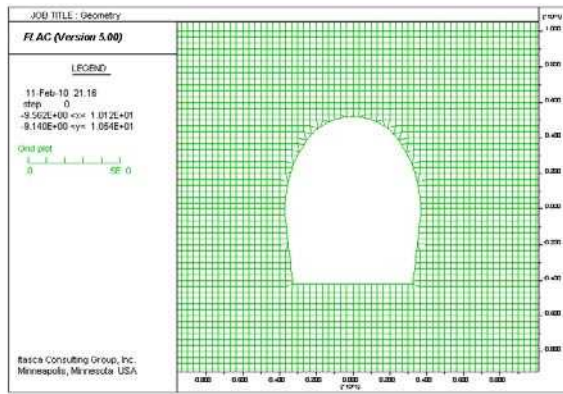
شکل ۸-۵- هندسه مدل عددی ساخته شده (قسمت Benching تونل اصفهان- شیراز با استفاده از نرم افزار FLAC)
