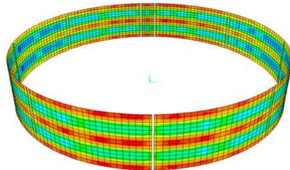
شکل ۱۰-۴۵- الگوی توزیع نیروی محوری در طول پوشش داخلی سگمنتی
