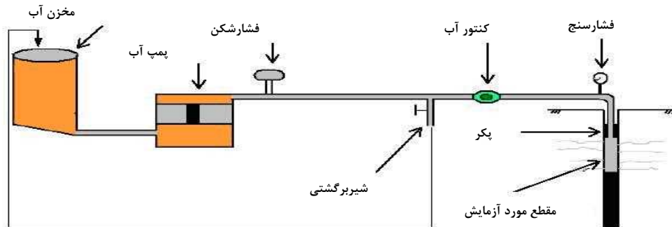
شکل ۴-۳۷- تجهیزات و نحوه اجرای آزمایش لوزان [۸۰]
