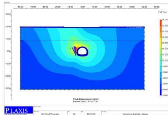
شکل ۱۰-۵۳- تغییر شکل
