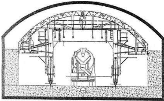
ب- نصب قالب لغزنده جهت بتن ریزی سقف تونل
