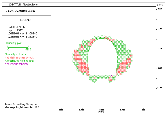
شکل ۸-۶- زون پلاستیک تشکیل شده در اطراف تونل اصفهان- شیراز با استفاده از نرم افزار FLAC
