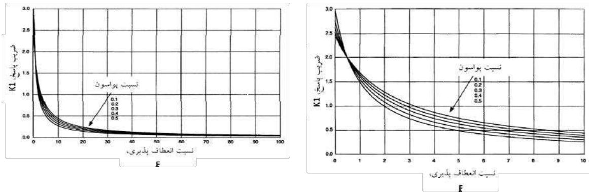
شکل ۹-۵- ضریب پاسخ پوشش داخلی تونل در مقابل نسبت انعطاف پذیری در شرایط لغزش کامل (تونل دایره ای) [۱۹۹]
