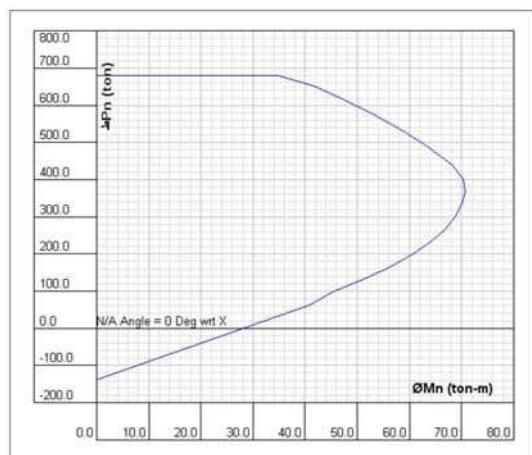
شکل ۱۰-۶۹- منحنی اندرکنش نیرو- ممان برای مقطع طراحی شده
