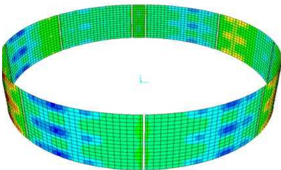
شکل ۱۰-۴۶- الگوی توزیع لنگر خمشی در طول پوشش داخلی سگمنتی
