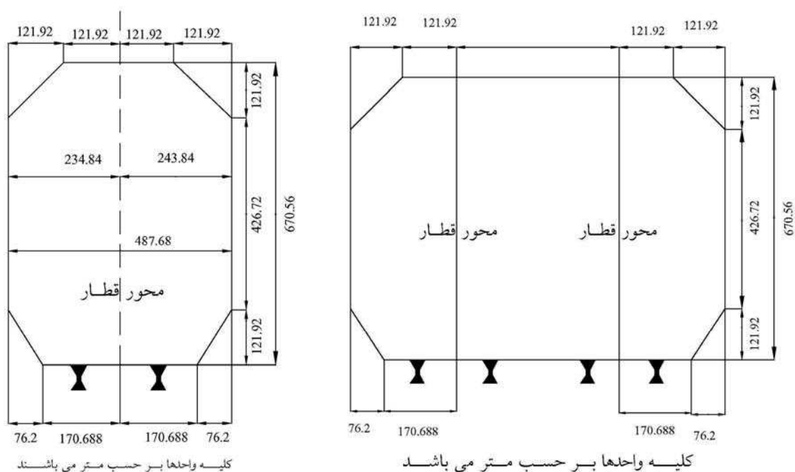
شکل ۲-۱۵- مقطع عرضی و حداقل فضای مفید تونل‌های راه آهن طبق توصیه انجمن مهندسين راه آهن آمريكا [۱۱]
