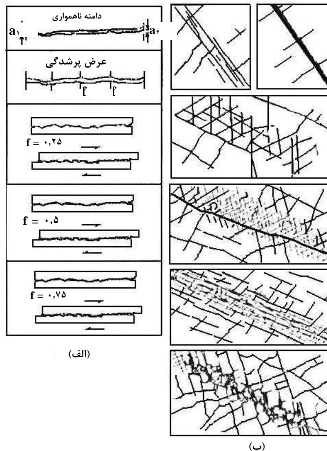
شکل ۴-۱۹- انواع پرشدگی ناپیوستگی‌ها (الف) در حالت پرشدگی ساده، عرض پرشدگی و دامنه ناهمواری سطح ناپیوستگی می‌تواند برای برآورد مقدار جابجایی برشی تا حد رسیدن به تماس سنگ به سنگ به کار آید ( a =دامنه ناهمواری، f =عرض پرشدگی) (ب) طرح‌های شماتیک از پرشدگی مرکب ناپیوستگی‌های سنگ [۶۳]
