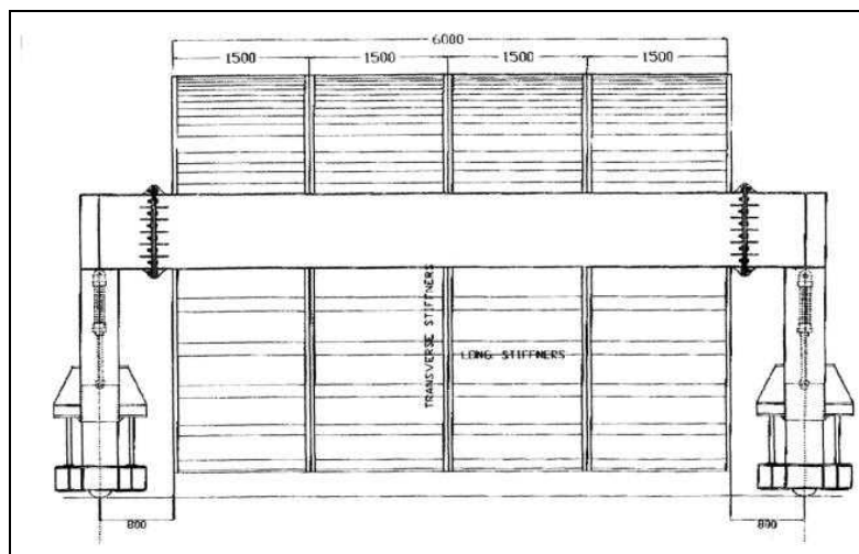
شکل ۱۳-۱۱- نماهایی از قالب لغزنده
