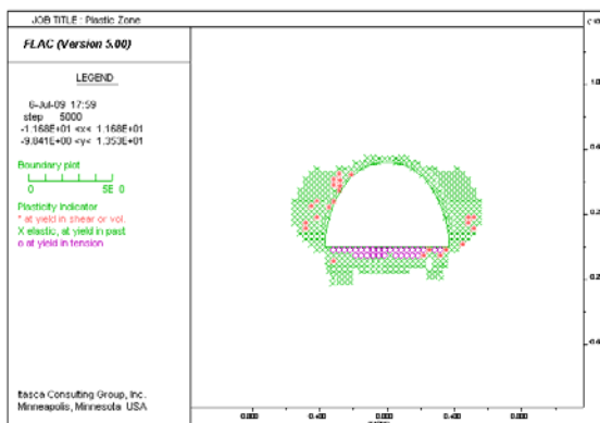
شکل ۸-۳- زون پلاستیک تشکیل شده در اطراف تونل اصفهان - شیراز با استفاده از نرم افزار (Top heading) FLAC
