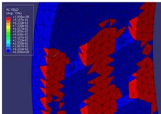
شکل ۳۱-۱۰- تسلیم در نزدیکی محفظه بولت‌ها
