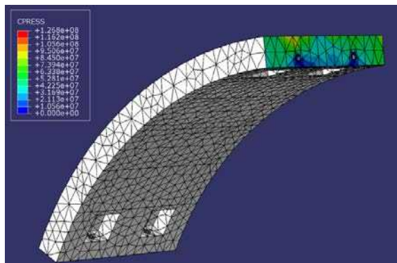
شکل ۱۰-۳۷- فشار در سطح تماس بین دو سگمنت
