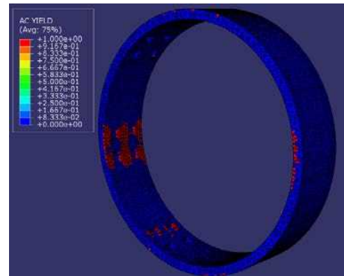
شکل ۳۰-۱۰- مناطق تسلیم شده رینگ تحت بارهای وارده
