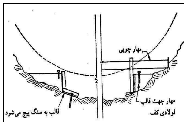
شکل ۱۳-۱۲- قالببندی و بتن ریزی جدولها
