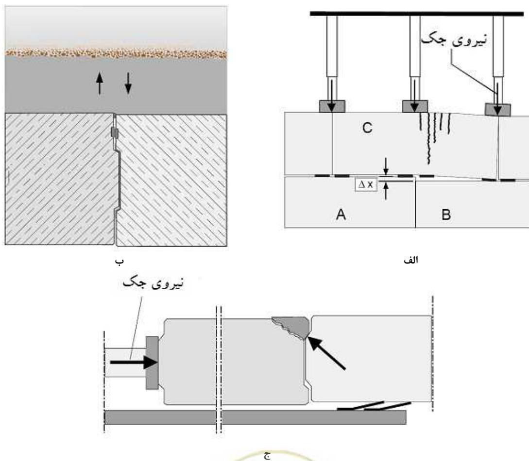
شکل ۱۲-۳۸- آسیب دیدگی سگمنت در حین پیشروی TBM در اثر الف) فشار جک‌های پیشرو، ب) فشار تزریق، ج) جاافتادگی
