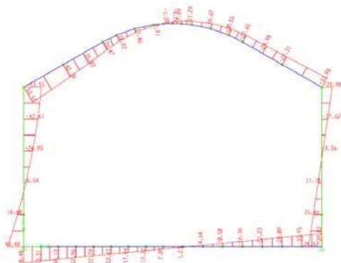
شکل ۱۰-۶۷- خمش ناشی از بار مرده
