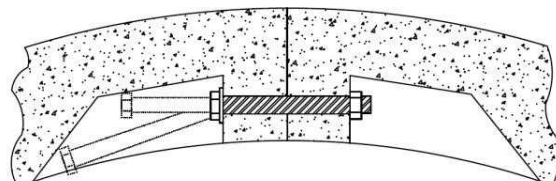
نمونه‌ای از بولتهای مستقیم (بولت یک مهره ای) [۲۲۸]
