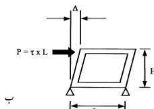
شکل ۹-۸- سختی نسبی خاک و یک قاب مستطیلی [۱۸۶]
