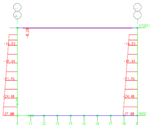
شکل ۱۰-۷۷- نیروی محوری ایجاد شده بر اثر بار مرده
