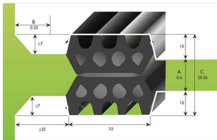
یک نوع نوار آبی‌بند (واحدها بر حسب میلی‌متر)
