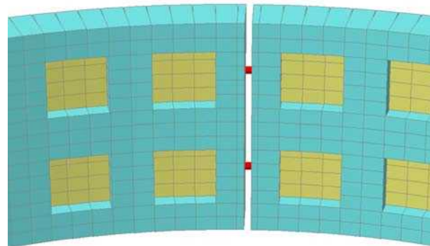
شکل ۱۰-۴۲- الگوی مدلسازی بولتهای موجود بین سگمنتها
