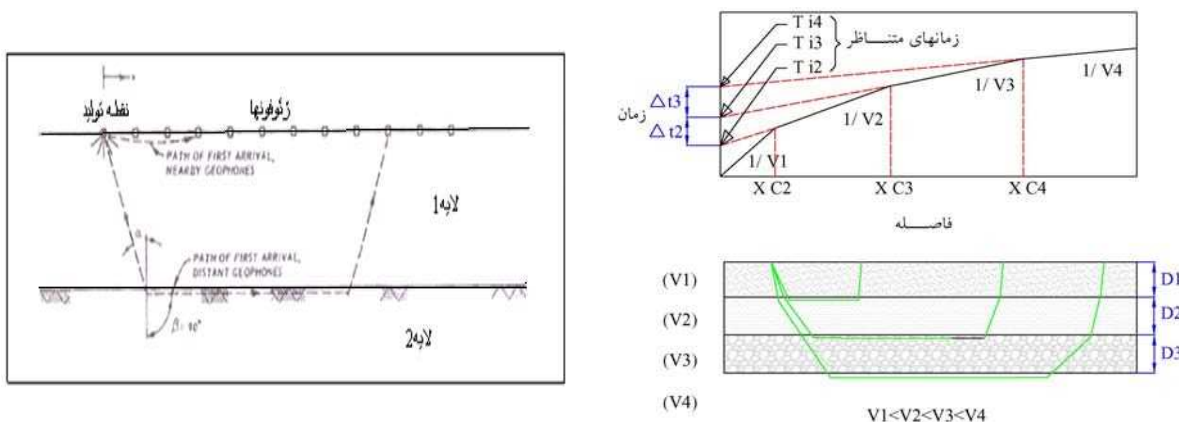
شکل ۴-۴۹- نمای شماتیک از چگونگی تولید و ثبت امواج لرزه ای [۹۵]
