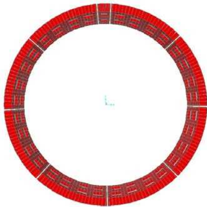
شکل ۱۰-۴۳- مدلسازی پوشش داخلی سگمنتی بصورت منفصل با قرار گیری کلید در سقف تونل
