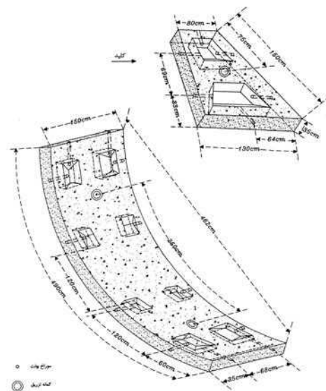
ج- نمایی از یک قطعه سگمتی و یک کلید سگمتی
