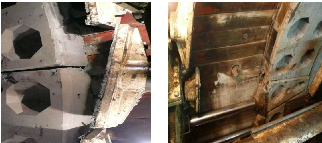
شکل ۱۲-۳۷- نمایی از آسیب دیدگی سگمنت در حین پیشروی TBM
