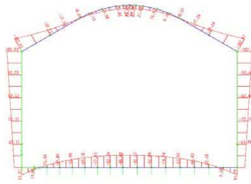
شکل ۱۰-۶۶- خمش ناشی از بار زلزله
