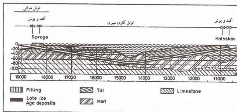
شکل ۱۵-۱۵- نیمرخ طولی زمین شناسی تونل استوربلت جدول ۹-۱۵- مشخصات عمومی پوشش تونل استوربلت
