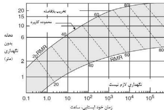
شکل ۴-۶- زمان خود ایستایی بر حسب دهانه سقف برای کلاسهای
