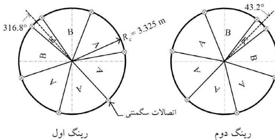
شکل ۱۰-۱۶- مشخصات لاینینگ سگمتی و محل فرار گیری اتصالات رینگ [۲۲۰]
