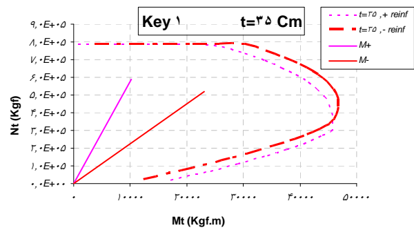
شکل ۱۰-۴۹- نمودار اندرکنش نیروی محوری - ممان در مقطع ضخیم پوشش داخلی سگمندی
