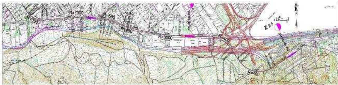
شکل ۴-۴- یک نمونه نقشه توپوگرافی و مسیر راه آهن شهری طراحی شده بر اساس آن
