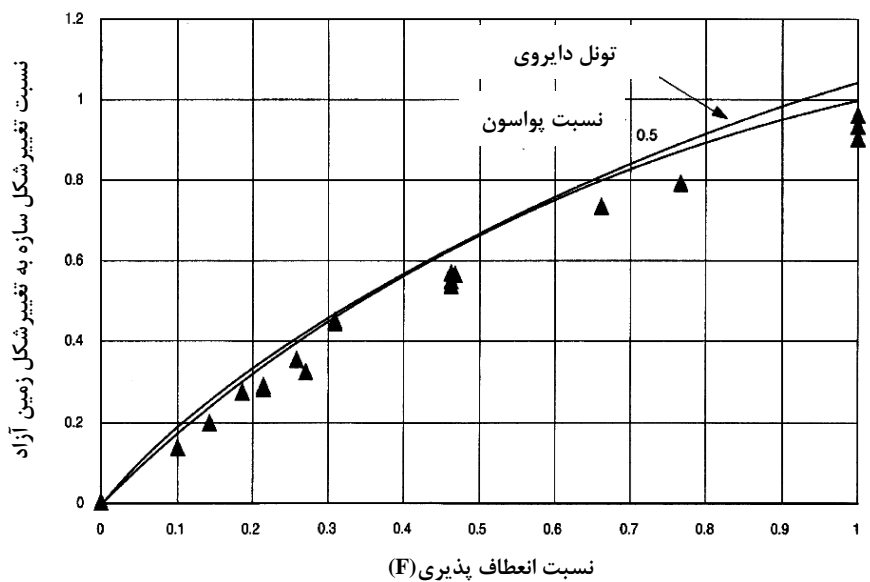
شکل ۹-۱۰- مقایسه تغییر شکل سازه ای بی بعد شده در مقابل نسبت انعطاف پذیری برای تونل‌های مستطیلی و دایره ای [۱۹۶] اشکال مثلثی برای تونل‌های مستطیلی شکل می‌باشند خطوط برازش شده برای تونل‌های دایره ای شکل می‌باشند
