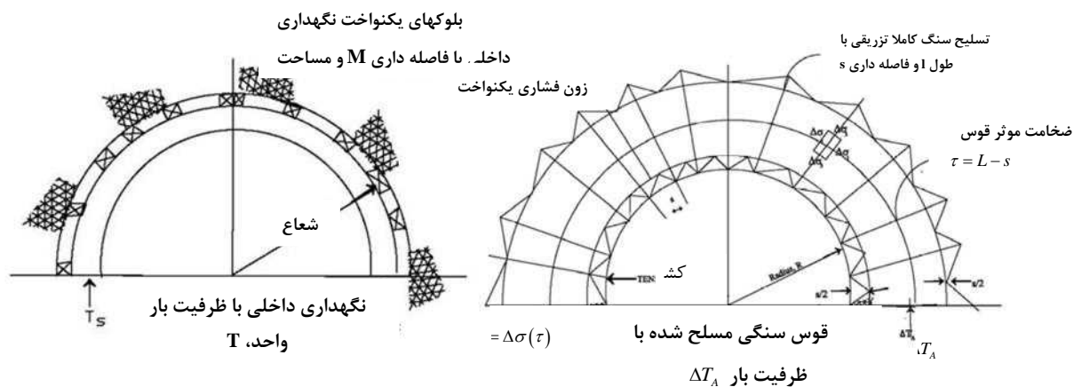
شکل ۷-۹- قوس سنگی مسلح شده
