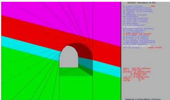
شکل ۸-۱۴- نمای سه بعدی تونل ۴ غربی معدن زغالسنگ پروژه ۵ طیس با استفاده از نرم افزار 3DEC
