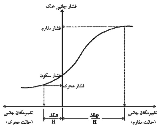
شکل ۱۰-۷- تغییرات فشار جانبی خاک در مقابل تغییر مکان سازه در حالات مختلف [۲۱۵]
