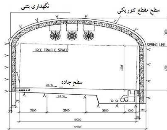
الف- مقطع بخش تونلی تونل کرک
