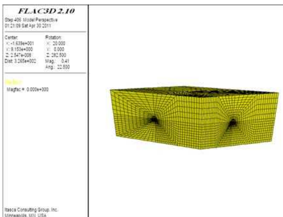
ب- هندسه مدل عددی ساخته شده تقاطع تونل ۴ غربی معدن زغالسنگ پروده ۵ طیس با استفاده از نرم افزار FLAC 3D
