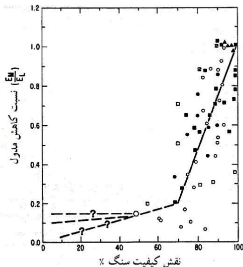
شکل ۶-۱۱- ارتباط بین RQD و نسبت مدول توده سنگ به بکر [۱۲۶]
