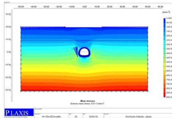
شکل ۱۰-۵۱- تنش اصلی
