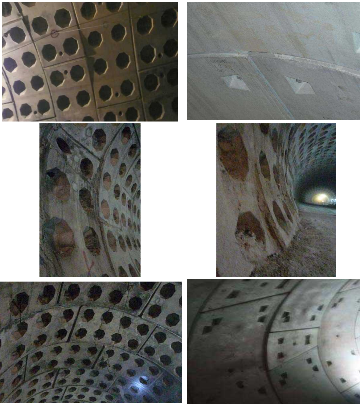
شکل ۱۲-۳۰-نمایی از بیرون زدگی سگمنت در اثر عدم نصب مناسب اتصالات
