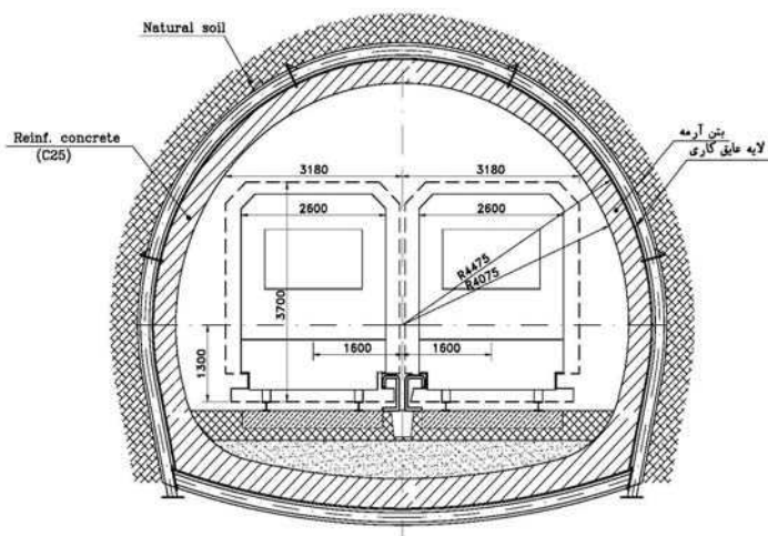
شکل ۲-۴-ب - تونل راه آهن دو خطه با مقطع نعل اسبی پس از کف سازی
