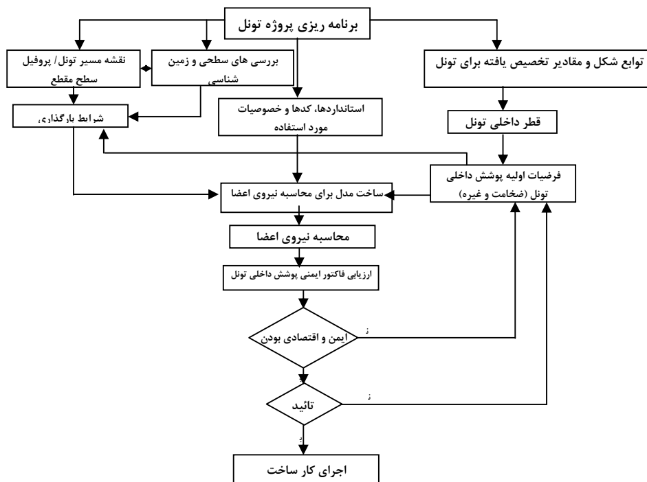
شکل ۱۰-۱- فلوجارت طراحی پوشش داخلی تونلها [۲۰۳]
