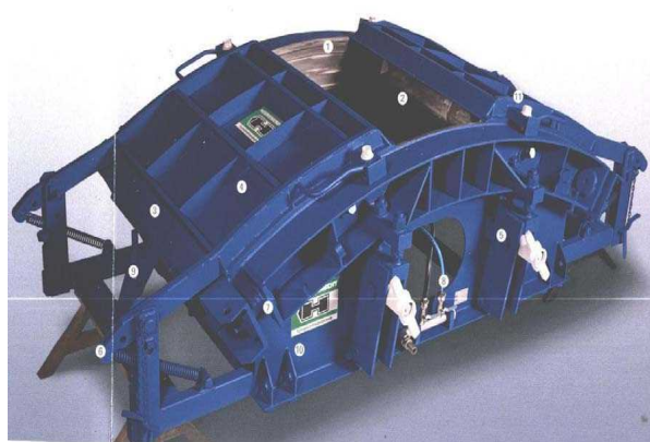
نمایی از قالب آماده شده برای جایگذاری قفسه آرمانتور و بتن ریزی [۲۳۰] شکل ۱۲-۱۲- مراحل ساخت و آماده کردن قالب برای تولید قطعات سگمندی
