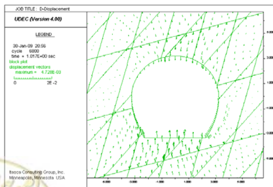
شکل ۸-۱۱- بردارهای جابجایی در اطراف تونل زاب با استفاده از نرم افزار UDEC
