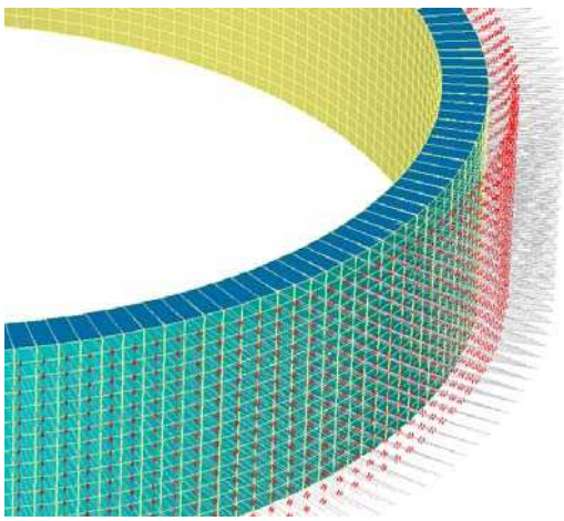
شکل ۱۰-۴۴- نحوه مدلسازی خاک اطراف توسط المانهای غیر خطی link
