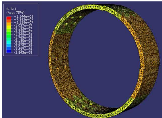
شکل ۲۹-۱۰- تنش S11
