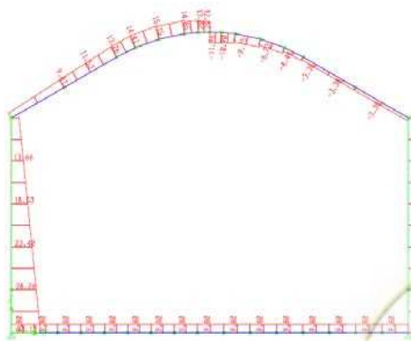
شکل ۱۰-۶۵- نیروی برشی ناشی از بار زلزله
