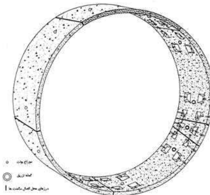
ب- نمای سه بعدی از یک رینگ سگمتی (۵+۱)
