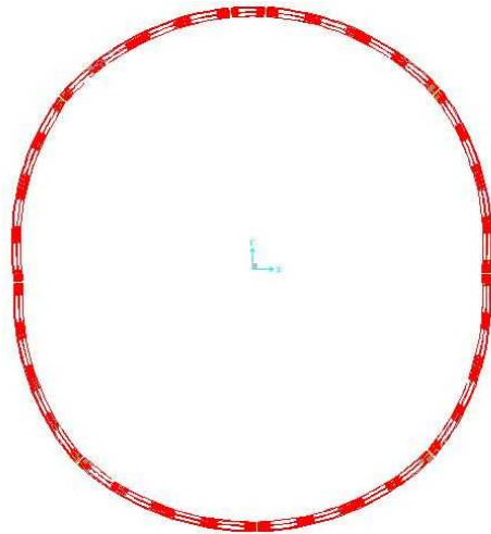
شکل ۱۰-۴۸- تغییر شکل ایجاد شده روی پوشش داخلی سگمندی
