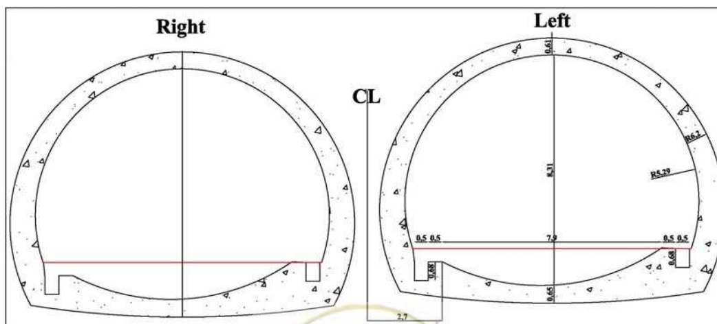
شکل ۲-۵ - تونلهای راه یک طرفه با مقطع نعل اسبی
