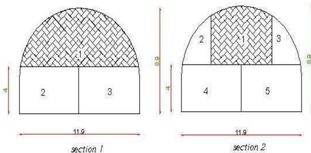
شکل ۱۲-۱۵- مقاطع حفاری تونل، (Section ۱) طبق طراحی و (Section ۲) در اجرا
