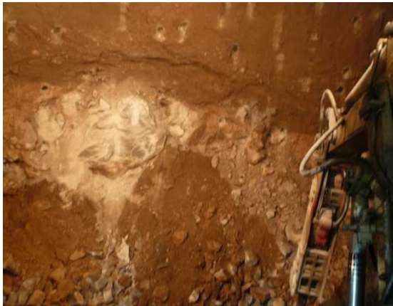
لایه سنگ در ارتفاع چهار متری از مقطع سینه کار تونل در کیلومتر حدود ۱۷+۹۵۰ (بر اساس شکل ۴-۶۰)
