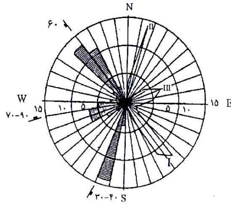
شکل ۴-۱۴- دو روش نمایش داده‌های مربوط به جهت داری در نمودار گلسرخی [۶۳]
