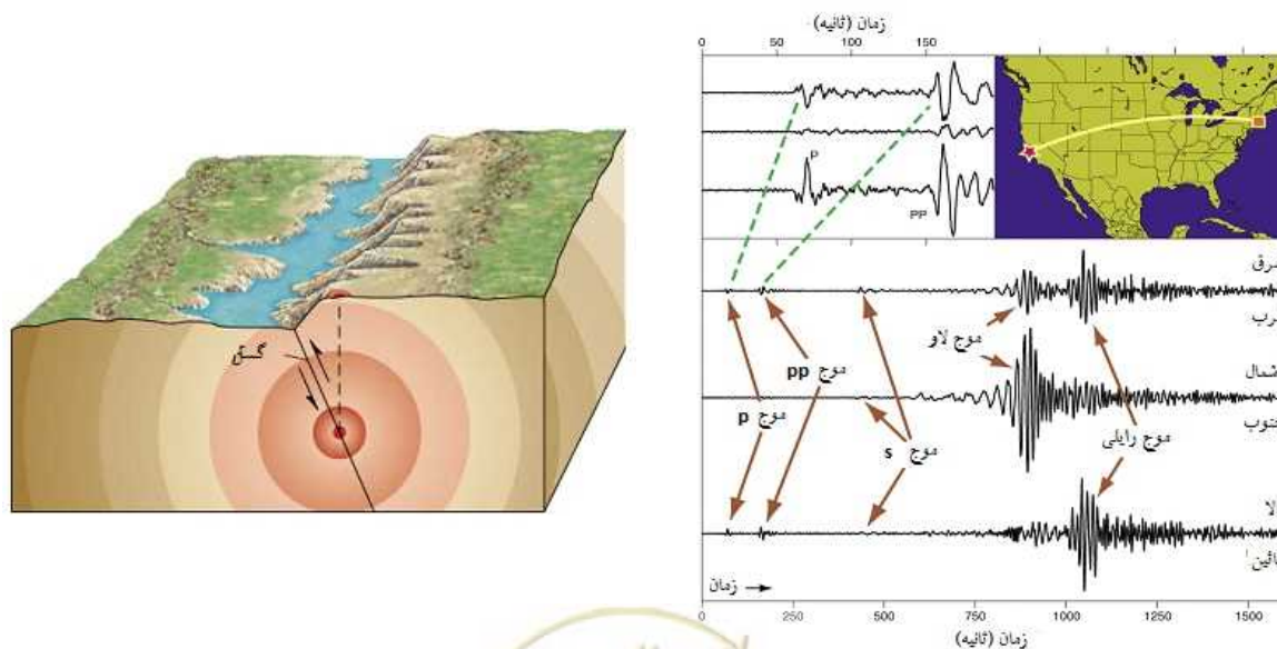
شکل ۳-۴۴- نحوه ثبت امواج مختلف زمین لرزه توسط
