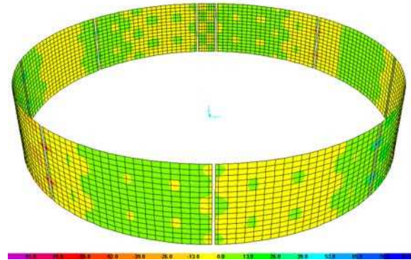
شکل ۱۰-۴۷- الگوی توزیع نیروی برشی در طول پوشش داخلی سگمندی
