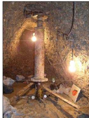
آزمایش بارگذاری صفحه‌ای عمودی
