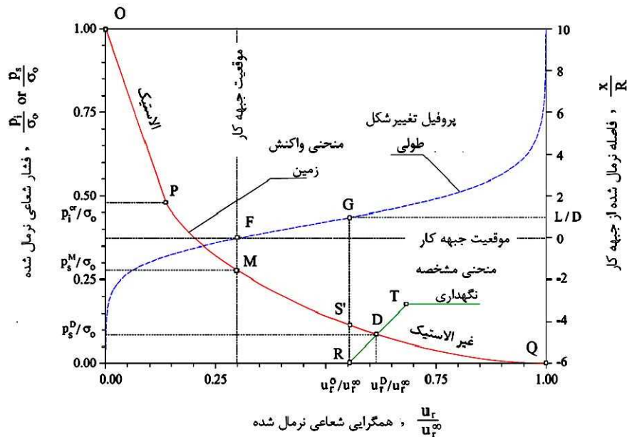
شکل ۷-۲- نمایش شماتیک منحنی واکنش زمین، منحنی مشخصه سیستم نگهداری، پروفیل تغییر شکل طولی [۱۶۱] P_i : فشار زمین، P_s : فشار نگهداری، u_r : جابجایی شعاعی
