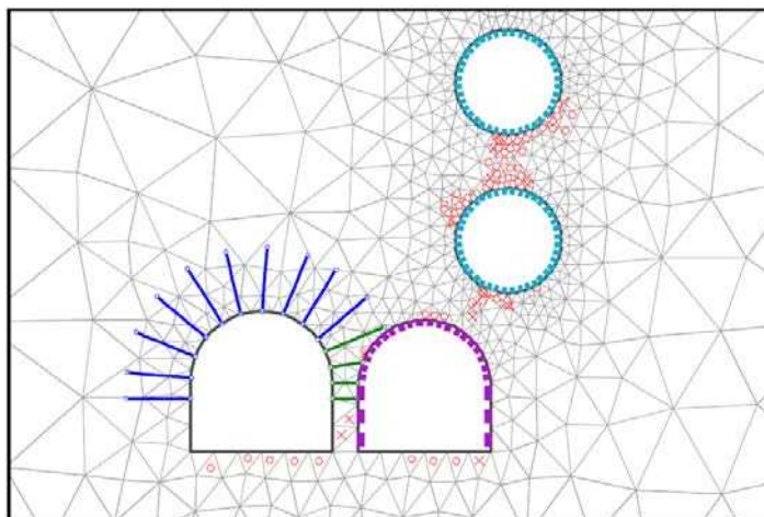
شکل ۸-۱- طراحی سیستم نگهداری با استفاده از روش اجزا محدود (x: تسلیم در کشش و ×: تسلیم در فشار) [۱۸۶]
