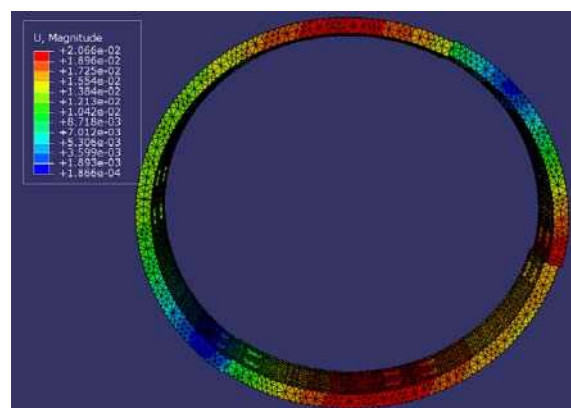
شکل ۲۸-۱۰- بزرگی جابجایی‌ها با فاکتور بزرگنمایی (x10)
