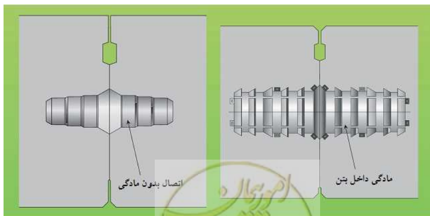
شکل ۱۲-۳۲- اتصالات داوولی [۲۳۰]
