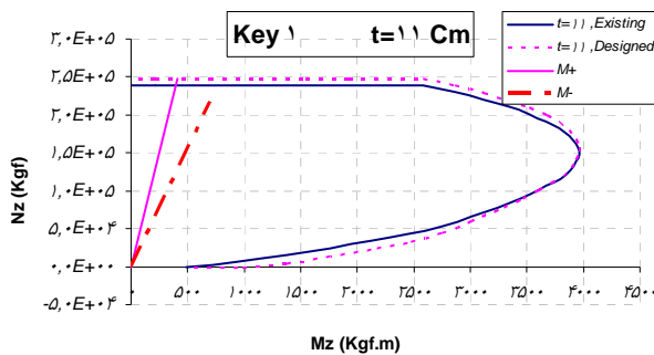
شکل ۱۰-۵۰- نمودار اندرکنش نیروی محوری - ممان در مقطع لانه زنبوری پوشش داخلی سگمندی
