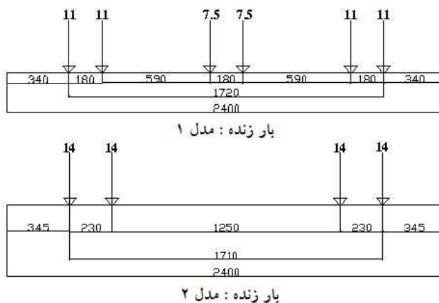
شکل ۱۰-۸ - بار زنده ناشی از تردد قطار در تونل [۲۰۵]
