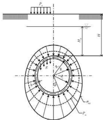
شکل ۱۰-۱۴ بار وارد بر روی سیستم نگهداری [۲۲۰]
