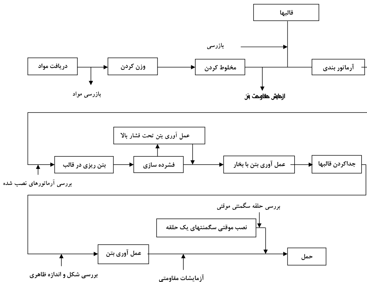
شکل ۱۱-۱۲- فلوجارت مراحل تولید سگمنت [۲۳۱]
