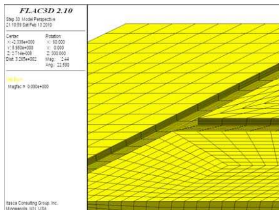
شکل ۸-۹- هندسه مدل عددی ساخته شده تقاطع تونل ۴ غربی معدن زغالسنگ پروده ۵ طیس با استفاده از نرم افزار FLAC^3D (برش از وسط)
