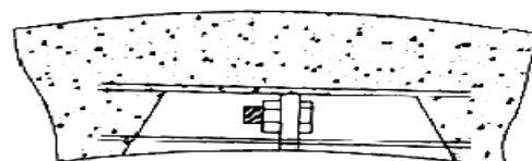
سیستم اتصال با استفاده از صفحه فولادی و بولتهای کوتاه [۵]
