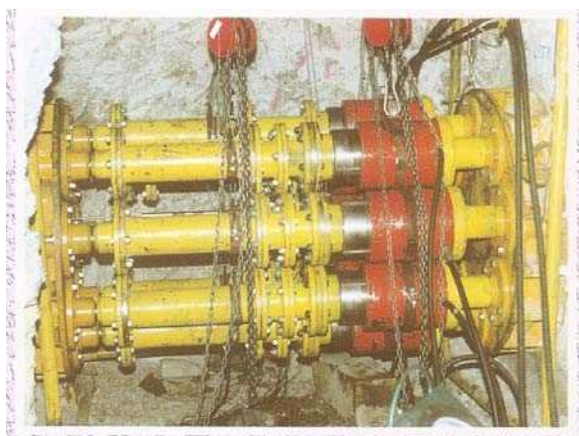
شکل ۴-۳۱- نحوه انجام آزمایش بارگذاری صفحه‌ای در سنگ
