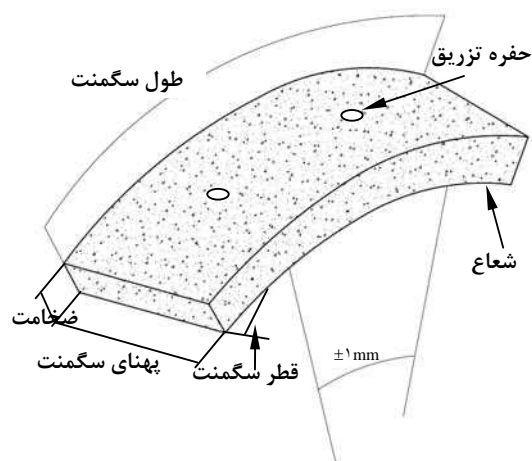
شکل ۱۲-۱- هندسه و حداکثر خطای مجاز سگمنت [۲۳۰]
