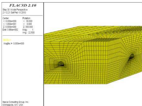
الف- هندسه مدل عددی ساخته شده تقاطع تونل ۴ غربی معدن زغالسنگ پروده ۵ طیس با استفاده از نرم افزار FLAC 3D شکل ۸-۸- هندسه مدل
