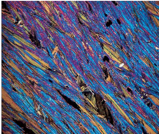
ب- نمایی از شیستوزیته در زیر میکروسکوپ
