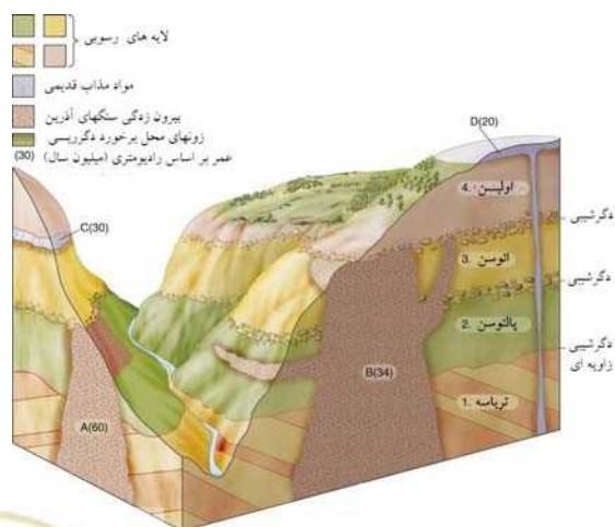
شکل ۳-۱۱- تشخیص لایه‌های مختلف زمین با استفاده از چینه شناسی [۲۸]
