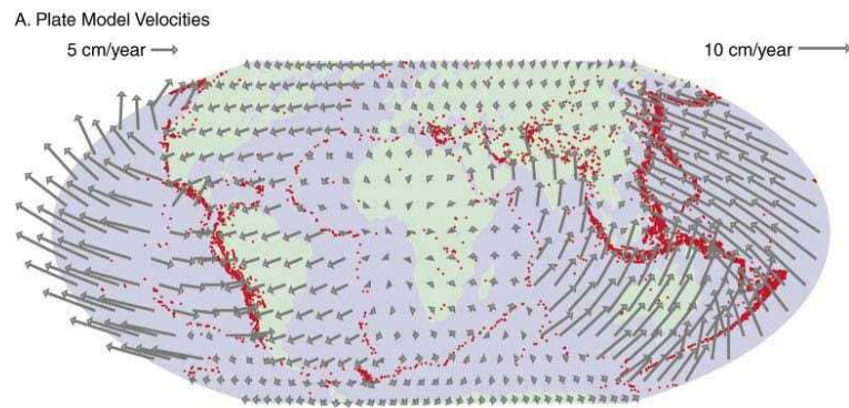
شکل ۳-۴۰- حرکت نسبی صفحات پوسته زمین [۲۸]
