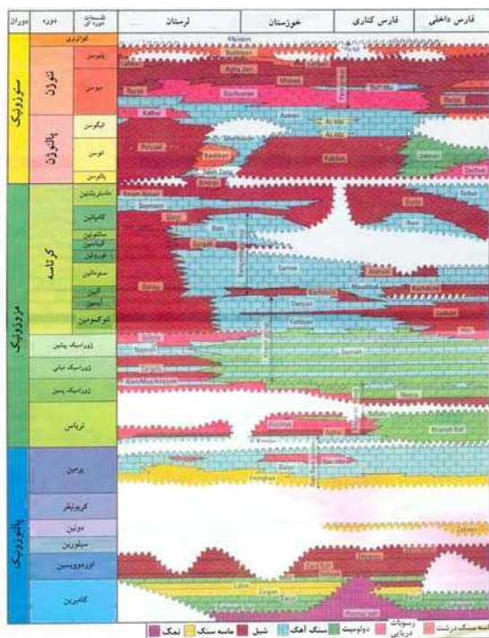
شکل ۳-۱۱- تشخیص لایه‌های مختلف زمین با استفاده از چینه شناسی [۲۸]
