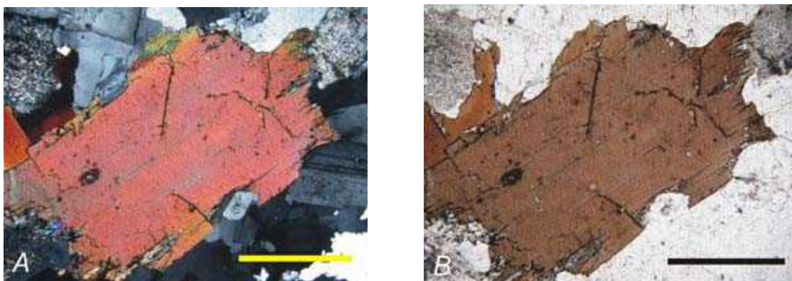
بیوتیت زیر نور پلاریزان
