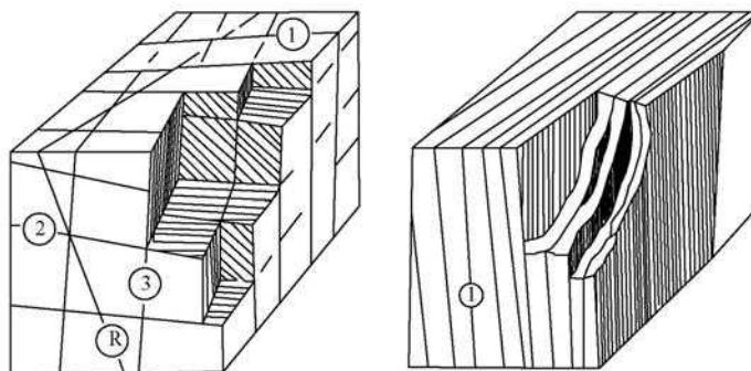
شکل ۴-۲۰- رابطه تعداد دسته درزه‌ها با رفتار مکانیکی و شکل ظاهری توده سنگ [۶۳]
