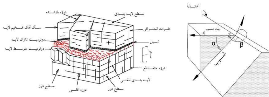
شکل ۴-۱۲- نمایش سه بعدی امتداد شیب و جهت شیب [۶۳]: \alpha : شیب، \beta : جهت شیب
