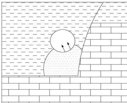
در امتداد سطح گسل اصطکاک کم و چسبندگی سنگ‌ها ضعیف است. به علت عبور آب‌های زیرزمینی از شکاف گسل، احتمال هوازدگی عمیق بنا بر این احتمال ریزش در این قسمت‌ها وجود دارد.
