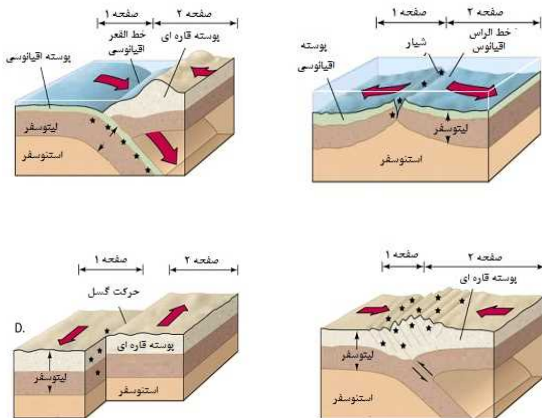
شکل ۳-۳۸- نحوه وقوع زمین لرزه [۱۳]
