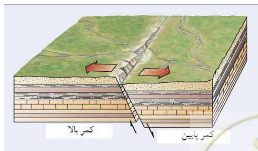
شکل ۳-۲۲- انواع گسل [۲۸]
