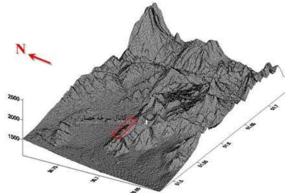
شکل ۴-۸- توپوگرافی سه بعدی تهیه شده از تصاویر ماهواره‌ای (Dem)
