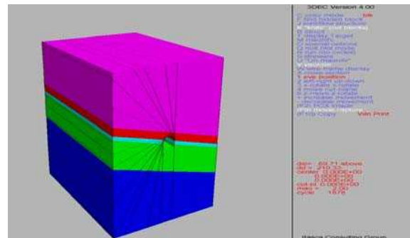
شکل ۸-۱۳- هندسه مدل عددی ساخته شده تونل ۴ غربی معدن زغالسنگ پروژه ۵ طیس با استفاده از نرم افزار 3DEC
