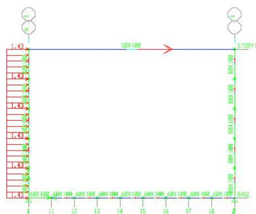
شکل ۱۰-۷۴- نیروی زلزله
