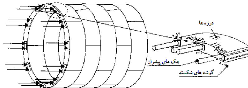
شکل ۱۲-۳۶- شکستگی ها در اثر نیروی جک ها [۲۴۰]
