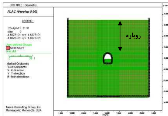
شکل ۸-۱- هندسه مدل عددی ساخته شده تونل اصفهان - شیراز با استفاده از نرم افزار FLAC
