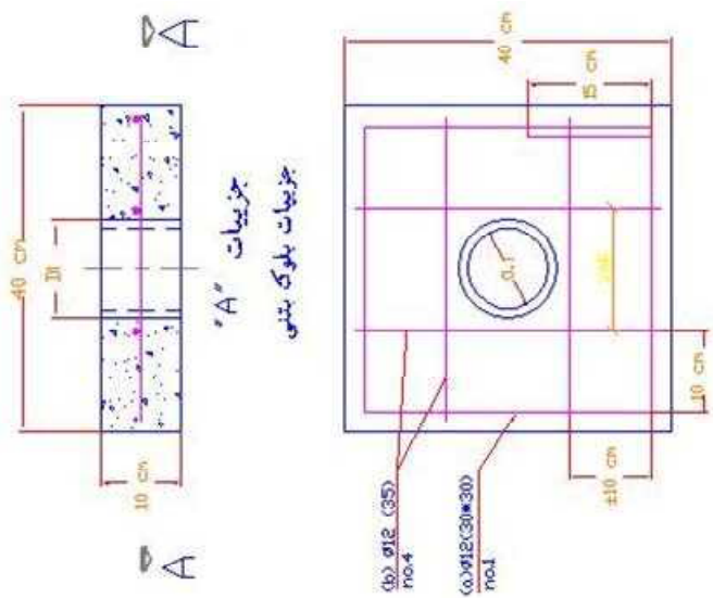
مقطع A-A
