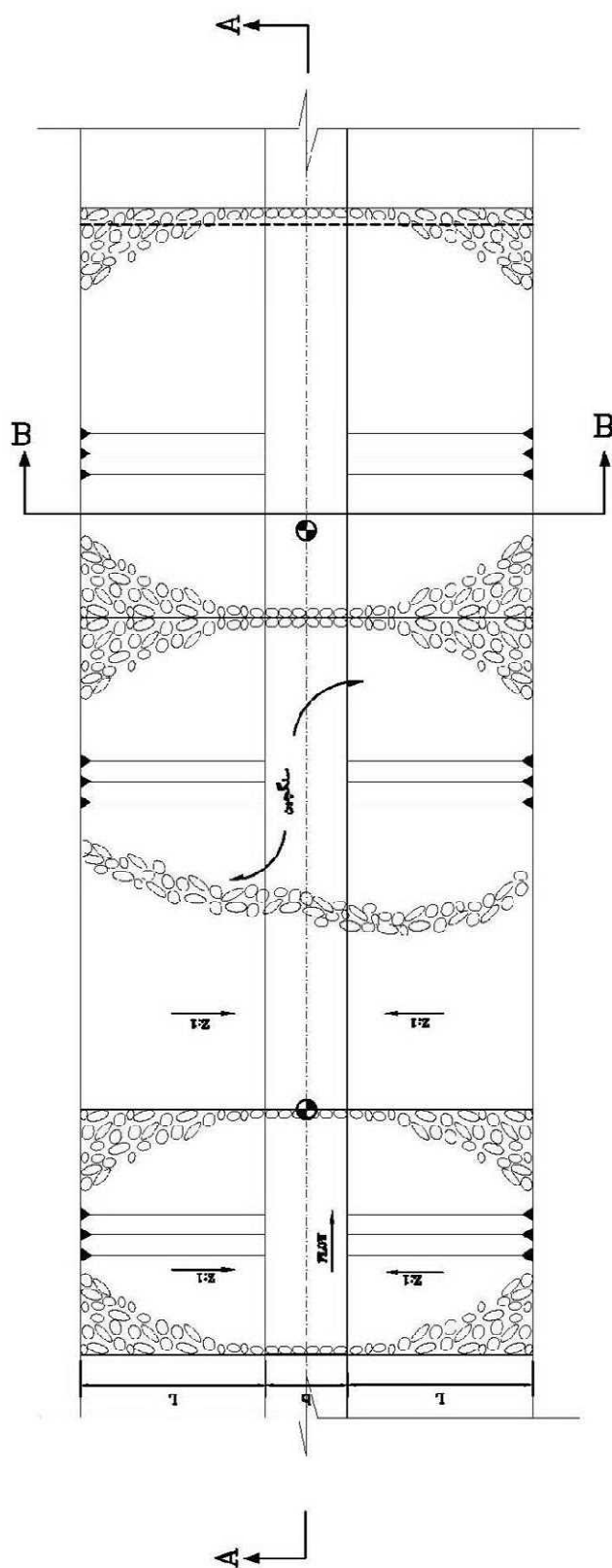
پلان آبخار در مسیر زهکش جمع کننده مزرعه
