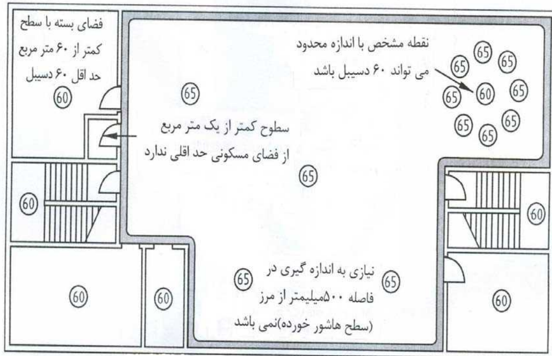
اعداد مندرج در شکل بیانگر سطوح حداقل بر حسب دسیبل می باشد
