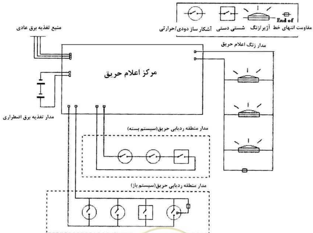
شکل ۱-۲-۱-۲-۳: نمونه سیستم اعلام حریق متعارف
