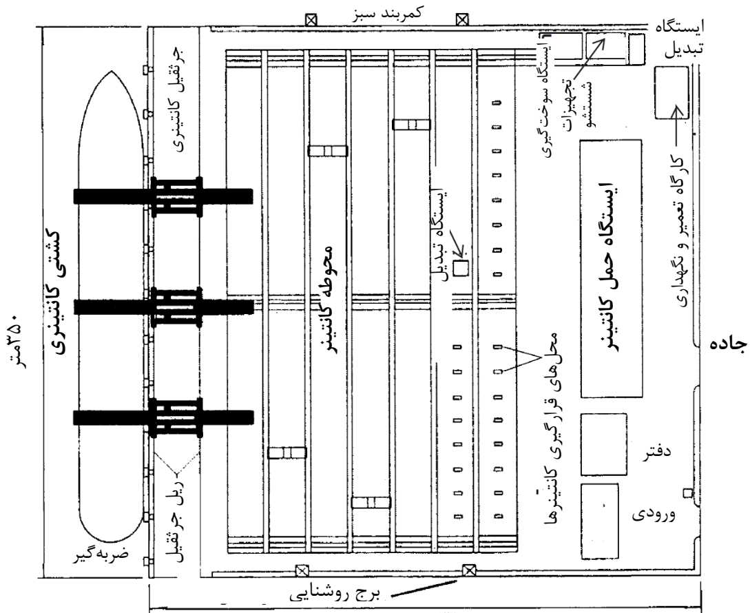
شکل ۱۰-۱- نمونه‌ای از جانمایی پلان تجهیزات یک پایانه کانتینری در اسکله‌های سپری ۳۵۰ متر
