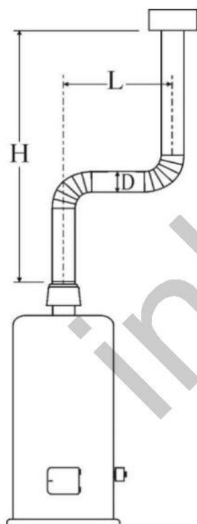
شکل ۱۷-۷-۱ دستگاه گازسوز برای استفاده یک دستگاه گازسوز
