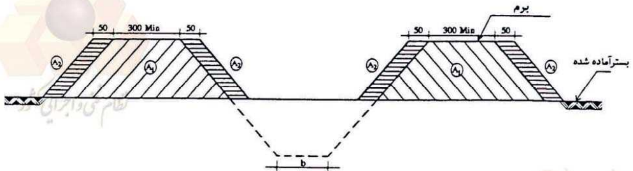
شکل ۶-۴. شمای مقطع خاکریزی
