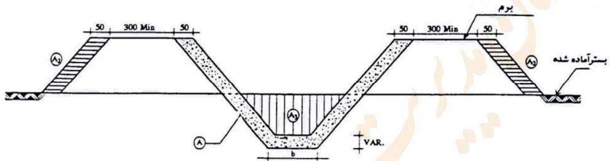
شکل ۶-۵. شمای مقطع خاکبرداری
