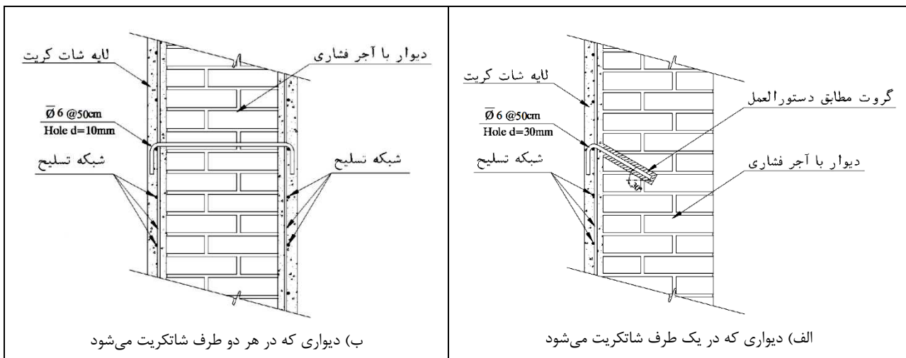
شکل ۷-۱- نحوه اتصال آرمانتور دوخت به دیوار
