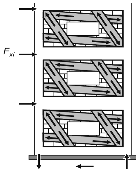
شکل ۶-۲- اعضای فشاری معادل میانقاب دارای بازشو
