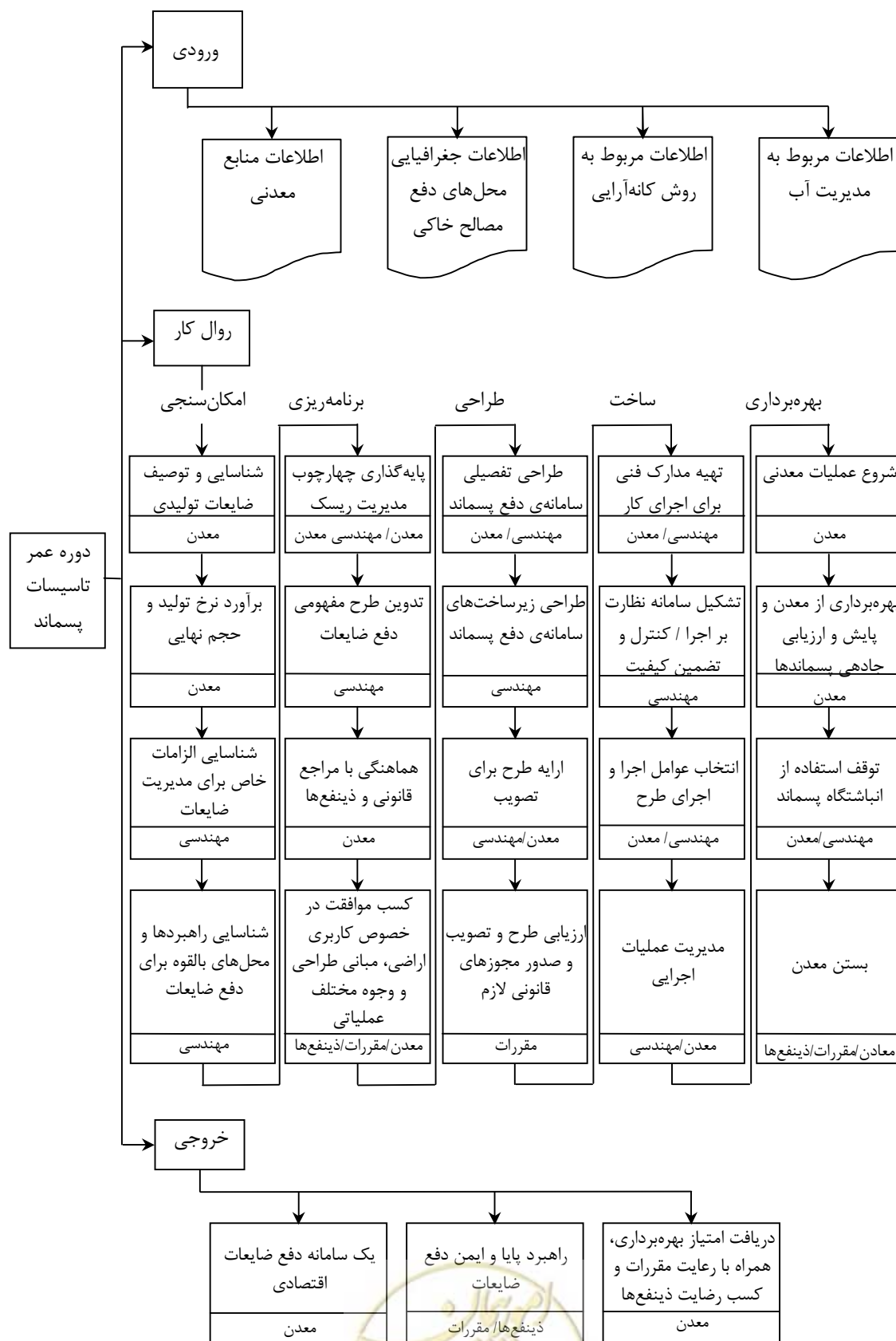
شکل ۱-۱-۱- روال برنامه ریزی، طراحی، ساخت، بهره برداری و بستن (رهاسازی) سدهای پسماند
