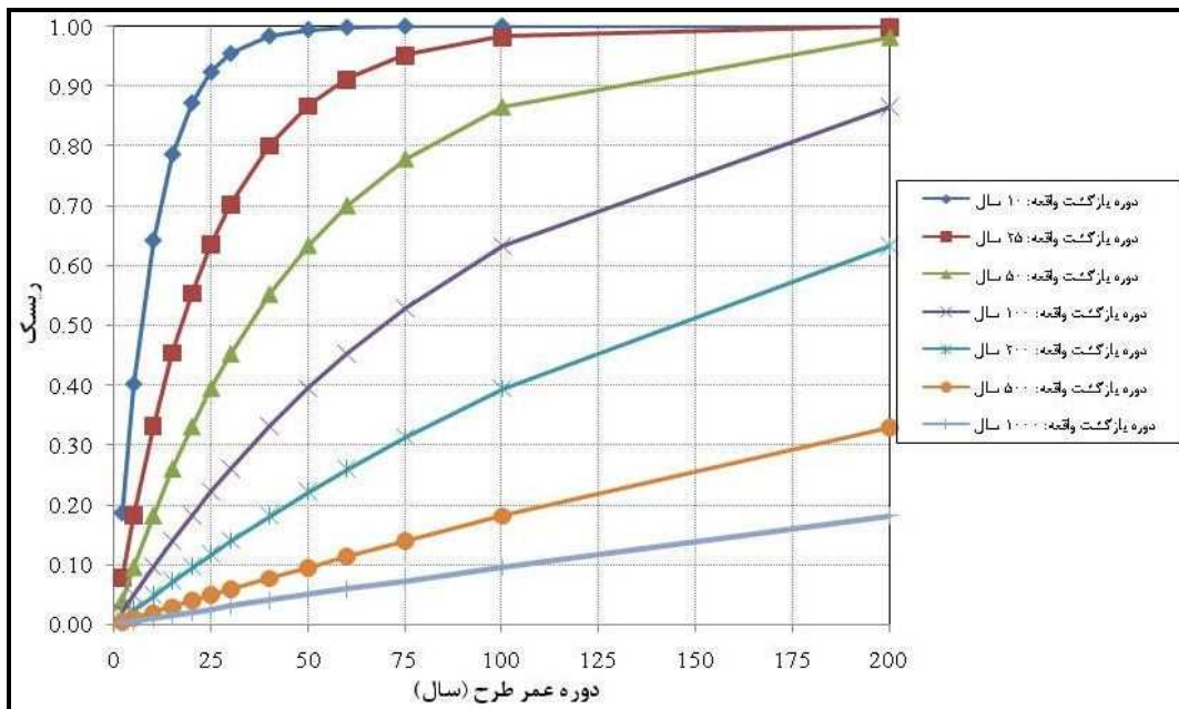
شکل پ.۱-۲- منحنی ریسک سیلاب برای دوره‌ی عمر مختلف طرح و دوره‌ی بازگشت مشخص- رخداد دوبار درسال
