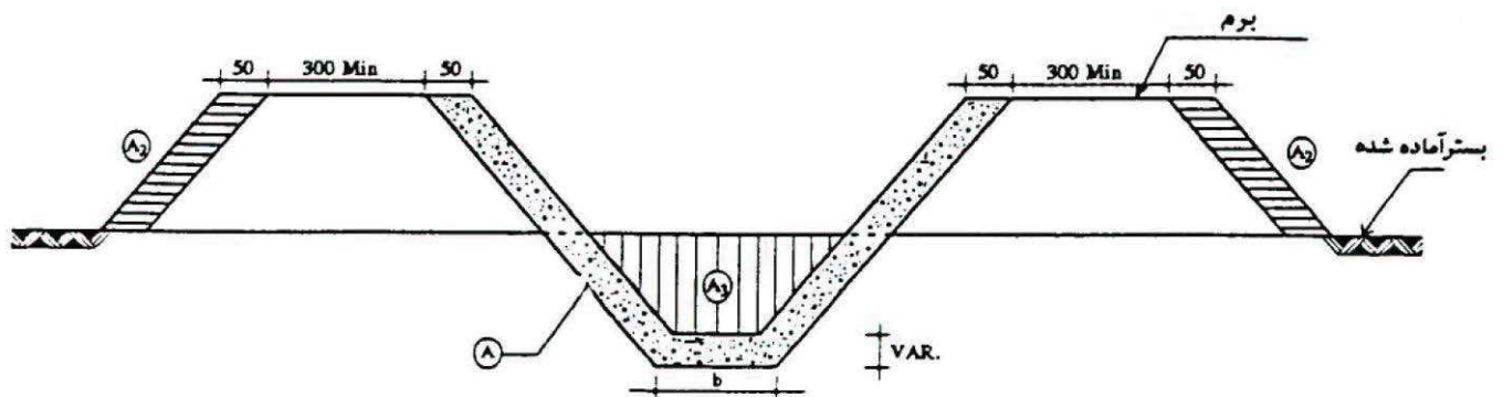
شکل ۶-۵. شمای مقطع خاکبرداری
