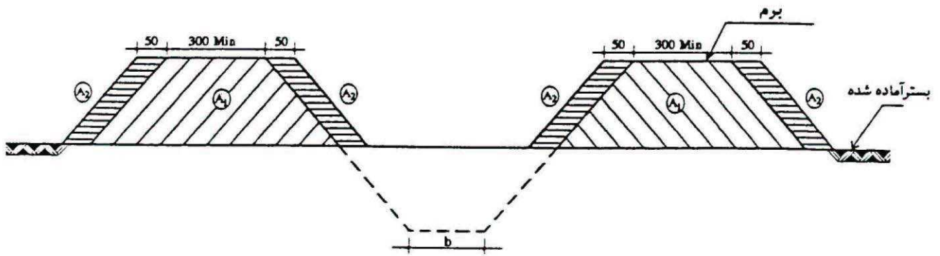
شکل ۶-۴. شمای مقطع خاکریزی
