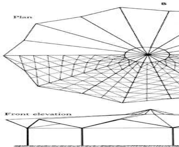
شکل ۴-۲- سازه فضایی با ستون‌های مستقل
