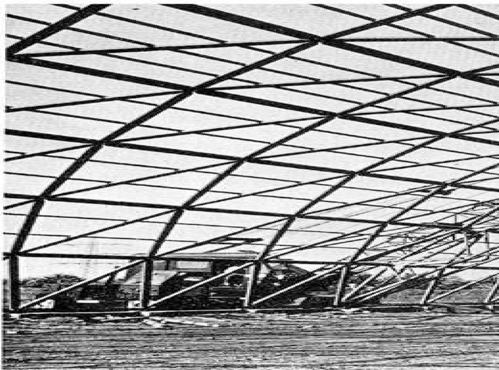
شکل ۴-۴- نمونه‌های ساخته شده سیستم‌های پوسته‌ای
