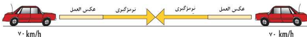
شکل ۳-۱۴- امکان تأمین دید وسایل نقلیه دو طرف نسبت به یکدیگر در محل باریک شدن
