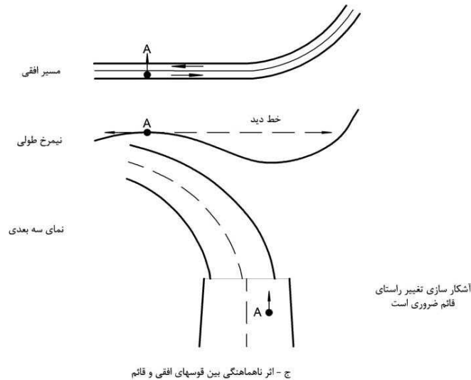
ادامه شکل ۳-۱۱- حالت‌های مختلف ترکیب راستای افقی و قائم
