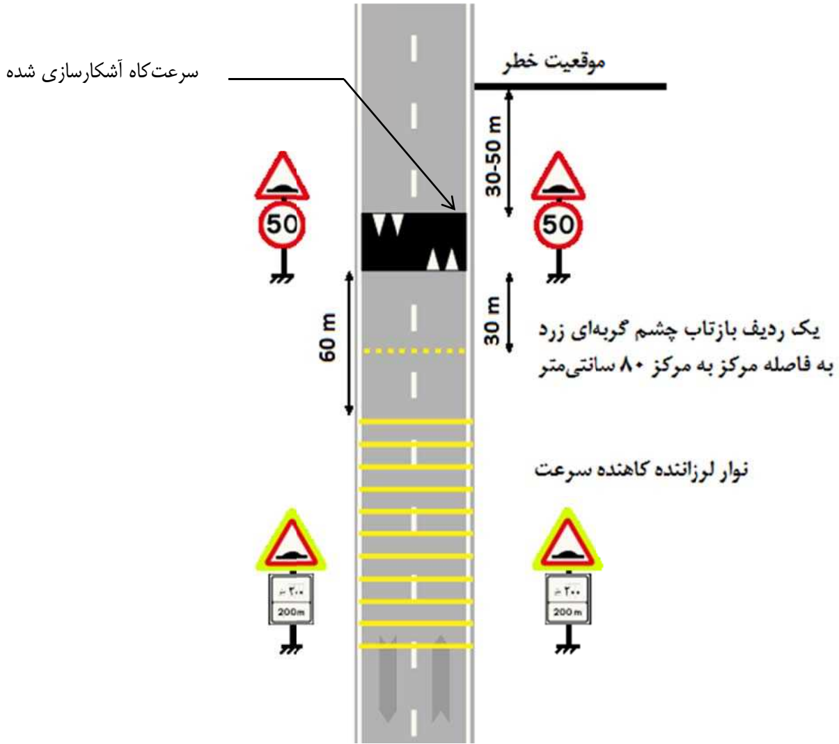
شکل ۳-۴۸-الف-نمونه‌ای از طرح سرعت‌کاه در راه‌ها، ده‌خطه
