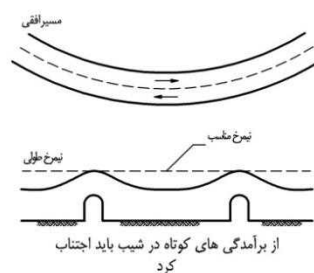
ب - نیمرخ با مسیر منحنی
