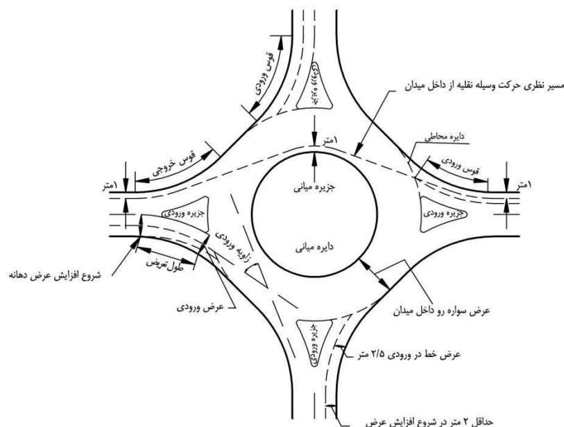
شکل ۳-۲۹- اجزای میدان
