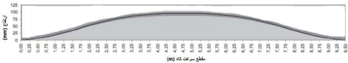
شکل ۳-۴۸-ب-مقطع عرضی سرعت‌کاه سینوسی با سرعت ۵۰ کیلومتر در ساعت
