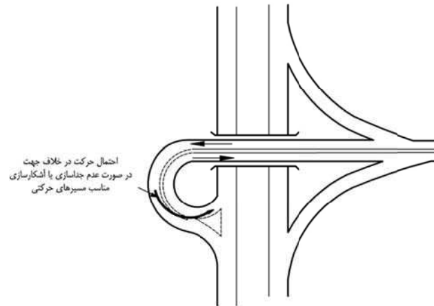
شکل ۳-۳۷- احتمال حرکت اشتباه در صورت عدم جداسازی مسیرهای حرکت در داخل گردراهه
