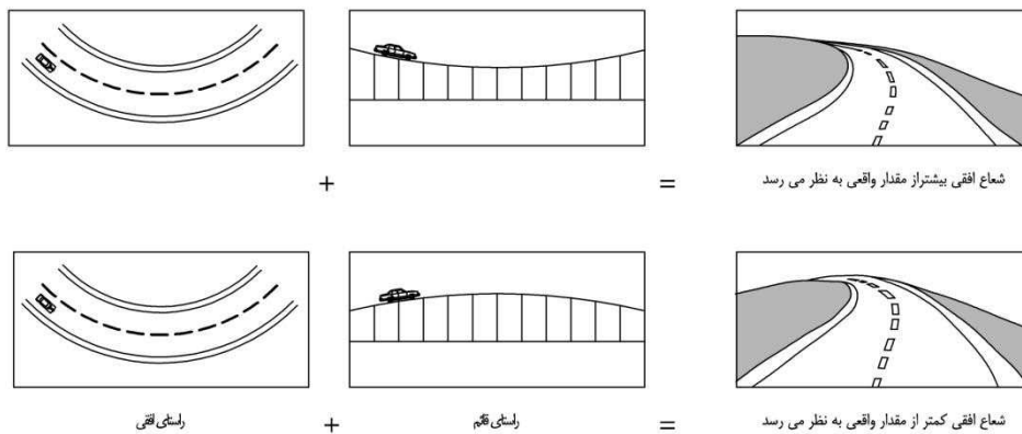
شکل ۳-۱۲- ترکیب قوس افقی و قائم و ایجاد خطا در تشخیص انحنای قوس افقی
