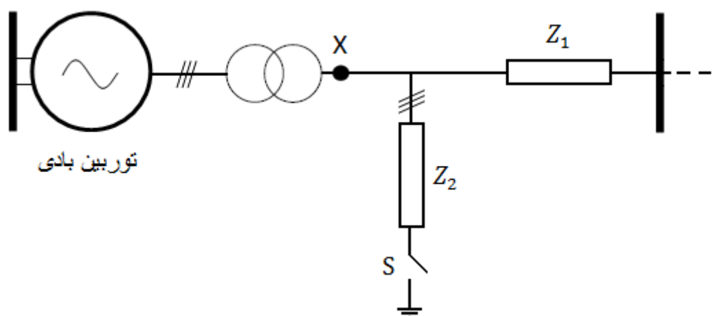
شکل (۲-۴): مدار تست LVRT
