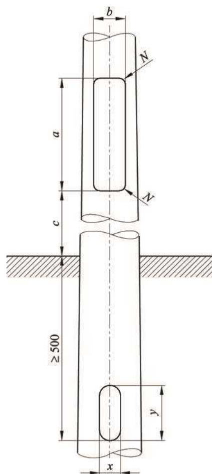
شکل (۱۴-۴): نمای مقابل برای آزمون ضربه درب دریچه
