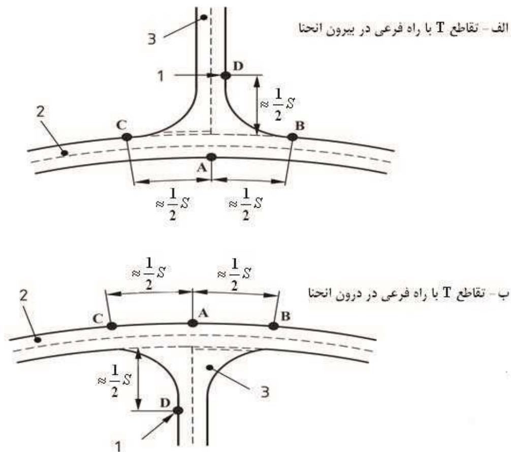
شکل (۸-۲): تقاطع‌های T در درون و بیرون انحنای
