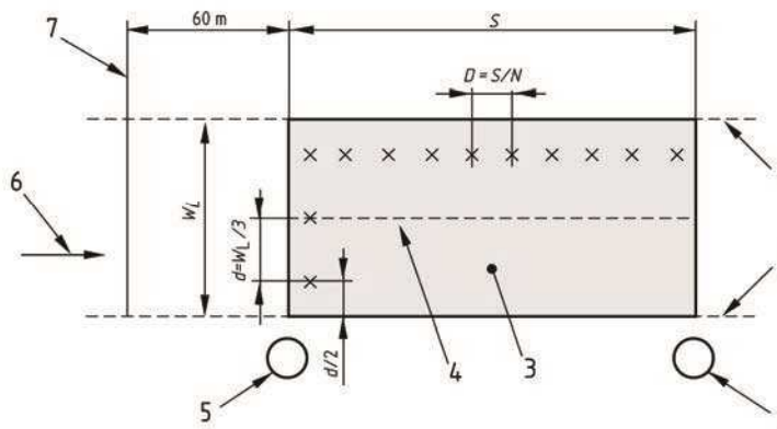
شکل (۵-۵): موقیعت نقاط محاسباتی در هر باند ترافیکی
