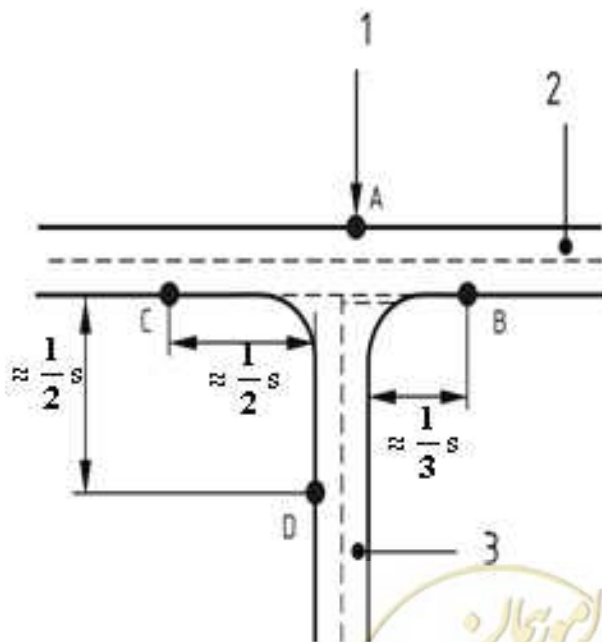
شکل (۸-۱): سیستم روشنائی تقاطع T در معابر مستقیم
