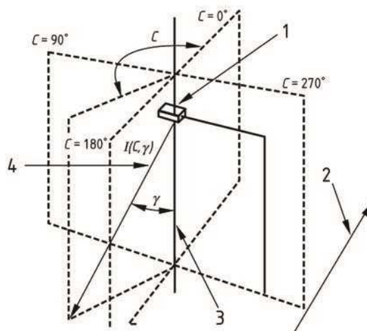
شکل (۲-۵): موقعیت سیستم مختصات C و \gamma نسبت به جهت طولی معبر
