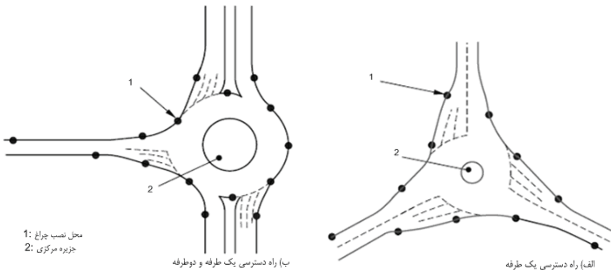
شکل (۸-۱۰): میدان در تقاطع‌های سه راهه
