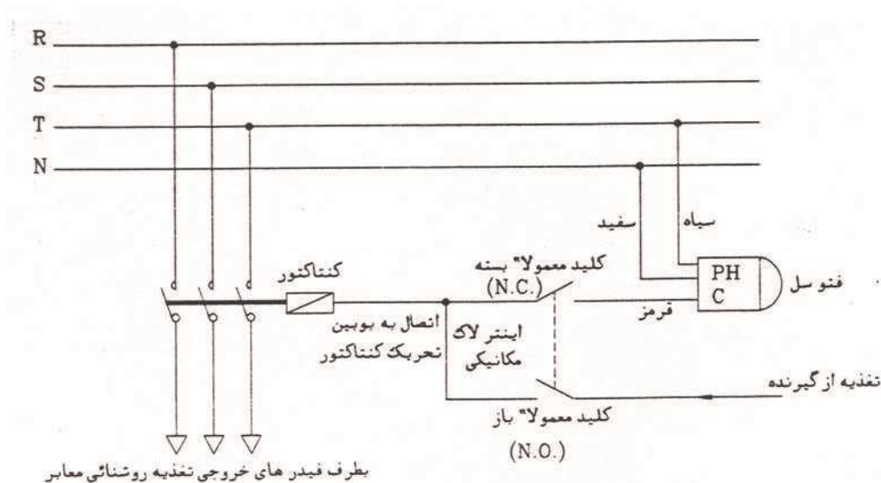
شکل (۱۶-۸): دیاگرام مدار فرمان روشنایی معابر با استفاده از سیستم کنترل از راه دور
