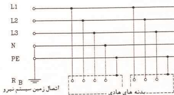
شکل (۱۶-۴): سیستم زمین نوع TN-S
