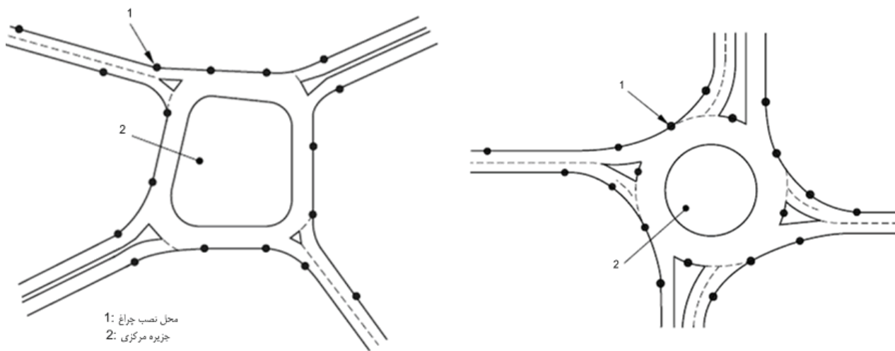
شکل (۸-۱۱): میدان در تقاطع‌های چهار راهه
