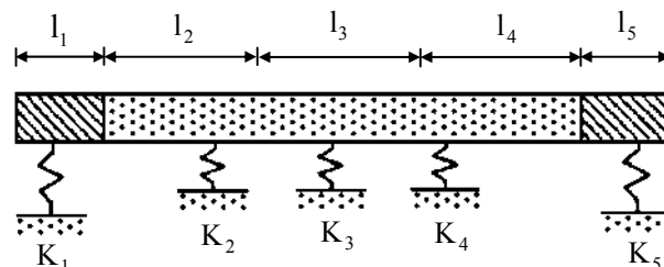
شکل (۴-۴): سختی فنرهای قائم برای پی‌های سطحی غیر صلب
