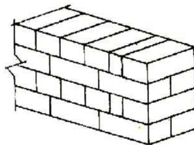
شکل (۱۱-۲): وضعیت رج‌های طرفین دیوار
