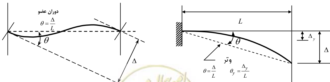
ب- مثال عضوی از یک قاب
