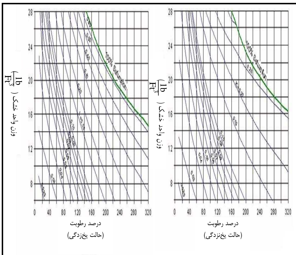
شکل پ. ۱-۶- متوسط ظرفیت انتقال حرارتی برای خاک‌های نباتی در دو حالت یخ‌زدگی و یخ‌نزدگی (برگرفته از Kersten, 1949 and Air Force, 1966 [۲۷ و ۲۵ و ۳۱])
