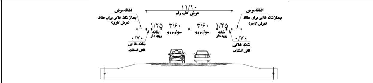
A3- راه شریانی دو خطه با ADT کمتر و برابر ۲۰۰۰
