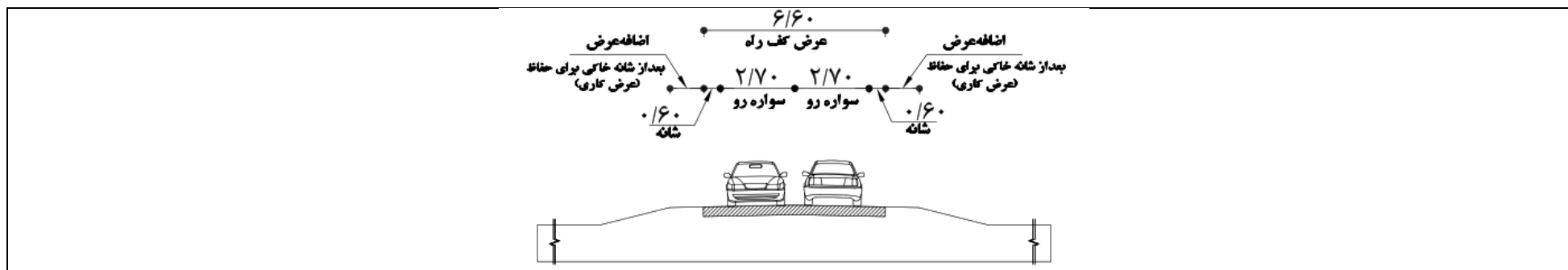
C1- راه جمع کننده دو خطه با ADT کمتر از ۲۵۰
