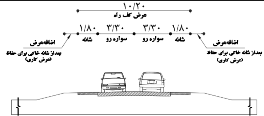
L4- راه محلی دو خطه با ADT بیشتر از ۲۰۰۰
