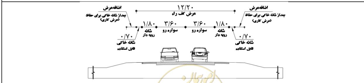
A4- راه شریانی دو خطه با ADT بیشتر از ۲۰۰۰
