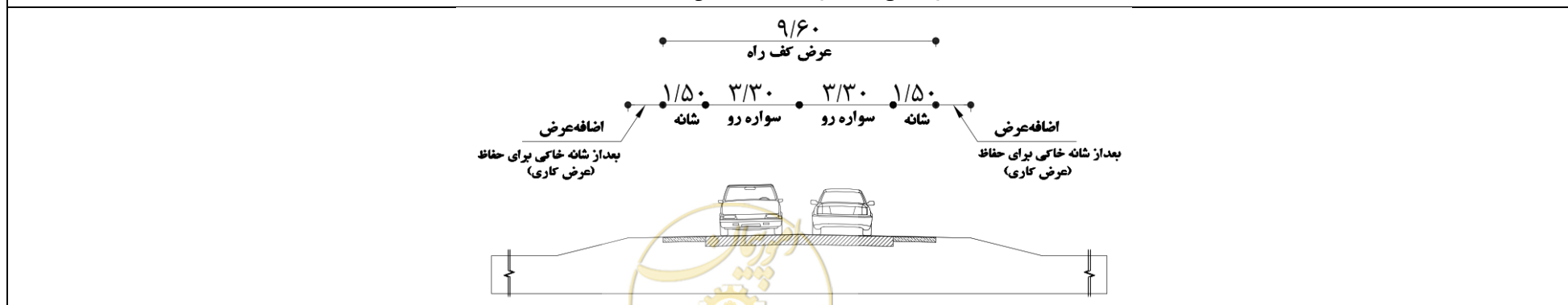
C3- راه جمع کننده دو خطه با ADT بین ۴۰۰ تا ۲۰۰۰
