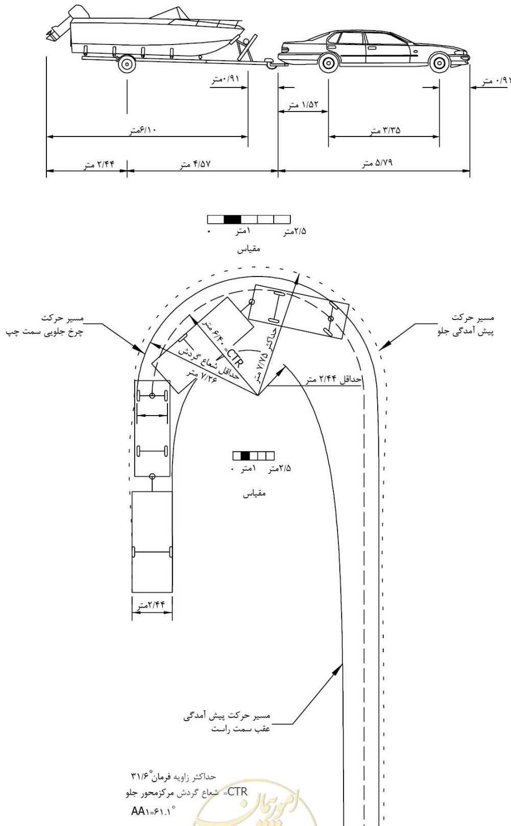
شکل ۴-۱۰- حد اقل مسیر گردش برای وسیله طرح سواری با یدک قایق
