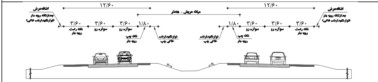
F10- آزادراه چهار خطه با DDHV برابر و بیشتر از ۲۵۰ با میانه عریض
