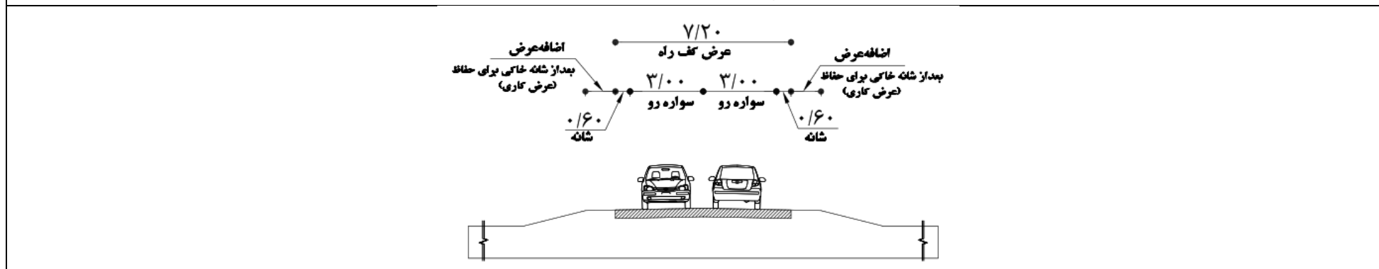
C2- راه جمع کننده دو خطه با ADT بین ۲۵۰ تا ۴۰۰
