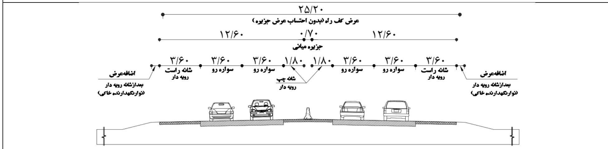
F2- آزادراه چهار خطه با DDHV برابر و بیشتر از ۲۵۰
