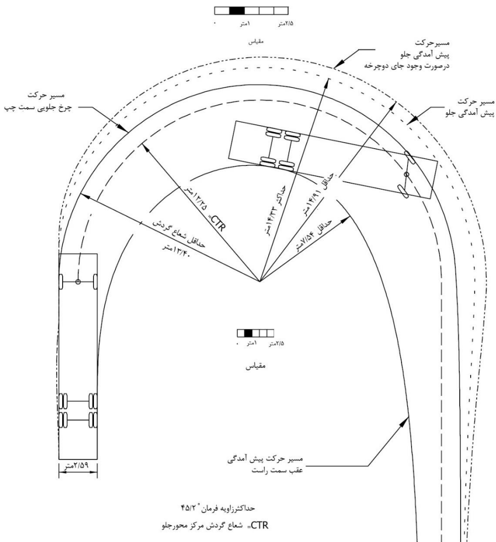
شکل ۴-۶- حداقل مسیر گردش برای وسیله طرح اتوبوس نوع ۲
