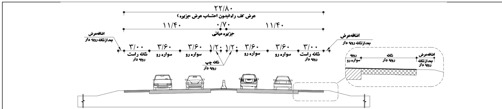
F1- آزادراه چهار خطه با DDHV کمتر از ۲۵۰
