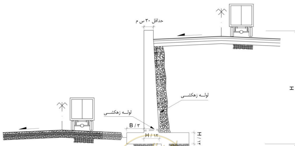
شکل ۶-۲۱- دیوار حائل وزنی
