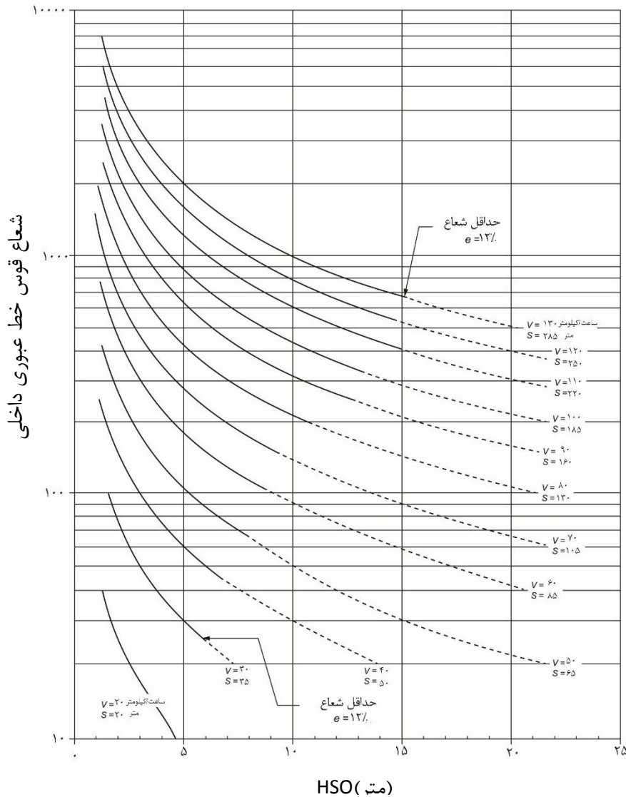
شکل ۵-۸- تعیین HSO در قوس افقی برای فاصله دید توقف فاصله خط دید افقی (مرکز خط داخل تا مانع) (متر) HSO (متر)
