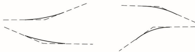
گردش‌دگی گوشه‌های سواره رو در محل اعمال بریلندی
