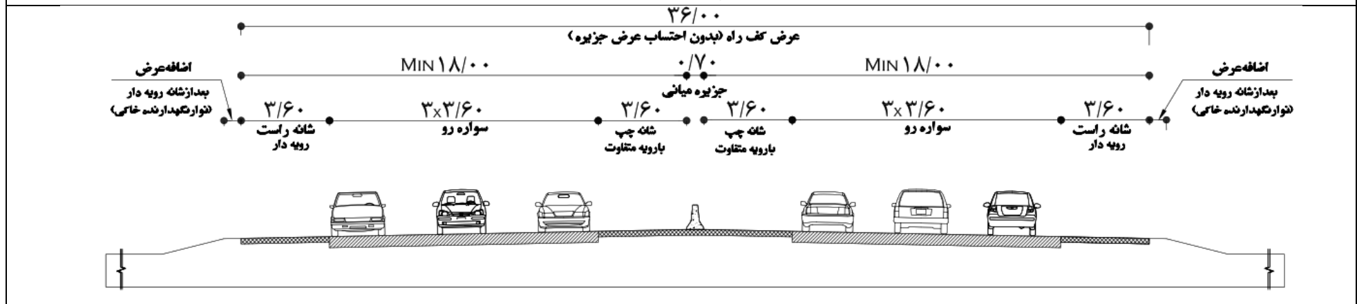
F4- آزادراه شش خطه با DDHV برابر و بیشتر از ۲۵۰
