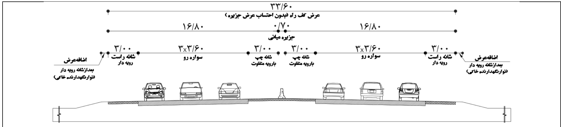
F3- آزادراه شش خطه با DDHV کمتر از ۲۵۰
