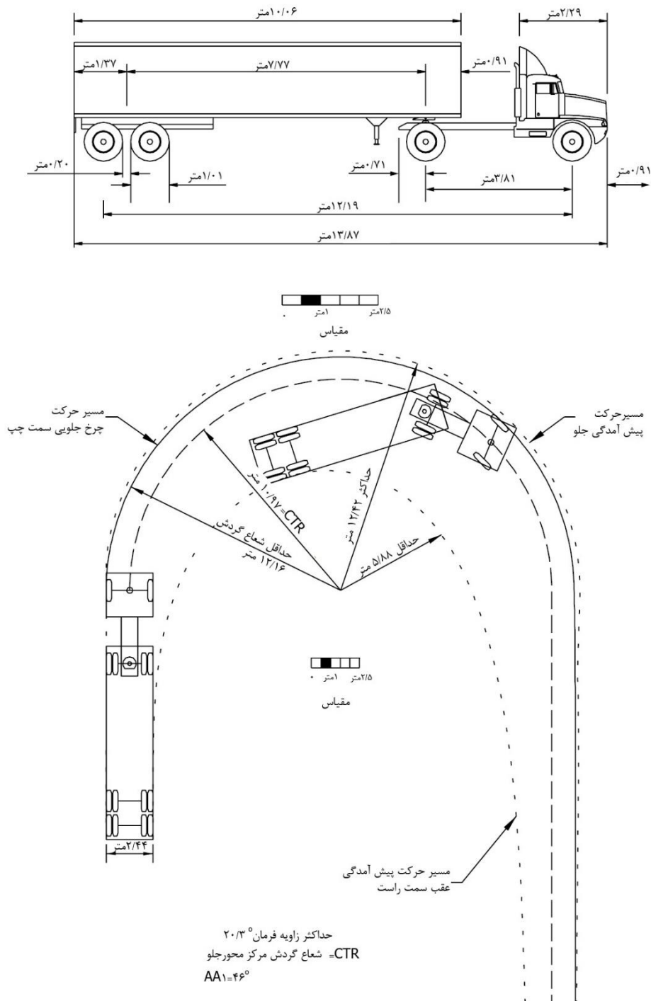
شکل ۴-۷- حدافل مسیر گردشی برای وسیله طرح تریلی نوع ۱
