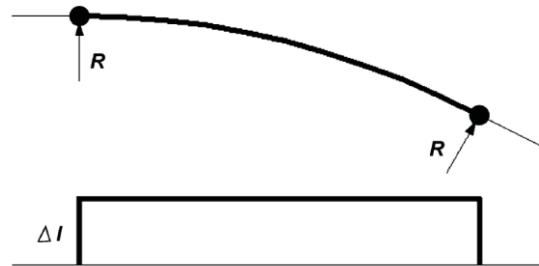
شکل ۵-۷ ترکیب قوس دایره و مسیر مستقیم بدون بریلندی (نمونه یک انشعاب استاندارد)
