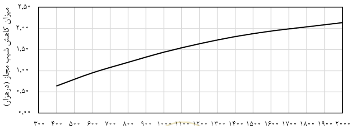
شکل ۲-۷ کاهش شیب مجاز بر حسب طول تونل
