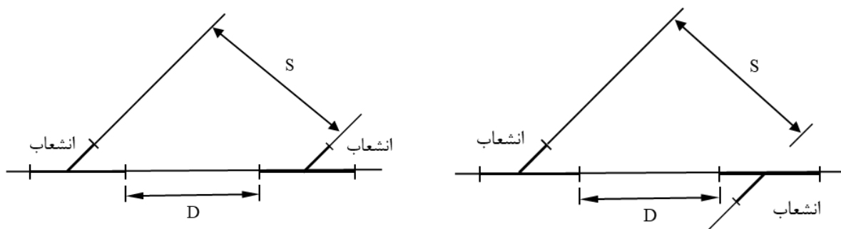
شکل ۵-۱۳ حالات استقرار انشعاب‌های موازی در یک خط
