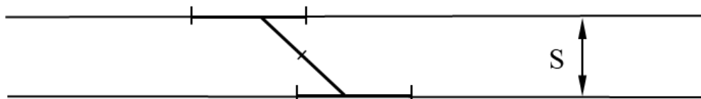
شکل ۹-۵ فاصله بین دو خط موازی با اتصال انشعاب
