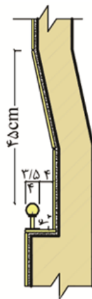
شکل ۲-۹۸: جزئیات تورفتگی میله دستگرد در دیوار
