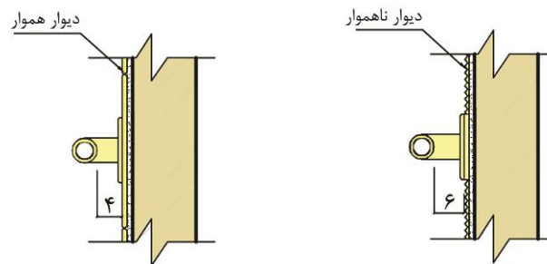
شکل ۲-۹۷: فاصله میله دستگرد در کنار دیوار هموار و ناهموار
