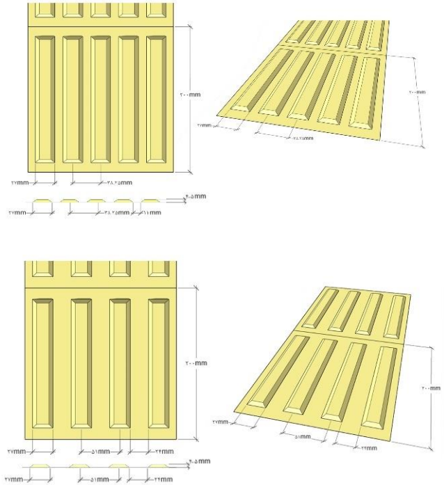
شکل ۲-۲۰: نشانگرهای لمسی هدایت‌کننده ۲۰ \times ۲۰ سانتیمتر با شیارهایی به عرض ۲۷ میلی‌متر (۴ و ۵ شیار)
