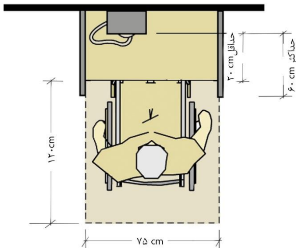
شکل ۲-۱۴۴: فضای آزاد دسترسی از روبرو به تلفن عمومی
