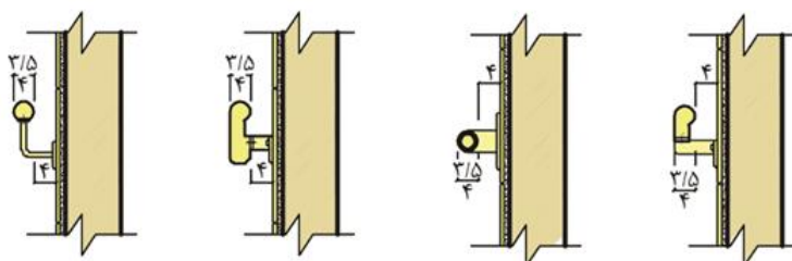
شکل ۲-۹۴: ابعاد مقطع عمودی میلۀ دستگرد
