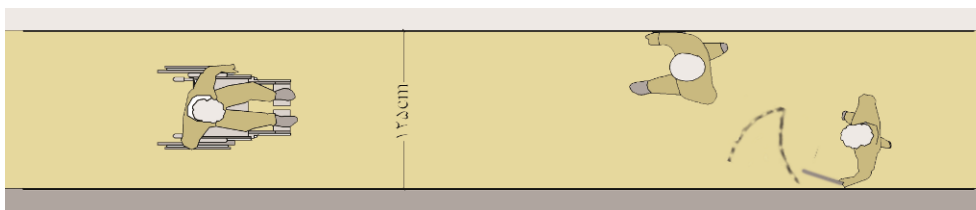
شکل ۲-۱: حداقل عرض مفید پیاده‌رو
