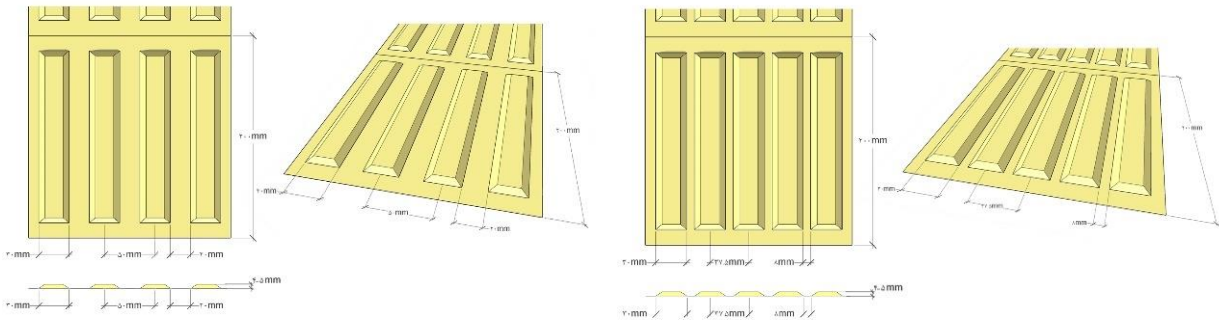
شکل ۲-۲۱: نشانگرهای لمسی هدایت‌کننده ۲۰ \times ۲۰ سانتیمتر با شیارهایی به عرض ۳۰ میلی‌متر (۴ و ۵ شیار)
