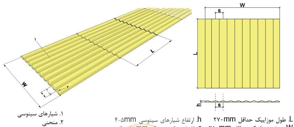
شکل ۲-۱۹: چیدمان، فواصل و ابعاد کفیوش شیاردار سینوسی
