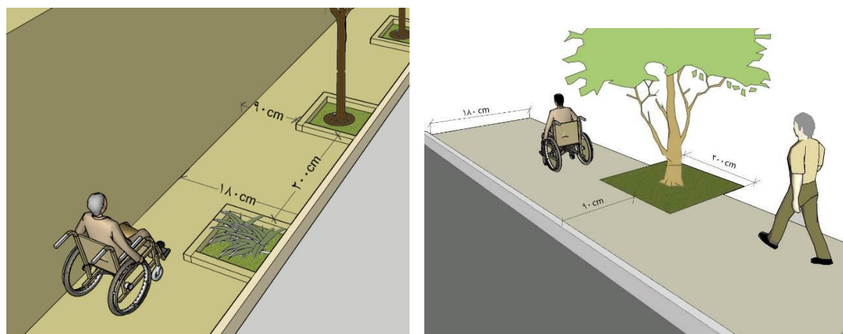
شکل ۲-۶: ملاحظات در محل کاهش عرض مسیر پیاده دسترس‌پذیر
