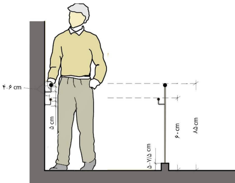
شکل ۲-۹۵: جزئیات میلۀ دستگرد
