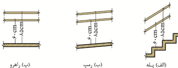
شکل ۲-۸۹: ارتفاع میله دستگرد از کف
