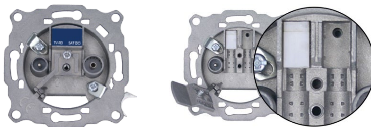
شکل ۲-۲۰- یک نمونه پریز انتهایی و نمای داخلی آن
