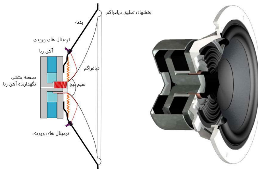
شکل ۷-۱۰۹- ساختمان داخلی یک بلندگو با واحد راه‌انداز دینامیک
