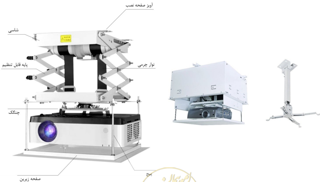
شکل ۸-۳۷- دو نمونه پایه ویدیو پروژکتور متحرک برقی چند نمونه پایه پرده ویدیو پروژکتور ثابت و برقی
