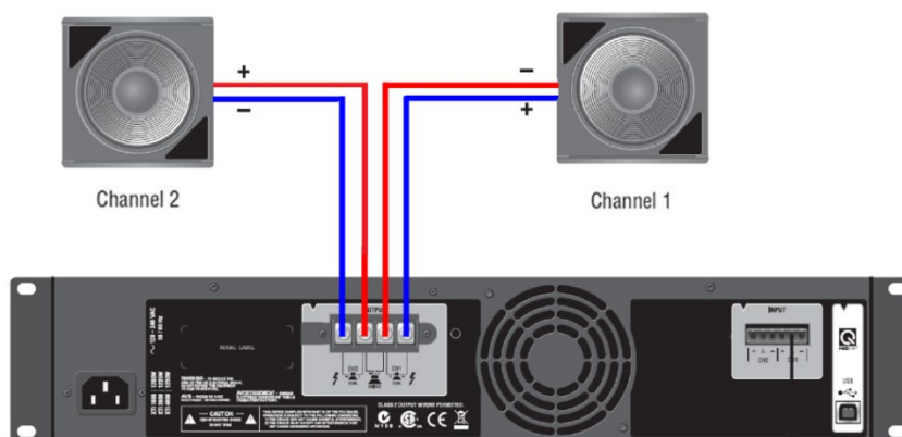
شکل ۷-۸۴- طریقه اتصال تقویت‌کننده به بلندگو در حالت دوتایی و Y
