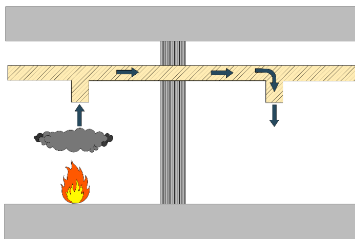
شکل ۴-۶۳- تصرفی بدون استفاده از دتکتور کانالی - شروع حریق از واحد سمت چپ
