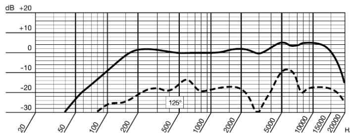
شکل ۷-۲۱- یک نمونه پاسخ فرکانسی میکروفن در محور اصلی و زاویه ۱۲۵ درجه
