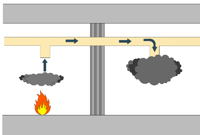
شکل ۴-۶۴- تصرفی بدون استفاده از دتکتور کانالی - حریق توسط کانال سیستم تهویه به واحد (های) دیگر سرایت می کند.
