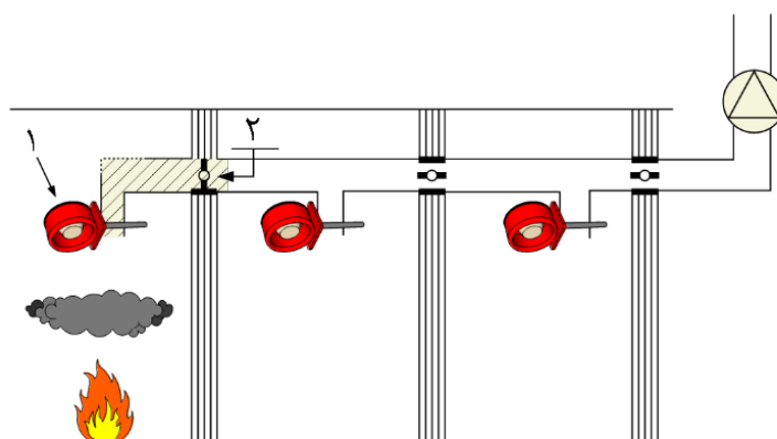
شکل ۴-۶۴- تصرفی بدون استفاده از دتکتور کانالی - حریق توسط کانال سیستم تهویه به واحد (های) دیگر سرایت می کند.
