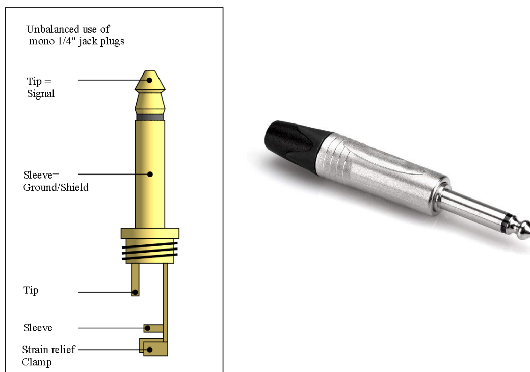
شکل ۷-۱۴۷- یک نمونه فیش TS و نام‌گذاری و اتصال پایه‌های آن
