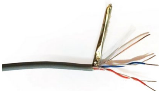
شکل ۶-۲- یک نمونه کابل ارتباطی سیستم‌های آوایر صوتی
