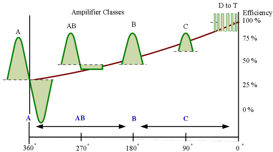
شکل ۷-۸۹- منحنی مقایسه چند کلاس مختلف از تقویت‌کننده‌ها
