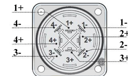
WIRING
