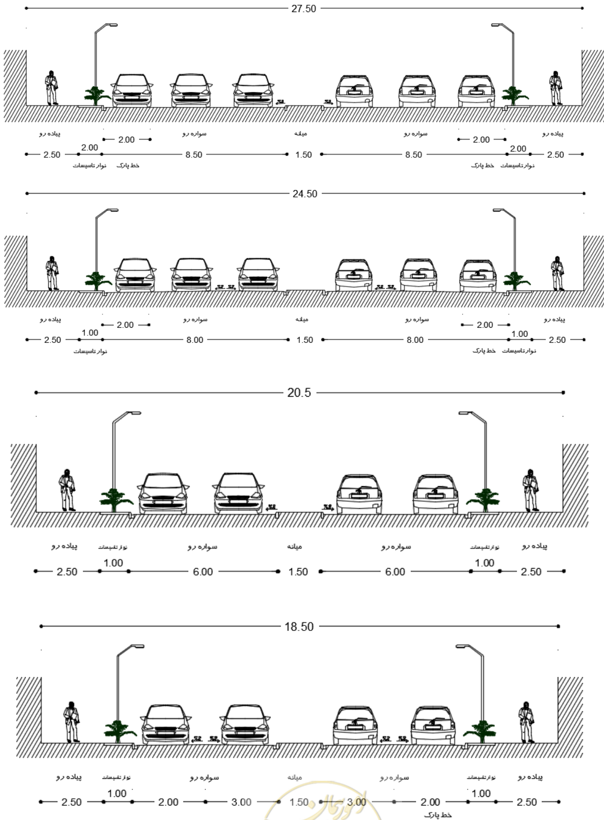
شکل پ ۱-۲- مقطع عرضی معبر تیب یک - عرض ۱۸.۵ و ۲۰.۵ و ۲۴.۵، ۲۷.۵ - جداول نوع A و B
