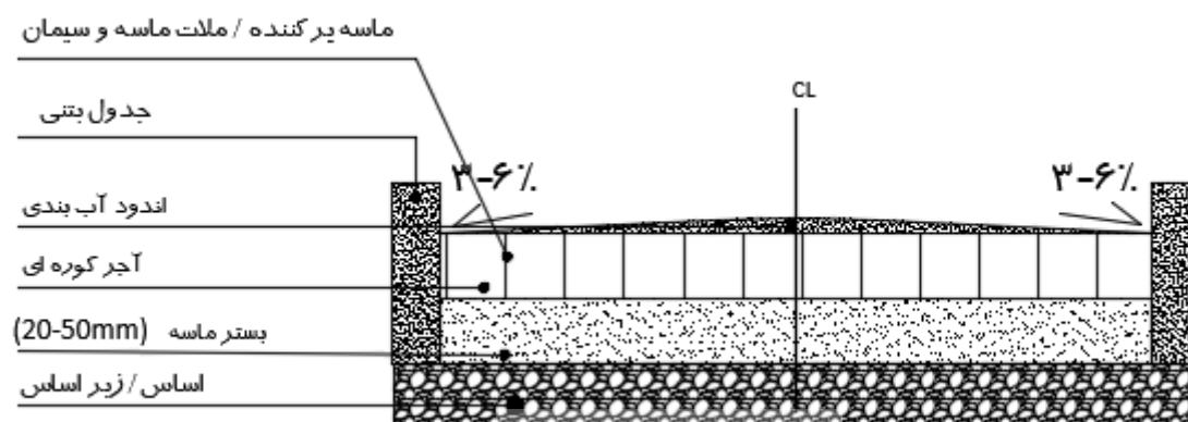
شکل ۶-۳۰- مطع عرضی روسازی معبر با رویه آجر فرش کوره ای
