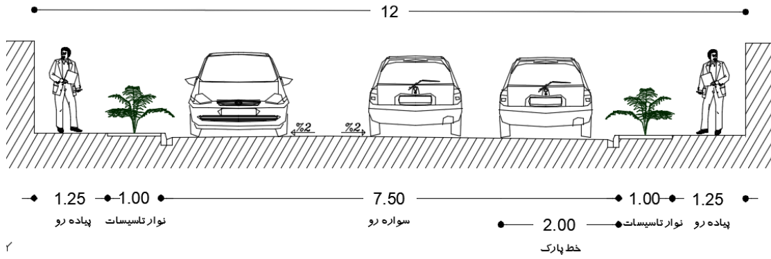
شکل ۲-۱۴- نمونه مقطع عرضی معبر تیب دو - عرض ۱۲- جدول نوع A و B
