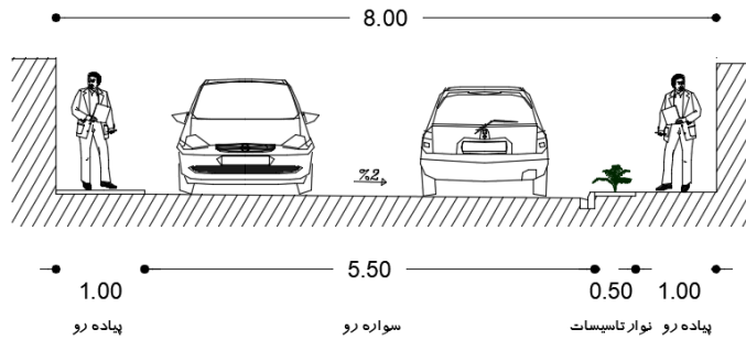
شکل ۲-۱۵- نمونه مقطع عرضی معبر تیب سه - عرض ۸- جدول نوع A و B
