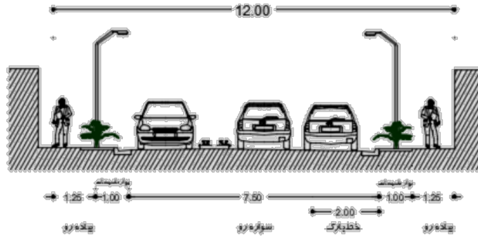
شکل ۲-۱۳- نمونه مقطع عرضی معبر تیب دو - عرض ۱۲- کانپو نوع D
