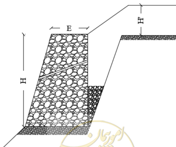
شکل ۵-۲۸-مقطع سیل بند با دیوار حایل سنگی
