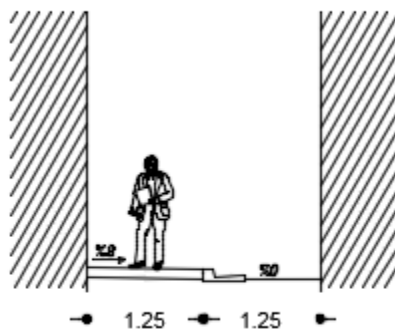
شکل پ ۲-۱۸-مقطع عرضی معبر تیپ پنج - تا عرض ۳- کانپو نوع D
