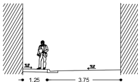
شکل پ ۲-۱۳-مقطع عرضی معبر تیب چهار - عرض ۳ تا ۶-کانیو نوع C
