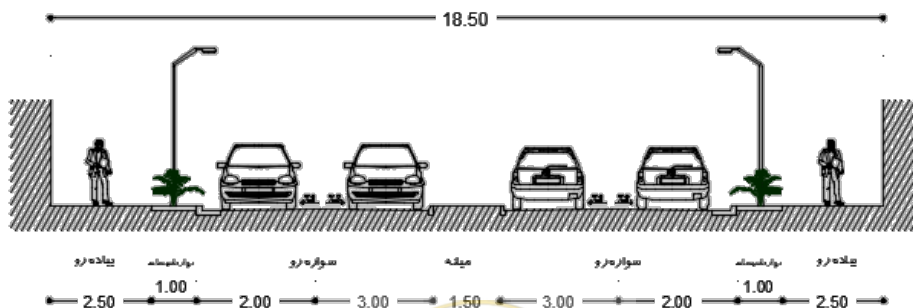
شکل پ ۲-۳-مقطع عرضی معبر تیب یک - عرض ۱۸,۵، ۲۰,۵، ۲۴,۵، ۲۷,۵ و ۱۸,۵-کانیو نوع D
