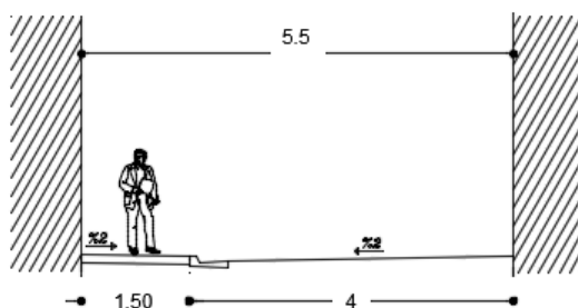
شکل پ ۲-۱۴-مقطع عرضی معبر تیب چهار - عرض ۵ و ۶-کانیو نوع D
