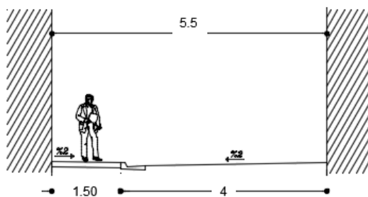
شکل پ ۲-۱۳-مقطع عرضی معبر تیب چهار - عرض ۳ تا ۶-کانیو نوع C
