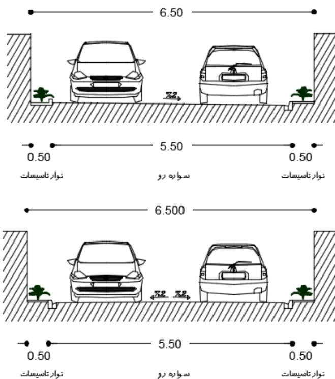
شکل ۲-۱۶- نمونه مقطع عرضی معبر تیپ سه-عرض ۶/۵-جدول نوع A و B
