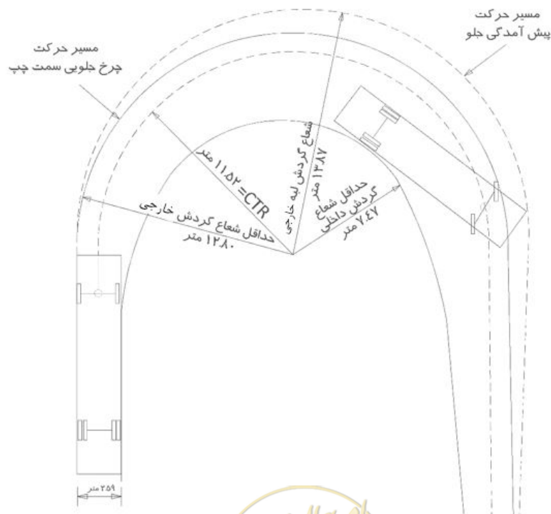
شکل ۲-۳ مشخصات مسیر گردش خودروی طرح، اتوبوس نوع اول با فرض زاویه فرمان ۴۱ درجه (CTR): شعاع گردش مرکز محور
