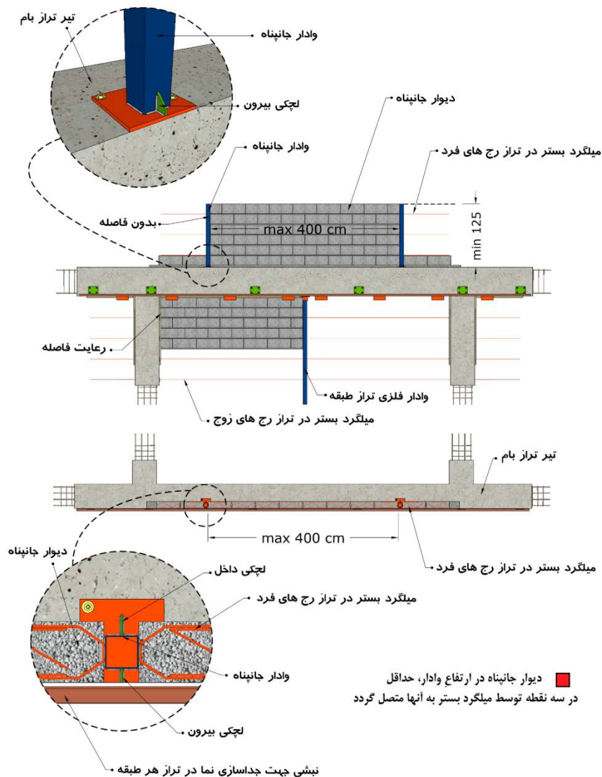
شکل ۱۲-۳۳- مهار جان پناه بنائی توسط وادیار فلزی
