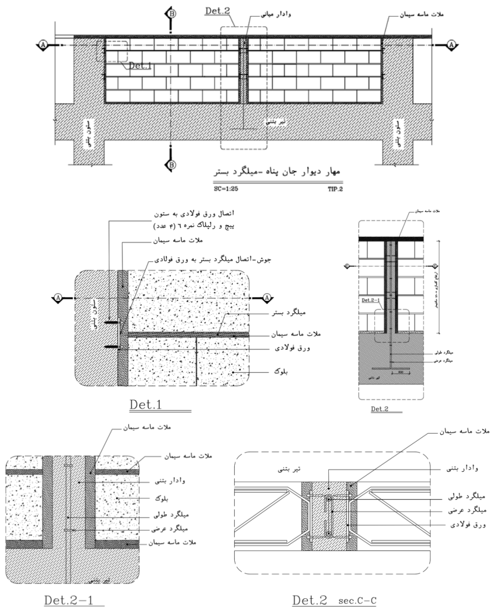
شکل ۱۲-۳۴- جزئیات اجرایی اتصال جان پناه با وادار بتنی
