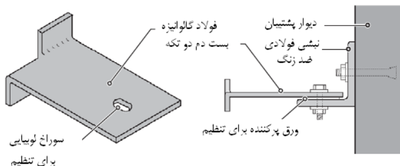
شکل ۴-۸- مهارهای دم دو تکه تنظیم شونده که به وسیله نیشی تکیه‌گاهی که به دیوار پشتیبان متصل شده‌اند
