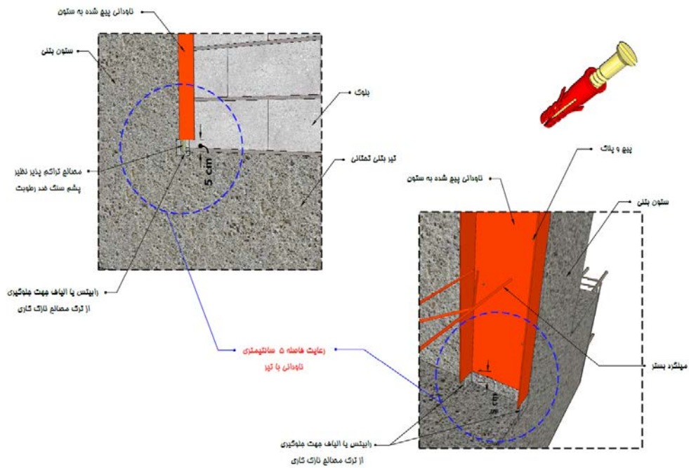
شکل ۱۲-۱۷- اجرای نودانی سرتاسری در مجاورت تیر و ستون در دیوارهای بیمارستانی
