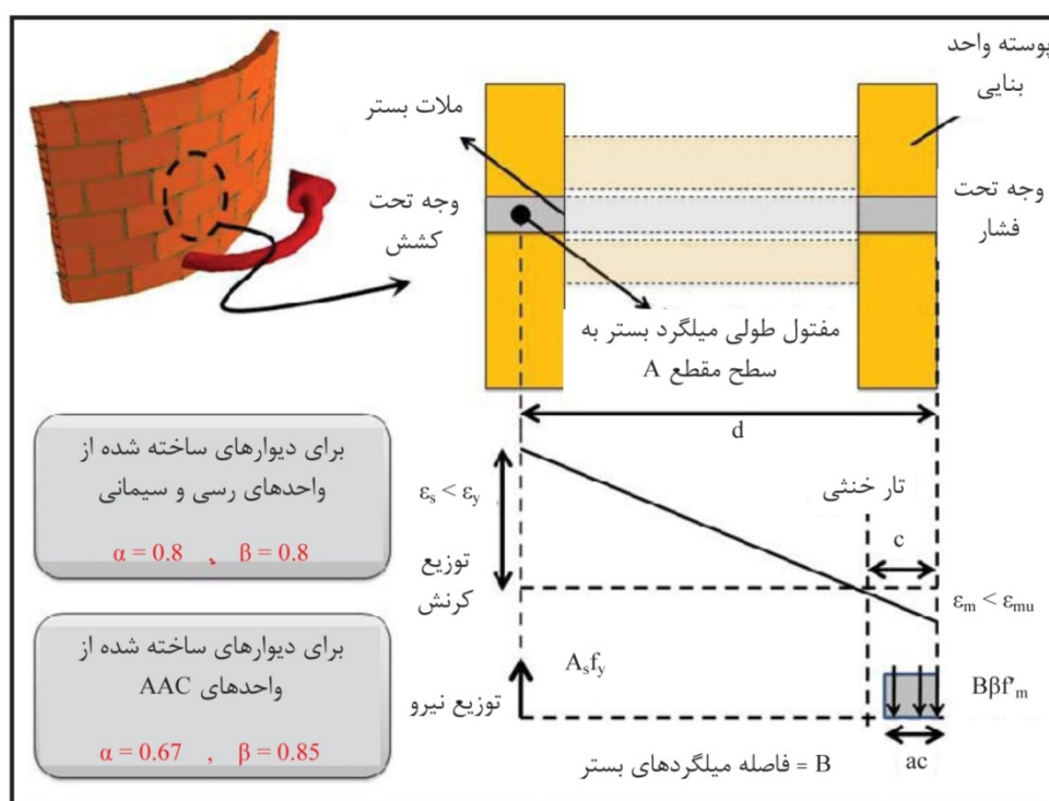
شکل ۱۲-۲- توزیع کرنش و نیرو در مقطع دیوار بنایی با میلگرد بستر ساخته شده از واحد بنایی توخالی
