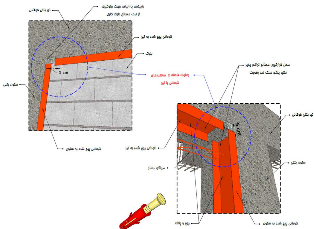
ب- عدم اتصال ناودانی قائم و افقی به یکدیگر شکل ۱۲-۱۸- جزئیات اتصال ناودانی سرتاسری به تیر و ستون
