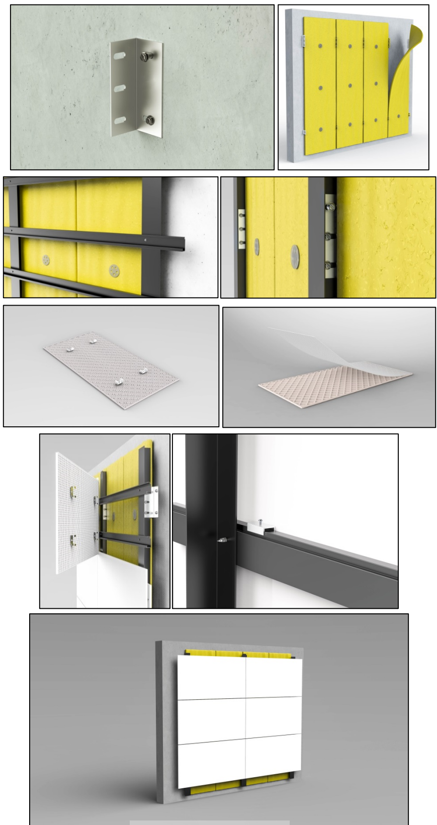
شکل ۷-۱۶- مراحل نصب سیستم نصب پنهان
