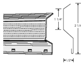
شکل ۱-۳- پروفیل ارتجاعی
