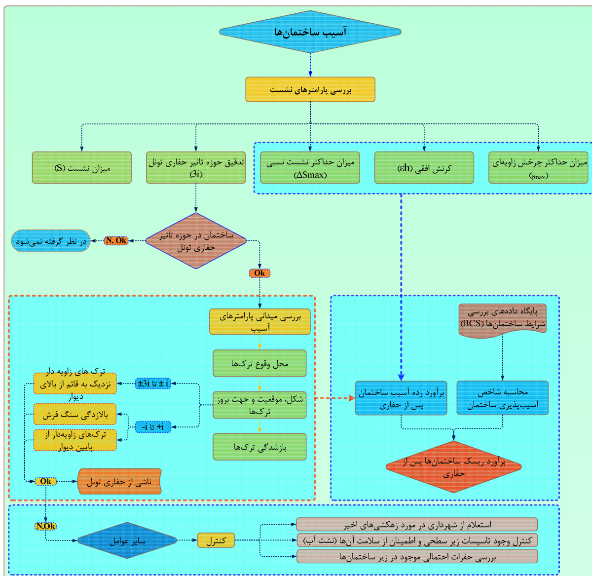
شکل ۶-۳- مراحل شناسایی و نحوه بررسی‌های میدانی آسیب ساختمان‌ها
