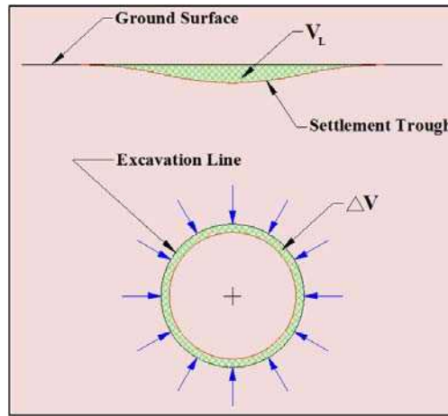
شکل پ.۸-۳- حجم نشست سطحی و حجم از دست رفته زمین
