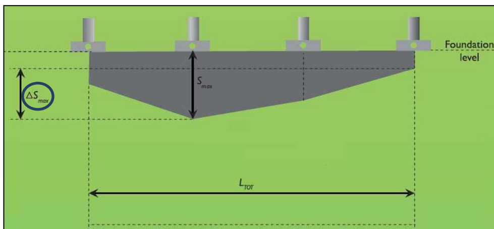
شکل پ.۸-۴- حداکثر تغییر مکان نسبی ( \Delta S_{max} )
