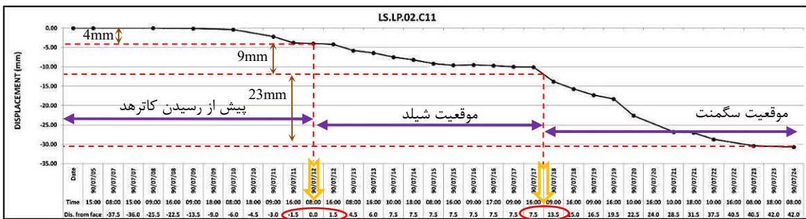
شکل ۵-۸- مقدار جابه‌جایی‌های ثبت شده در مقاطع مختلف حفاری
