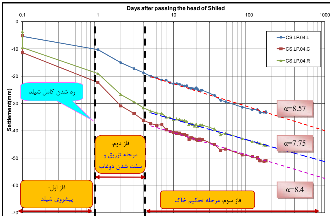
شکل ۵-۹- محاسبه ضریب \alpha و تخمین نشست‌های ۱۰۰۰ روزه برای سه ابزار نشست‌سنجی
