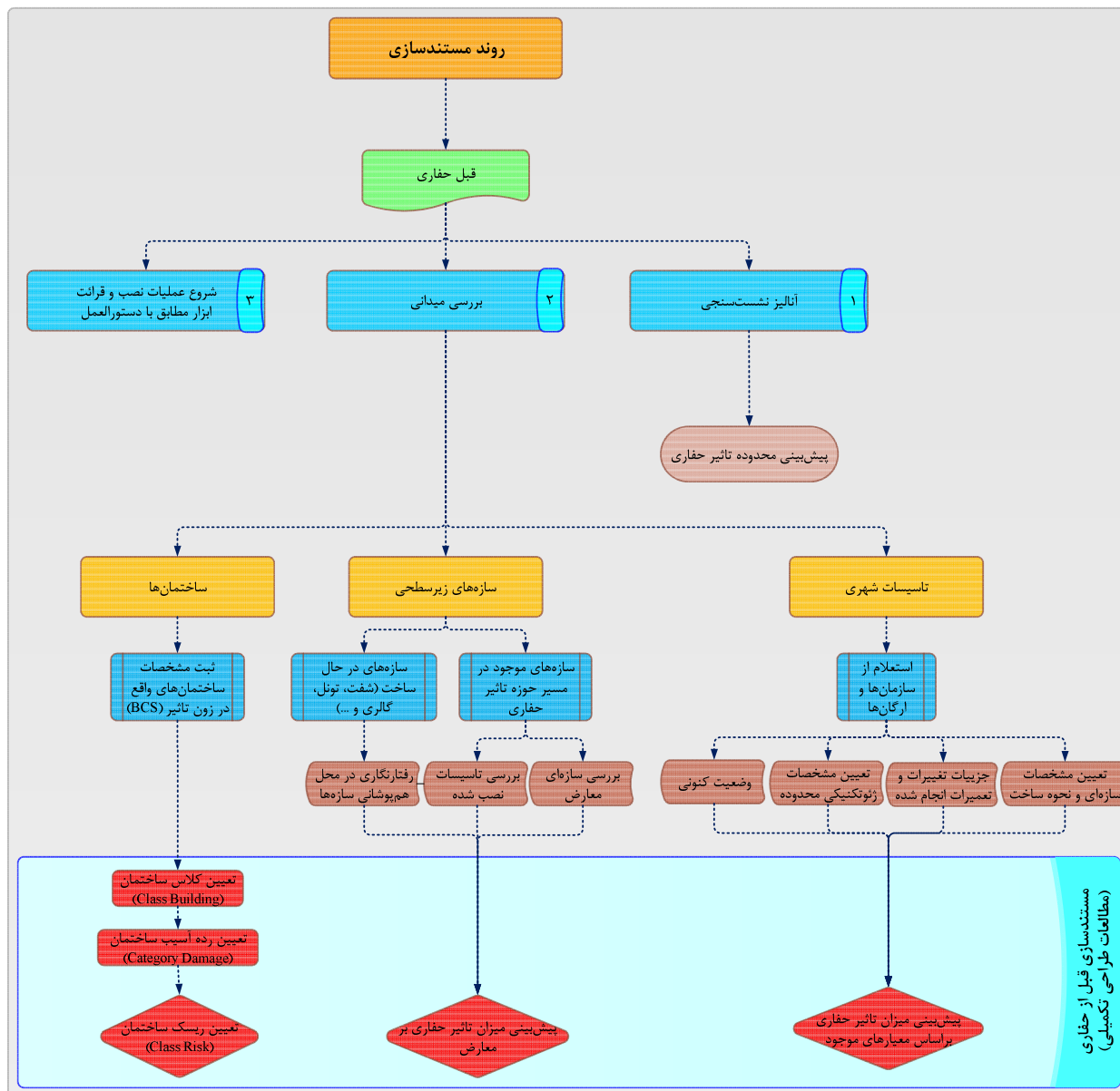
شکل ۶-۶- روند مستندسازی قبل از حفاری تونل
