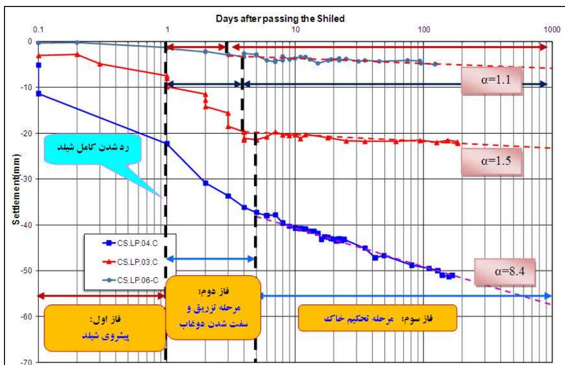
شکل پ. ۸-۷- محاسبه ضریب \alpha و تخمین نشست‌های ۱۰۰۰ روزه برای سه ابزار نشست‌سنجی
