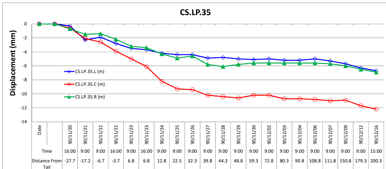
شکل ۵-۴- نمونه‌ای از نمودار نشست‌سنجی حاصل از پردازش اطلاعات تراز یابی
