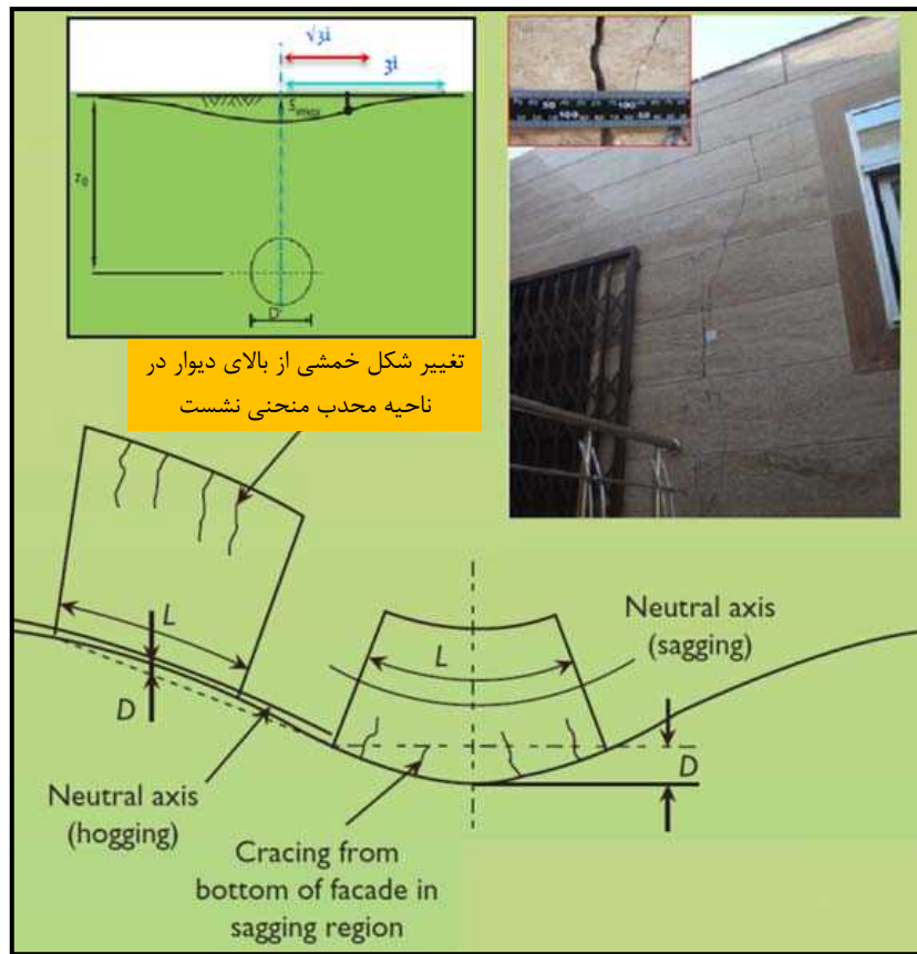
شکل پ. ۱۰-۲- تغییر شکل خمشی و ایجاد ترک کششی در فاصله \sqrt{3}i از محور تونل
