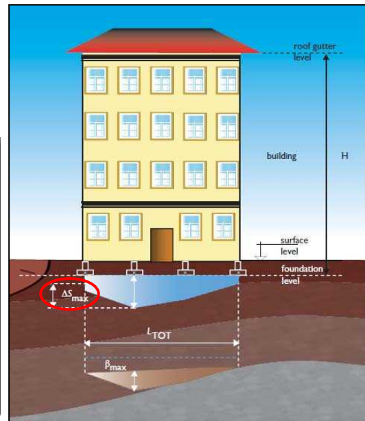
شکل پ.۸-۲- پارامترهای کنترلی \Delta S_{max} و \beta_{max} (راست) - ضریب \alpha (چپ)
