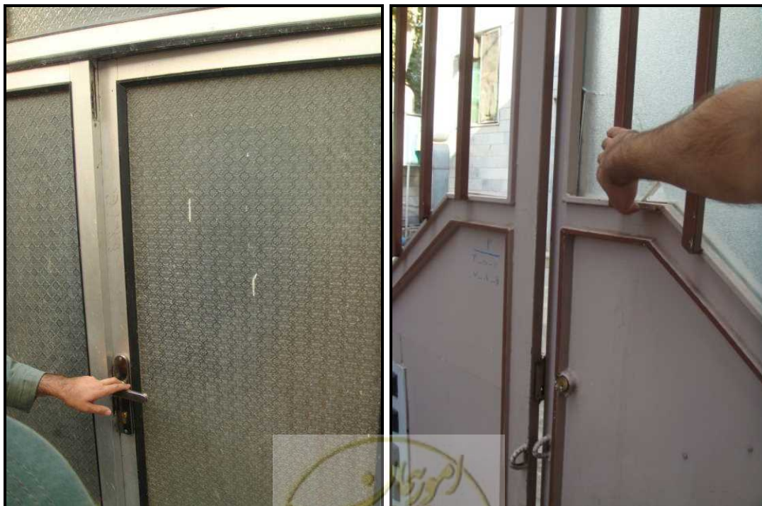
شکل پ. ۱۰-۳- گیرکردن در و پنجره‌ها در اثر نشست
