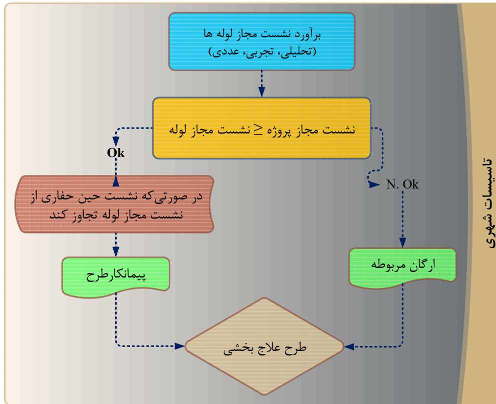
شکل ۴-۶- مراحل کنترل و بررسی میزان نشست‌ها جهت نیل به طرح علاج‌بخش
