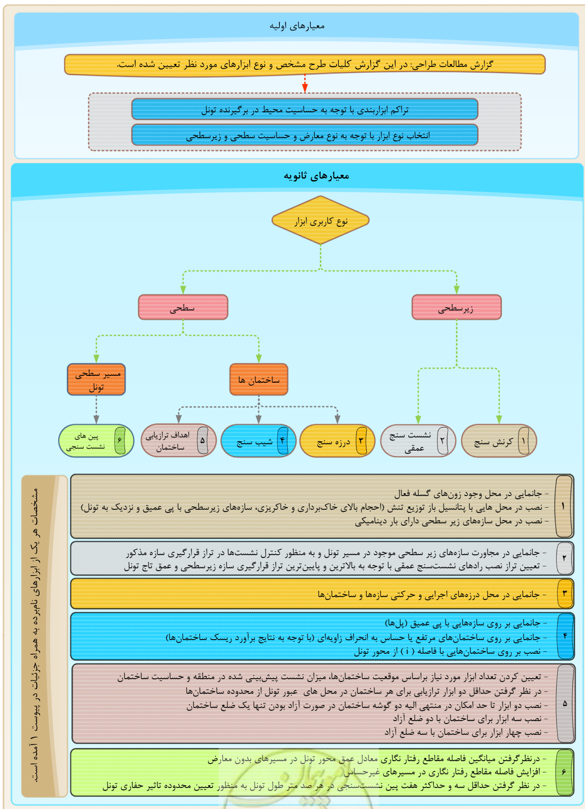
شکل ۲-۶- معیارهای کنترل کننده طراحی پلان جانمایی ابزار دقیق
