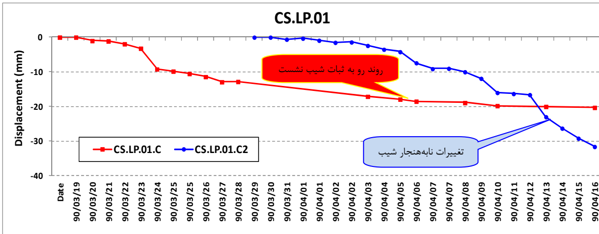
شکل ۵-۵ - روند روبه ثبات و همچنین تغییرات نابه‌هنجار در حین ثبت داده‌های رفتارنگاری
