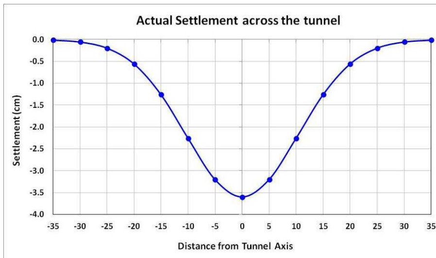
شکل پ. ۸-۶- نمودار نشست واقعی منطقه با توجه به نتایج ابزاربندی مقطع CS-LP-02 پروژه خط ۷ مترو تهران
