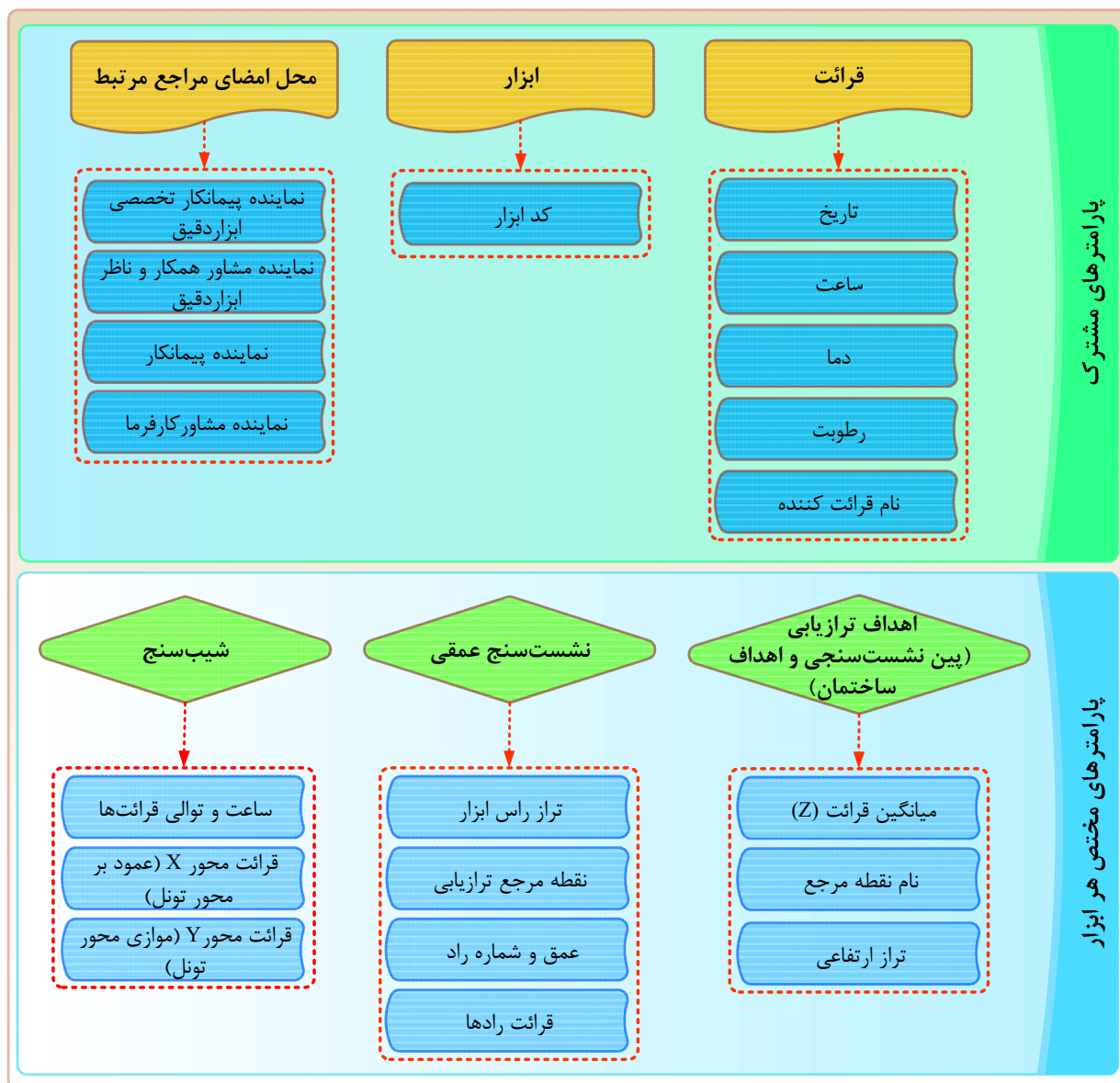
شکل ۲-۸- پارامترهای مهم در طراحی فرم قرائت ابزار
