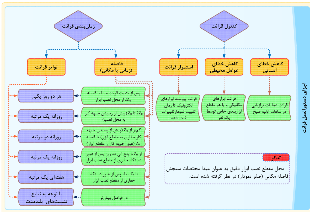
شکل ۴-۱- دستورالعمل قرائت ابزار دقیق
