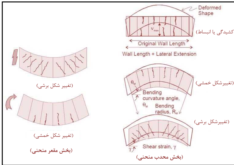
شکل پ. ۱۰-۴- انواع تغییر شکل‌های ممکن برای ساختمان در اثر نشست
