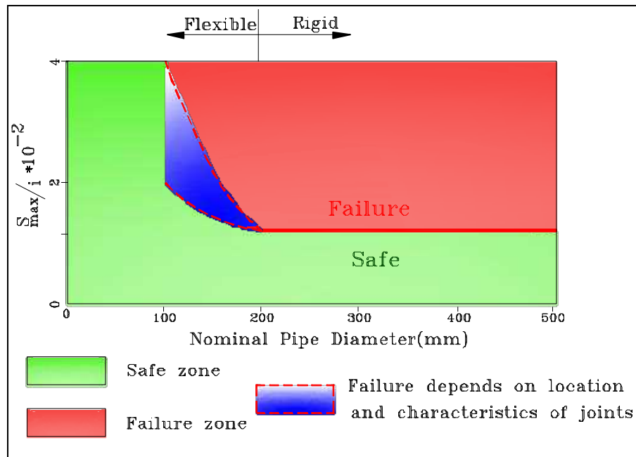
شکل پ. ۱۱-۲- نمودار تجربی ارائه شده توسط ارورکی و تروتمن (۱۹۸۲) برای ارزیابی نشست زمین بر لوله‌ها
