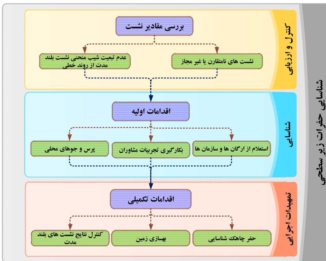
شکل ۶-۲- مراحل شناسایی حفرات
