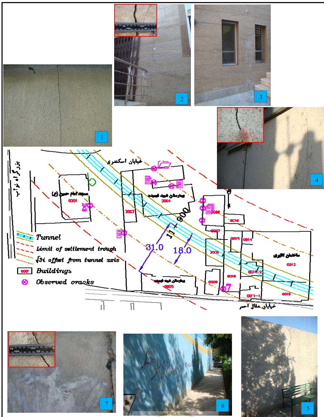
شکل پ. ۱۰-۶- بروز ترک‌های زاویه‌دار یا نزدیک به قائم از بالای دیوار (فاصله \sqrt{3}i از محور تونل)
