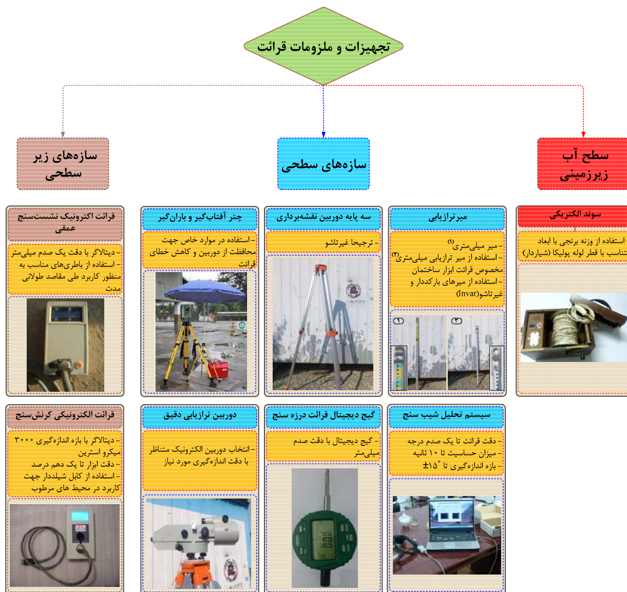
شکل ۴-۳- تجهیزات و ملزومات مورد نیاز برای قرائت ابزار دقیق
