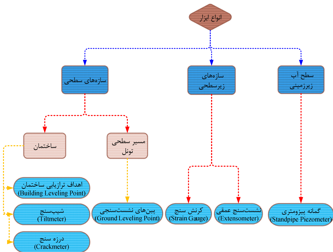
شکل ۲-۳- انواع ابزار پیشنهادی به منظور استفاده در پروژه‌های تونل‌سازی شهری مکانیزه
