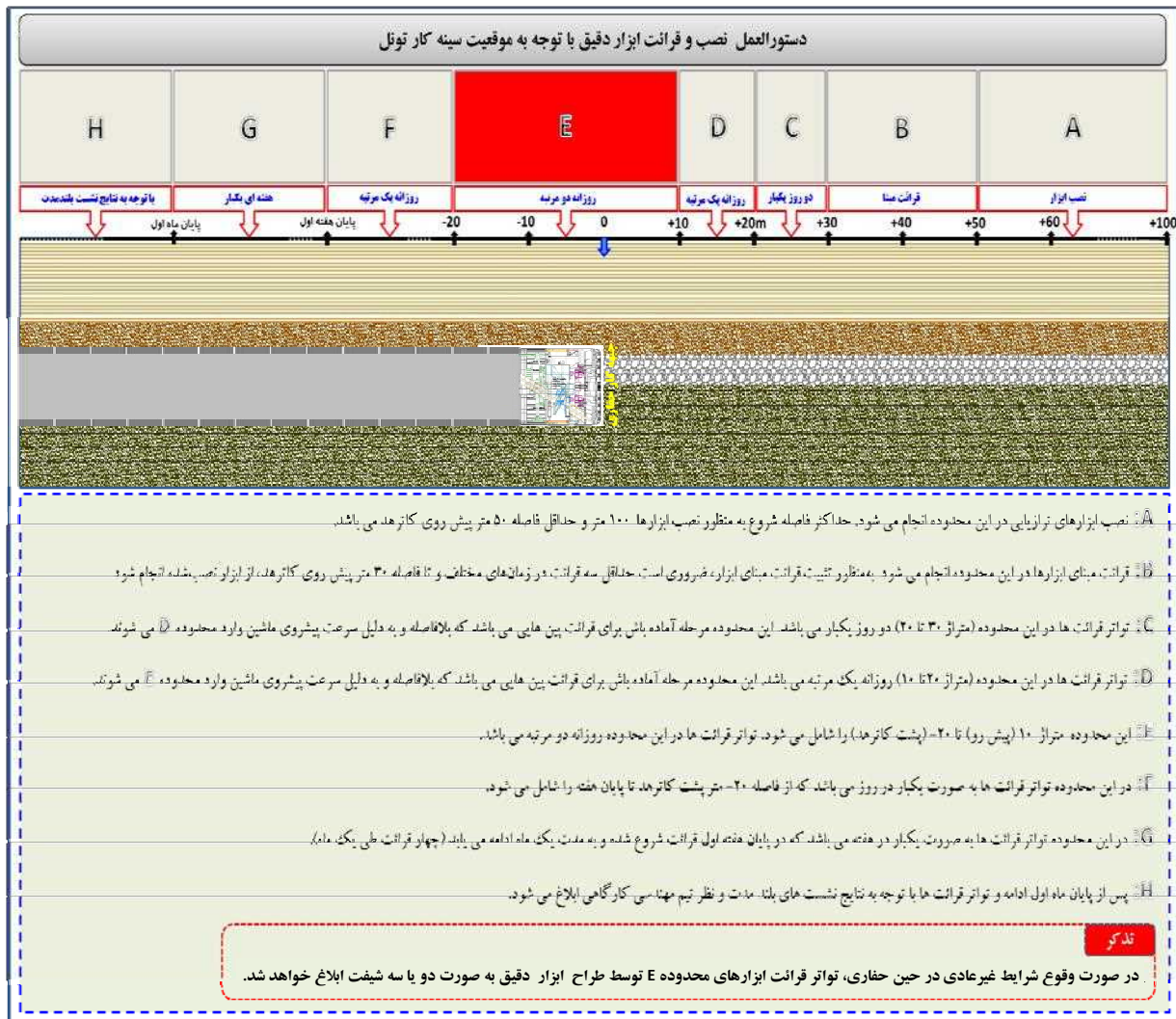
شکل ۴-۲- طرح شماتیک فواصل زمانی و تواتر قرائت ابزار دقیق
