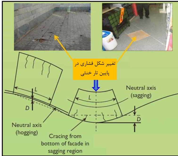
شکل پ.۱۰-۱- تغییر شکل فشاری و بالازدگی سنگ‌فرش بر روی محور تونل
