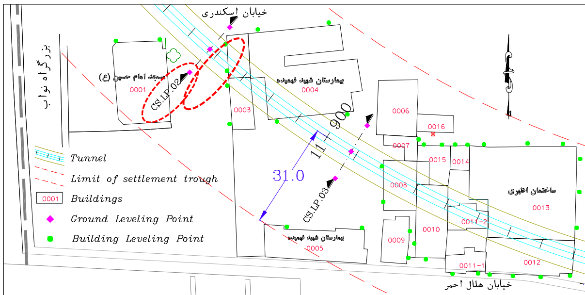
شکل پ. ۸-۵- تعیین حوزه تاثیر حفاری تونل با توجه به نتایج رفتارنگاری
