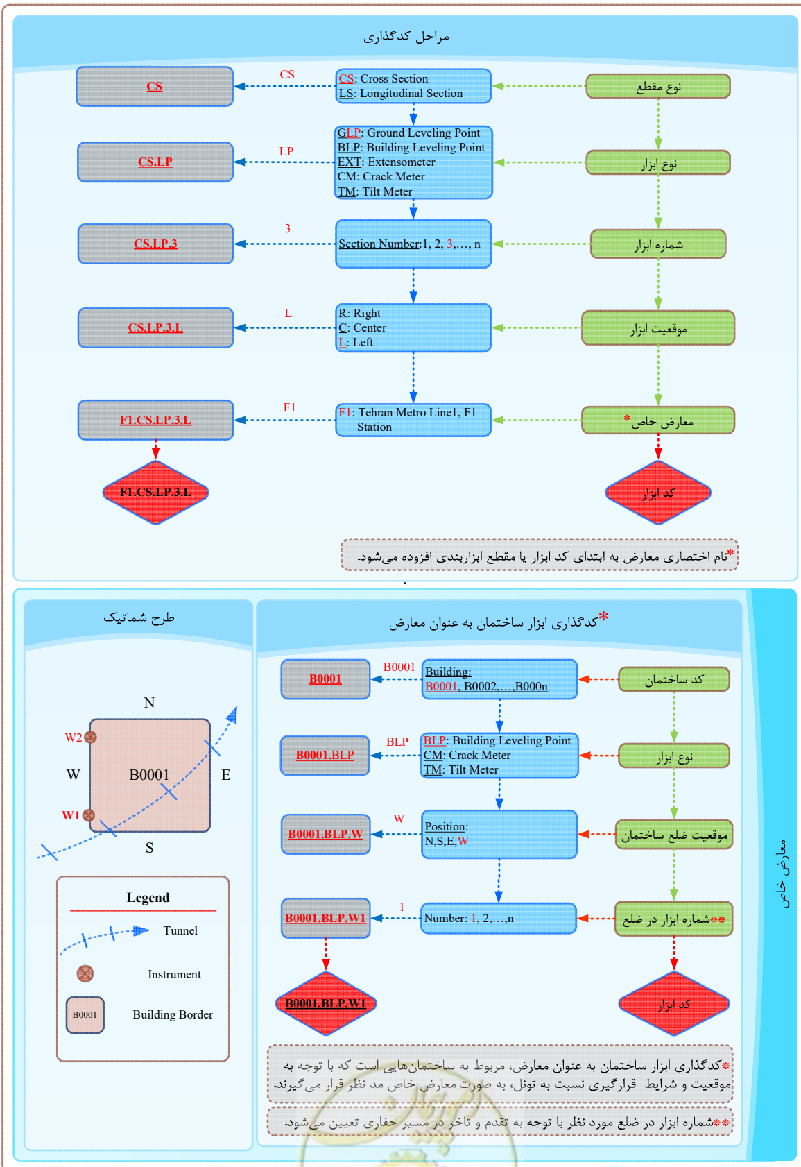
شکل ۲-۵- مراحل کدگذاری هر ابزار یا مقطع ابزاربندی
