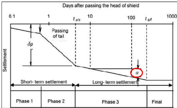
شکل پ.۸-۲- پارامترهای کنترلی \Delta S_{max} و \beta_{max} (راست) - ضریب \alpha (چپ)
