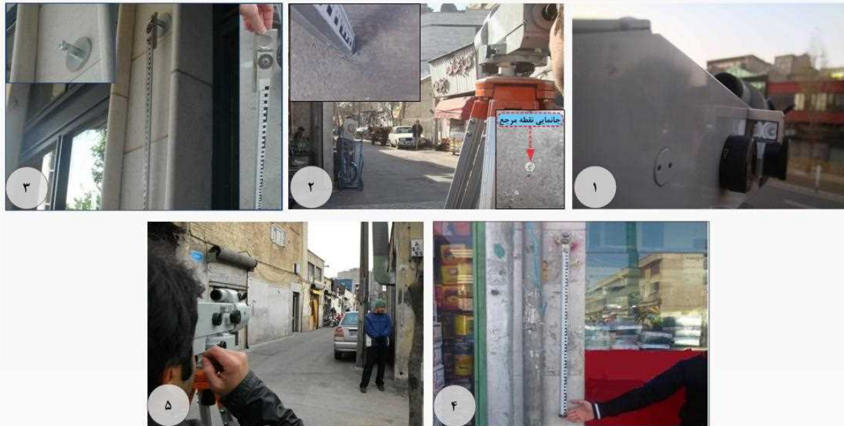
توضیحات: ۱- استقرار و تراز کردن دوربین ۲- قرائت نقطه مرجع ۳- استقرار میر ترازبایی مخصوص ساختمان بر روی شیار جانمایی شده بر روی ابزار ۴- ثابت کردن میر ترازبایی به منظور قرائت ۵- قرائت ابزار ترازبایی
