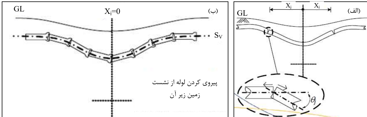
شکل پ.۱۱-۱- نحوه تغییر شکل لوله‌ها: الف- لوله کاملاً منعطف، ب- لوله کاملاً صلب با اتصالات منعطف
