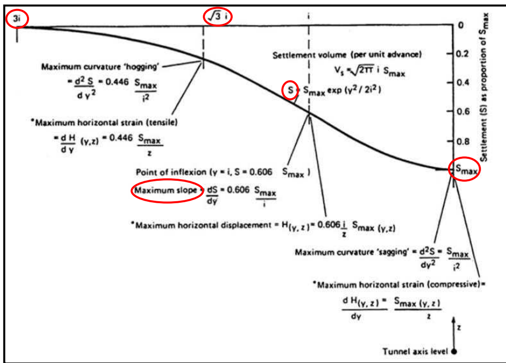
شکل ۸. پ. ۱-۸ پارامترهای کنترلی در بررسی نشست
