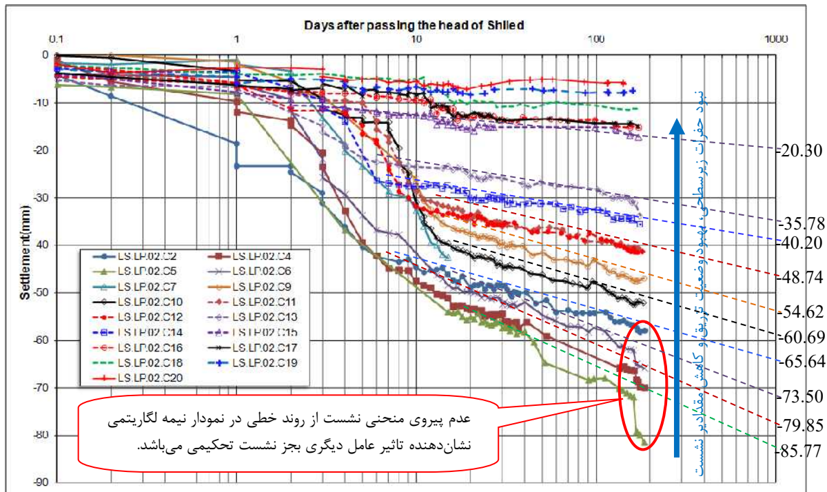
شکل پ.۹-۳- نمونه ای از عدم پیروی منحنی نشست از روند خطی در نمودار نیمه لگاریتمی
