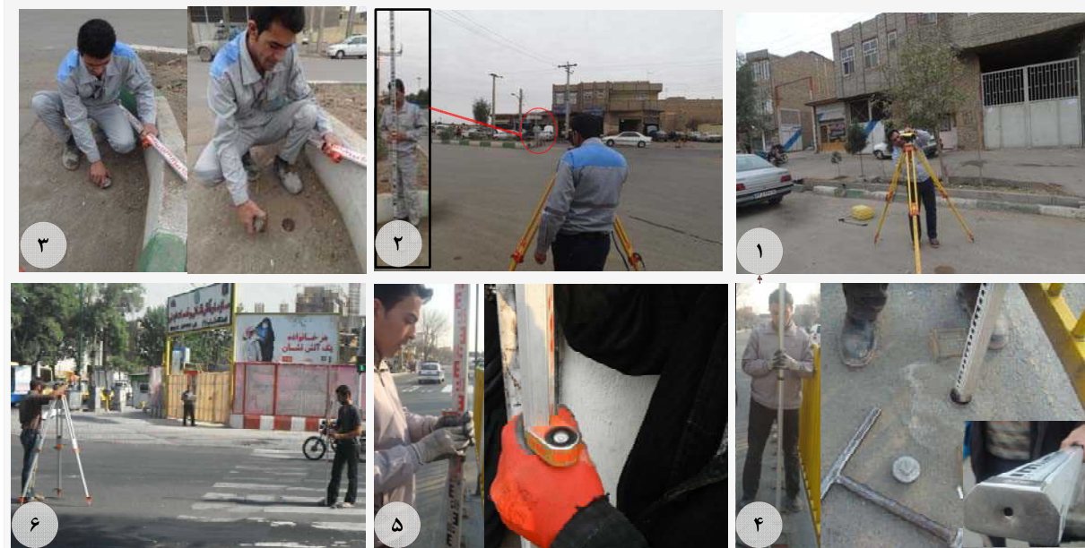
توضیحات: ۱- استقرار و تراز کردن دوربین ۲- قرائت نقطه مرجع ۳- باز کردن درپوش ۴- استقرار فرورفتگی میر ترازبایی بر روی ساچمه ۵- تراز کردن میر ترازبایی ۶- قرائت بین نشست‌سنجی
