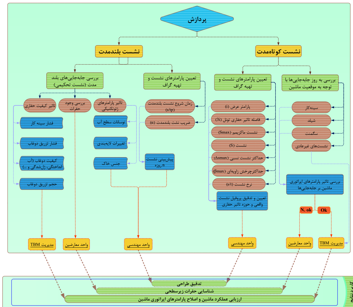
شکل ۵-۷- مراحل فرآیند تحلیل و تفسیر نهایی نتایج
