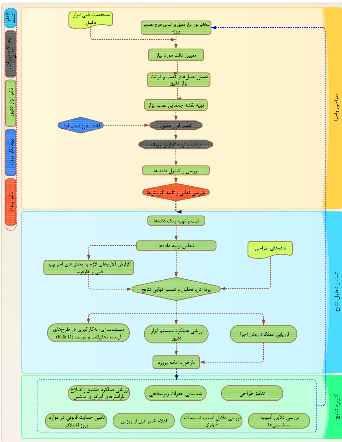
شکل ۲-۱- روند اجرای برنامه ابزاربندی و رفتارنگاری حین اجرای تونل‌های مکانیزه شهری
