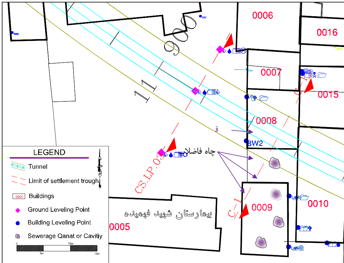
شکل پ.۹-۱- پلان مسیر تونل در محدوده ساختمان شماره ۸ و ۹
