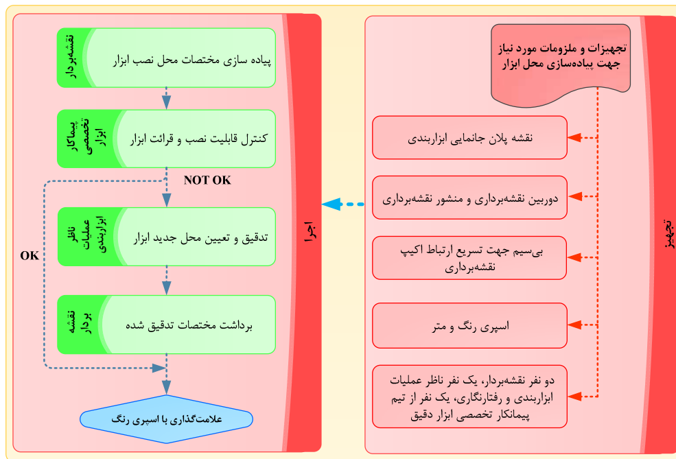
شکل ۱-۳- تجهیز و پیاده‌سازی ابزار
