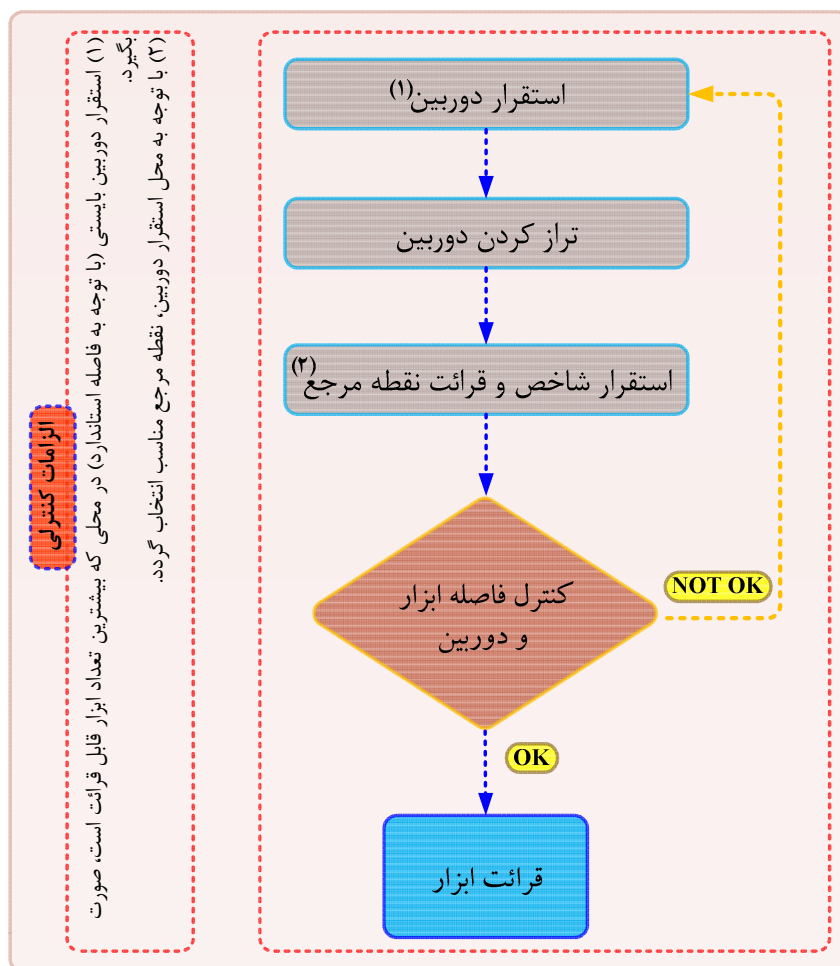
شکل ۴-۴ - نمودار جریان‌ی نحوه قرائت ابزار دقیق
